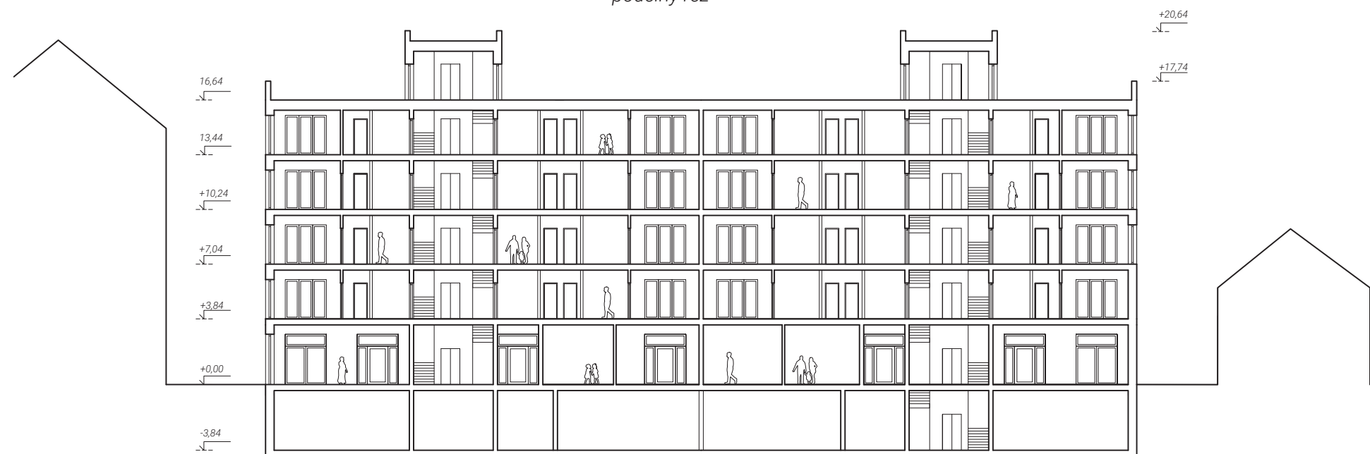
podelný řez
