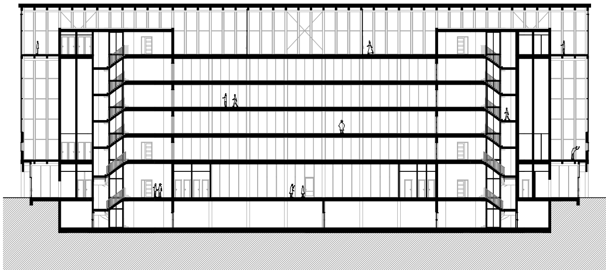
ŘEZ PODÉLNÝ 1:500
