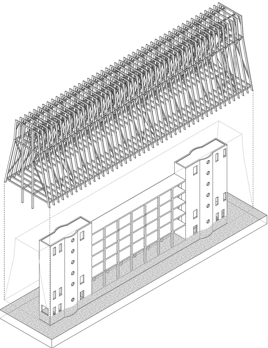
AXONOMETRIE KONSTRUKCE 1:500
