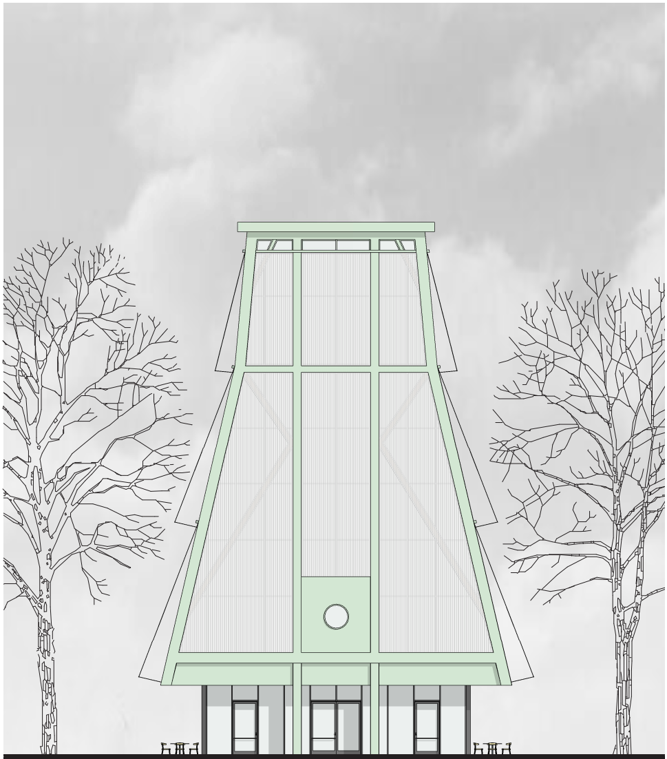
POHLED ZÁPADNÍ 1:250
