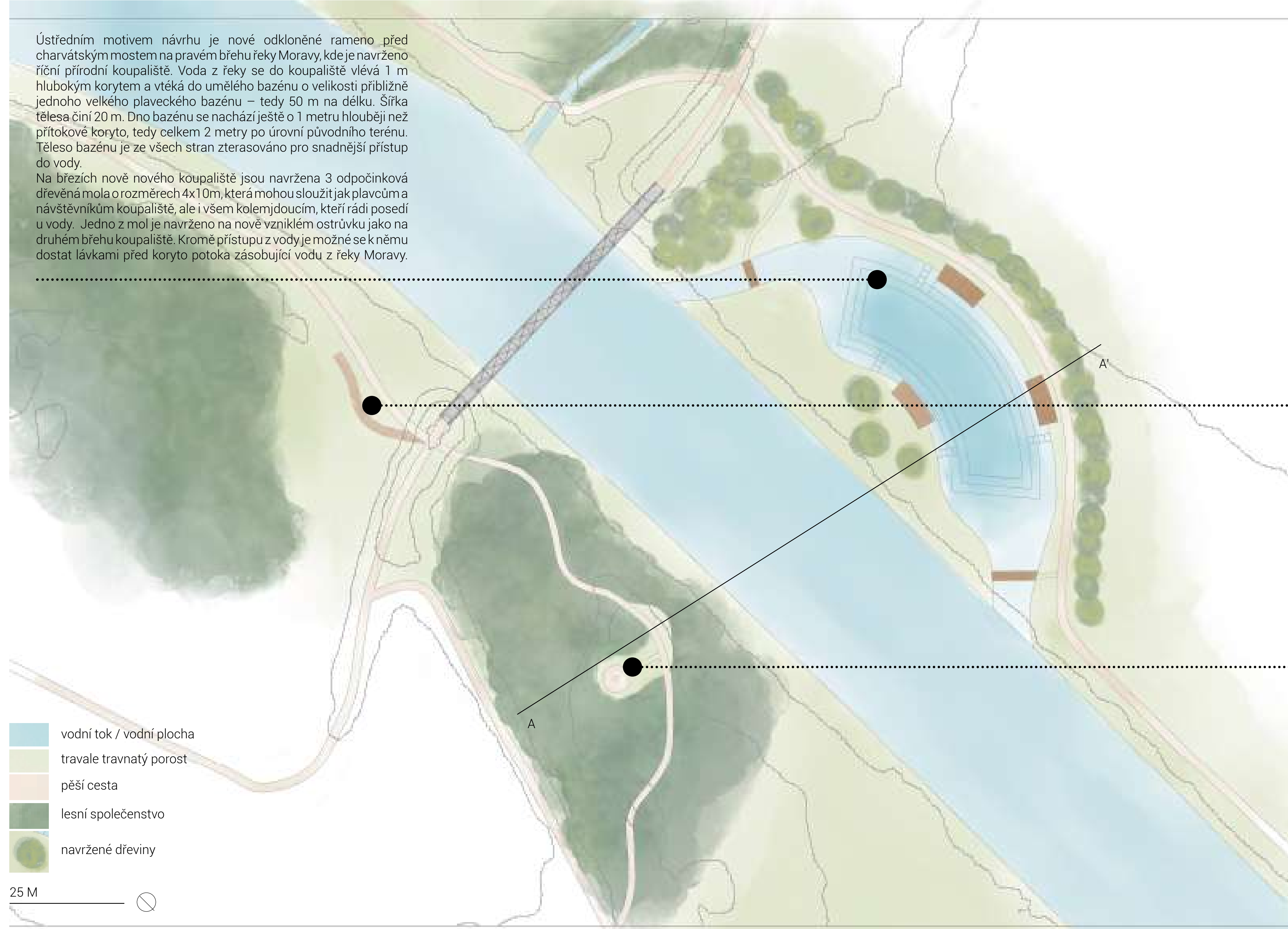
NÁVRHOVÁ SITUACE 1:500
