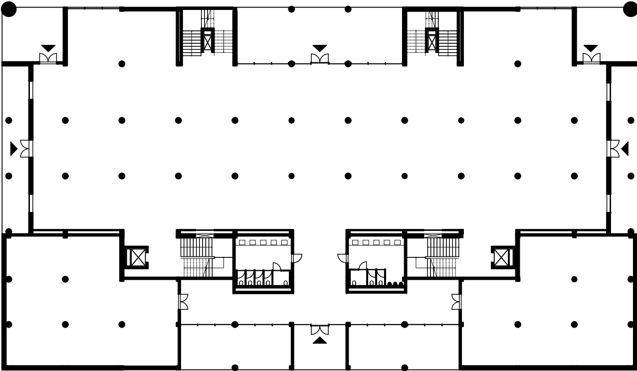
1.NP - Tržnica
