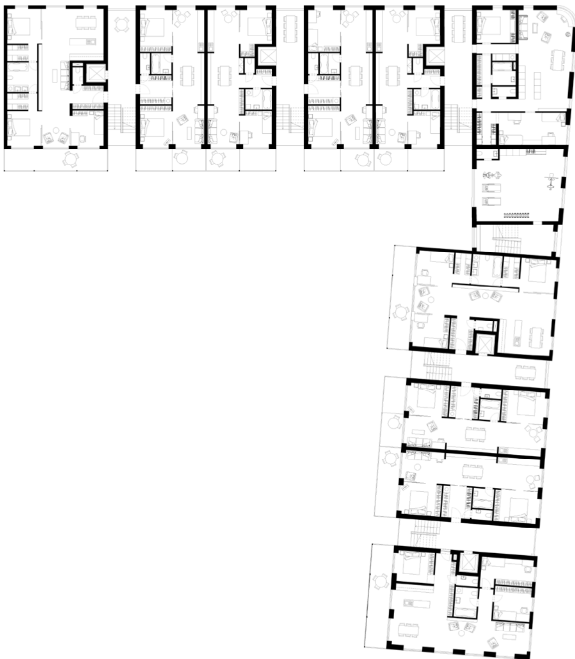
PŮDORYS 2. NP - 4.NP
