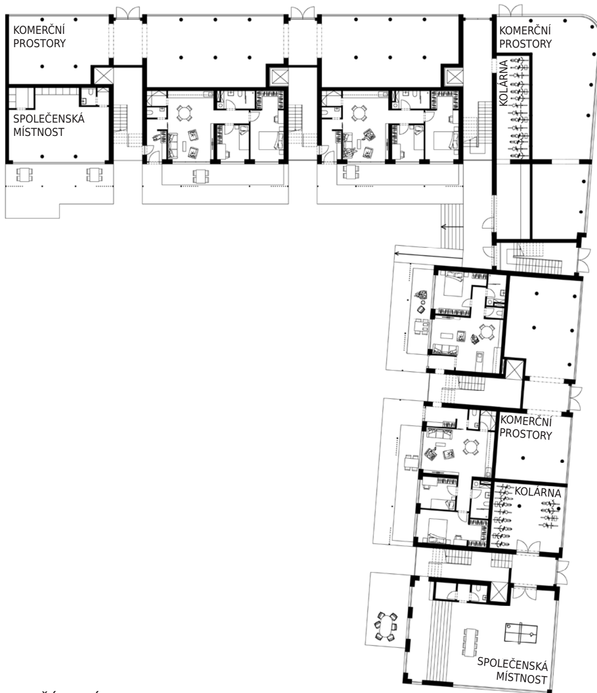
PŮDORYS PŘÍZEMÍ
