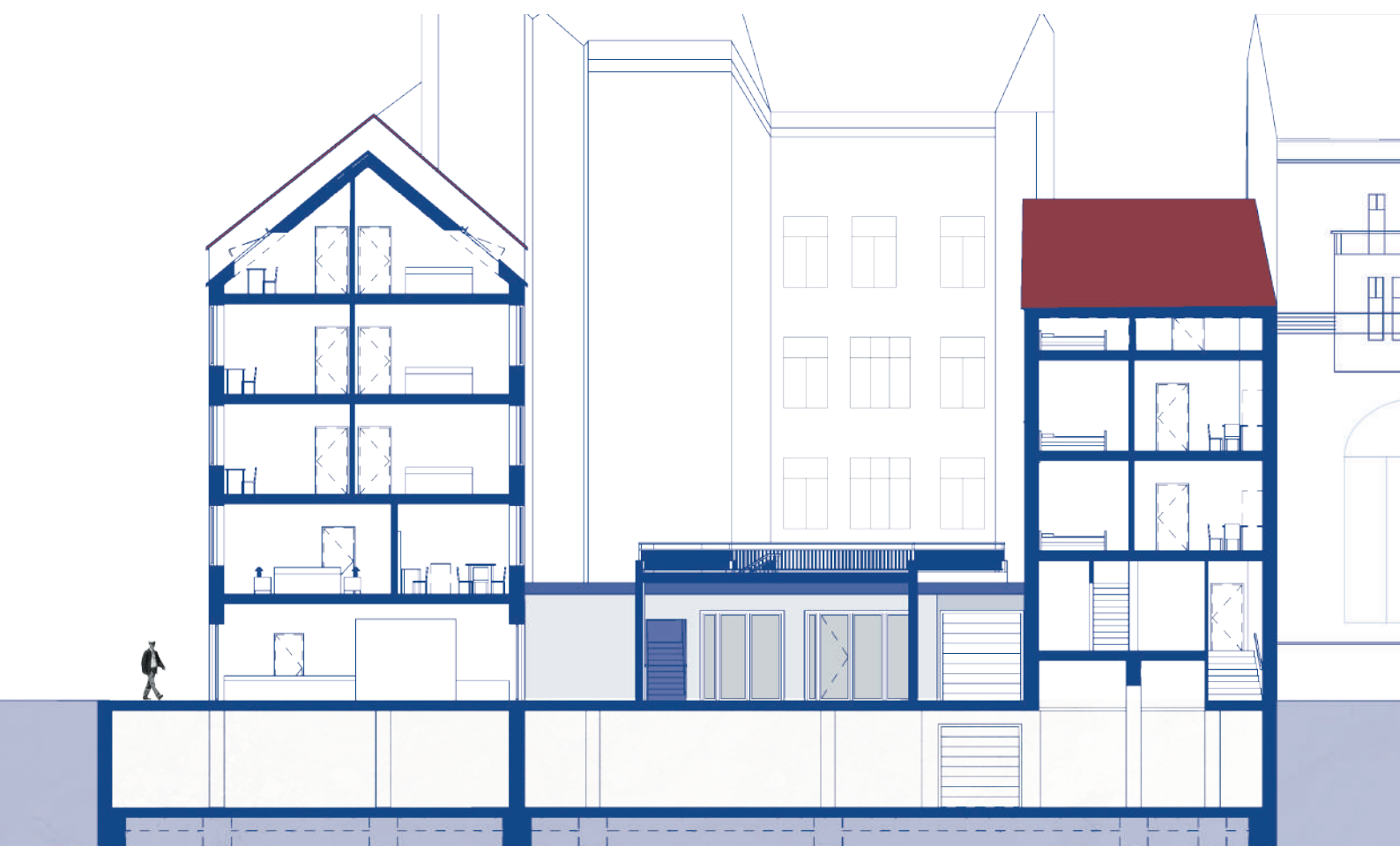
ŘEZ A-A
