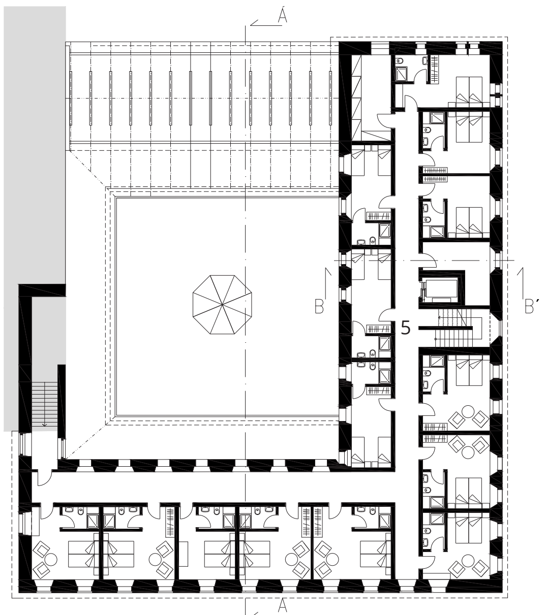
Půdorys 2NP - klášter M 1 : 250
