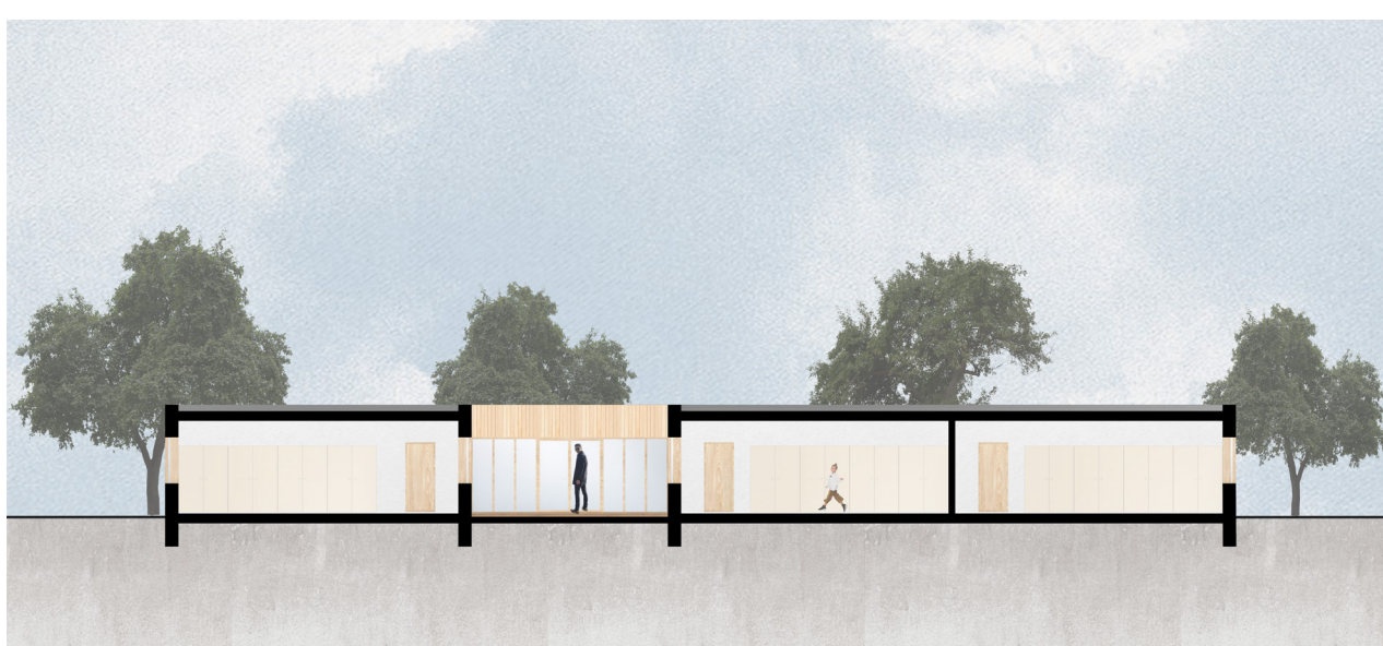
Řez budovou skautské klubovny M 1 : 250
