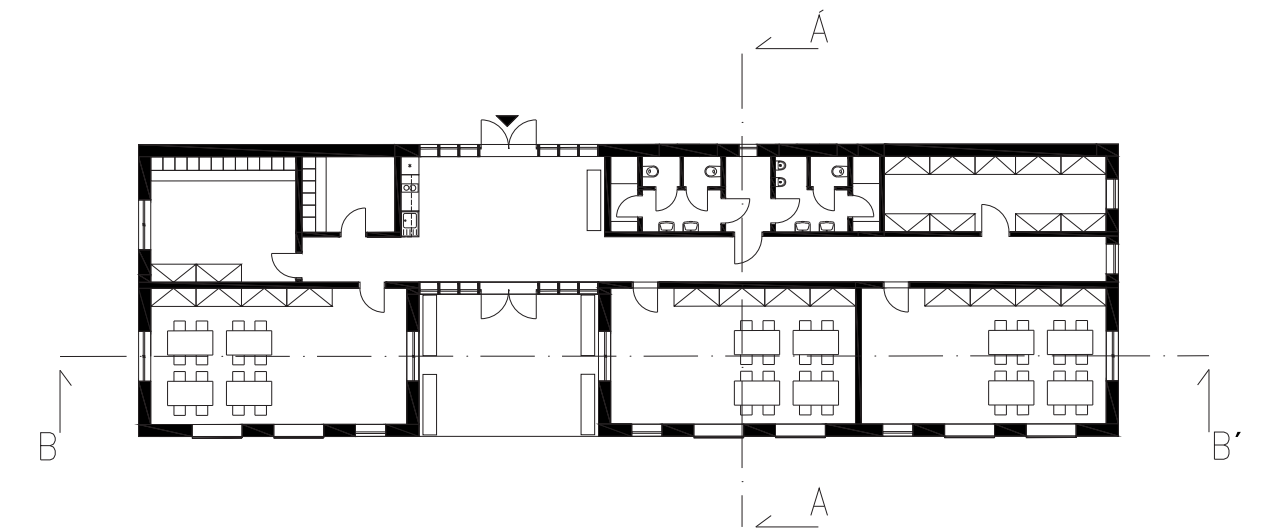
Půdorys 1NP - skautská klubovna M 1 : 250
