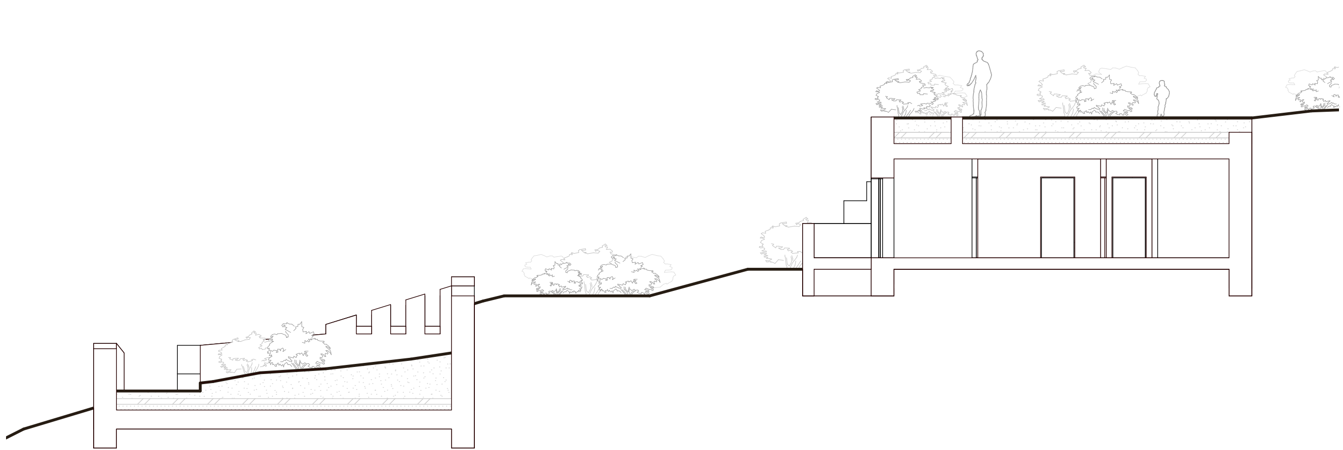
ŘEZ | OBJEKT C/B | M 1:100
