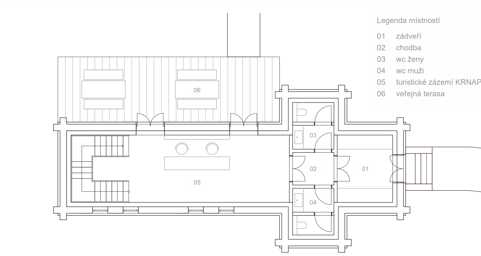
PŮDORYS 1.NP | OBJEKT A | M 1:100
