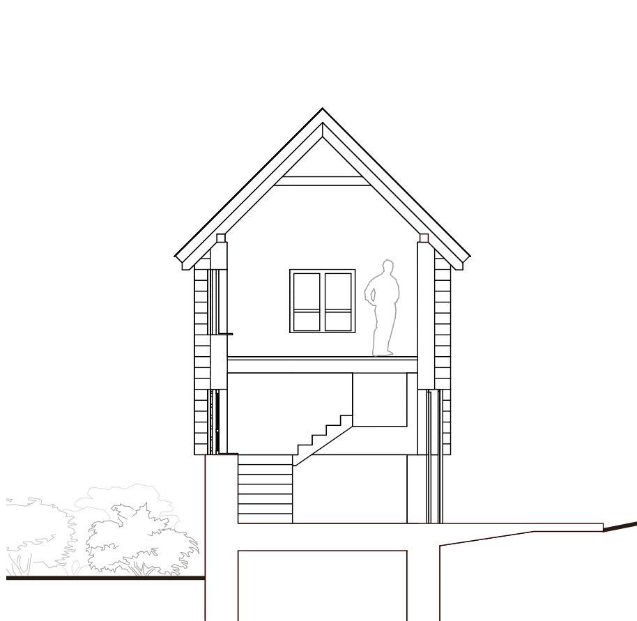
ŘEZ | OBJEKT A | M 1:100
