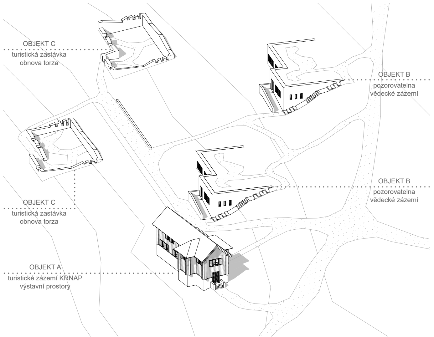
AXONOMETRIE
