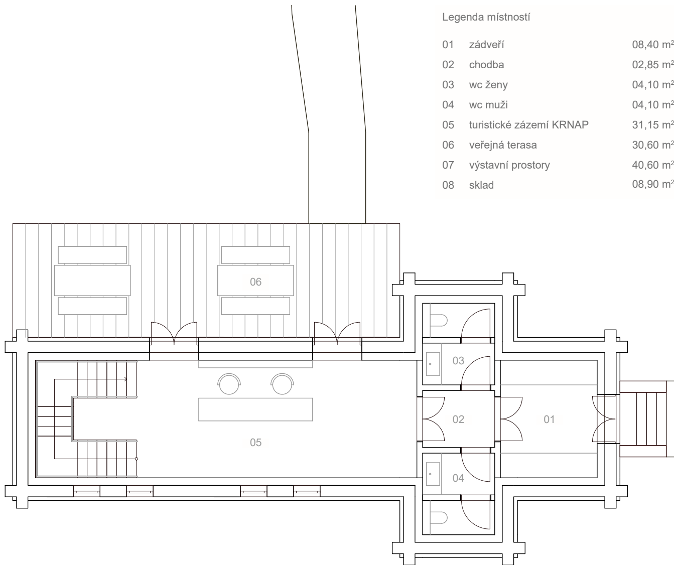
1.NP | M 1:100
