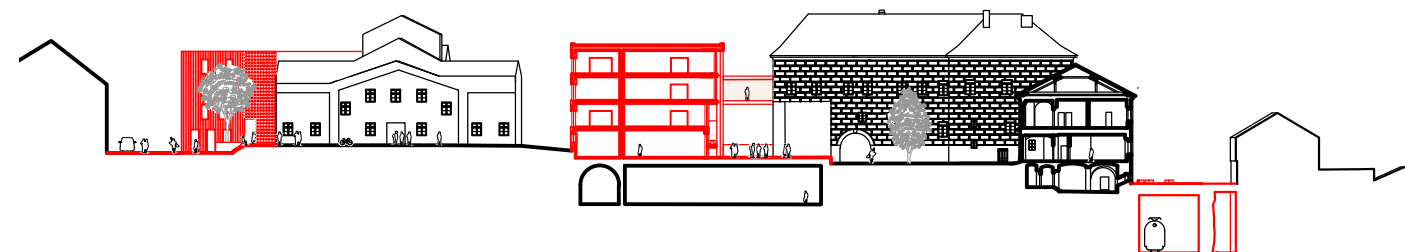
ŘEZOPHLED D-D' ŘEZ NOVOU BUDOVOU KNIHOVNY A POHLED NA BYTOVÝ DŮM U DIVADLA
