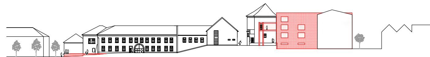
POHLED B-B' MOSTEK SPOJUJÍCÍ NOVOU A STAROU BUDOVU KNIHOVNY
