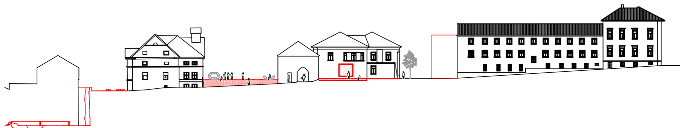
POHLED A-A' NOVÉ OKNO BÝVALÉHO PURKRABSTVÍ A OBNOVRNÁ GOTICKÁ BRÁNA
