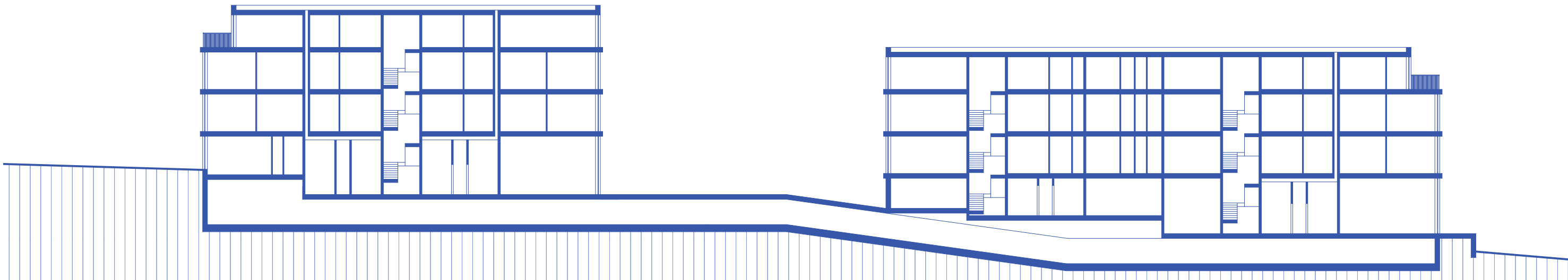
ŘEZ A - A' M 1:333
