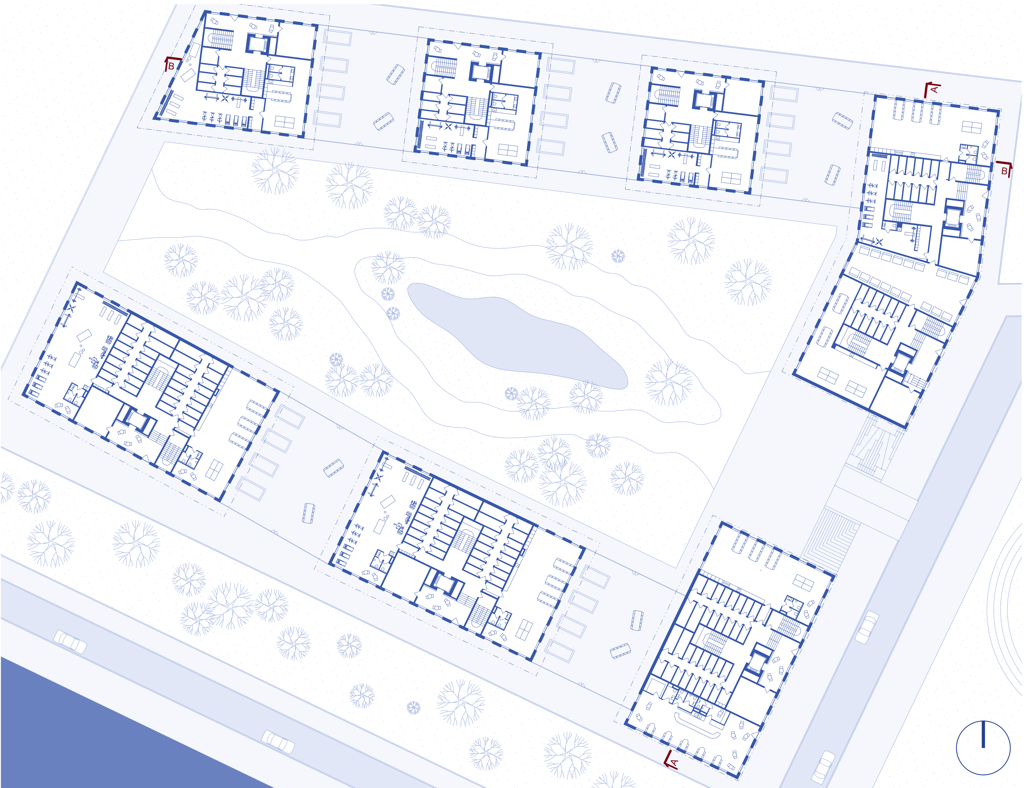
PŮDORYS 1 NP M 1:333
