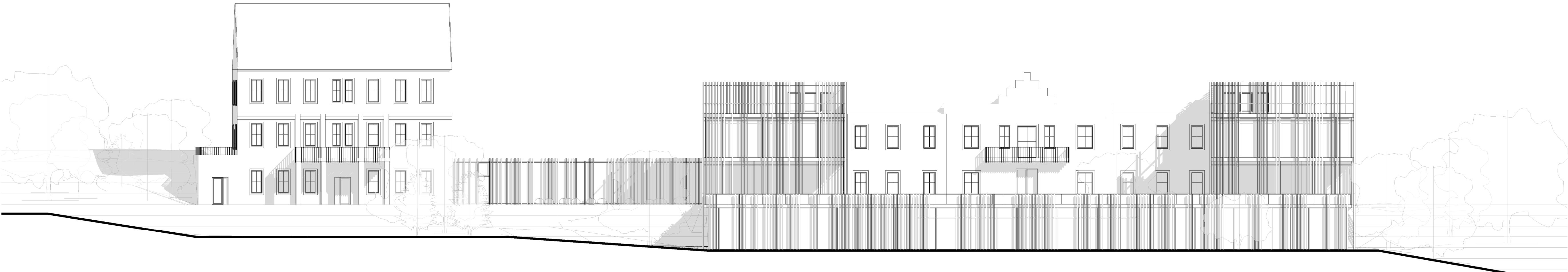
POHLEDY 1:200
