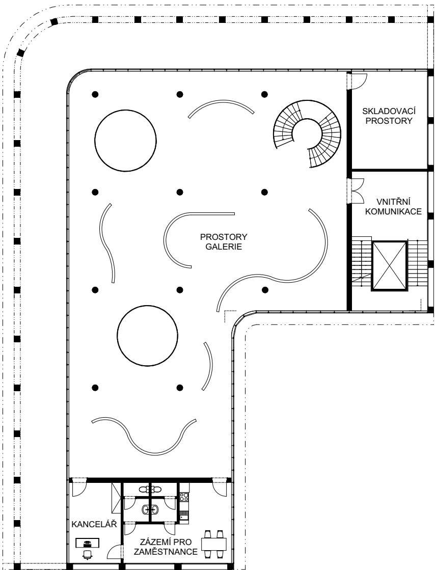
PŮDORYS DRUHÉHO PODLAŽÍ 1:250
