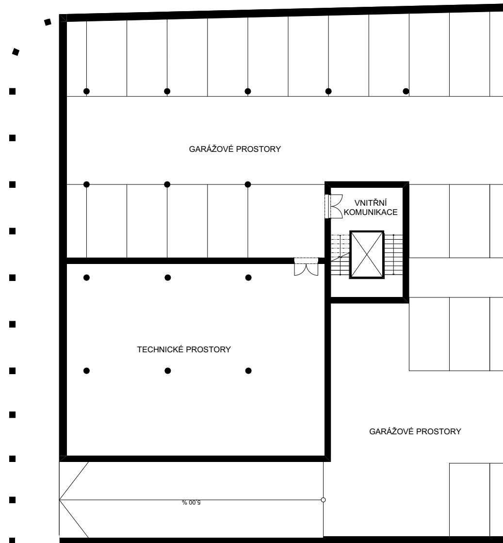
PŮDORYS SUTERÉNU 1:250
