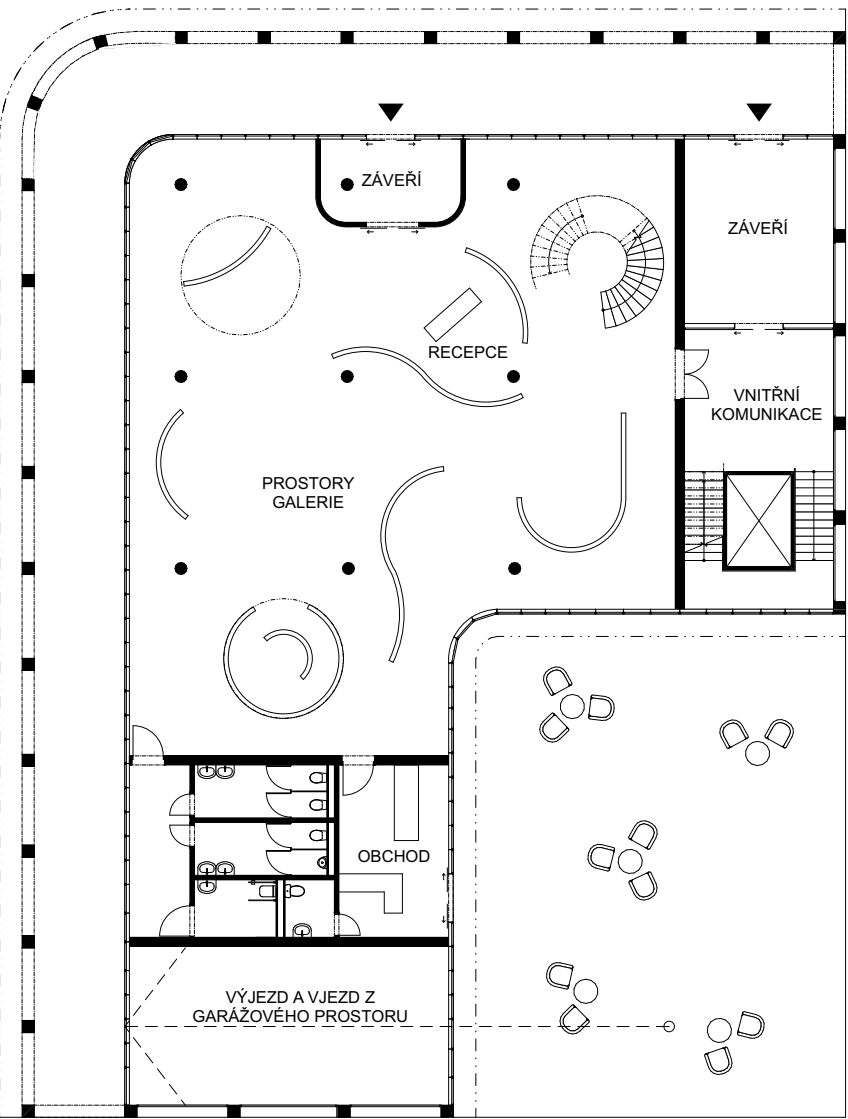
PŮDORYS PŘÍZEMÍ 1:250
