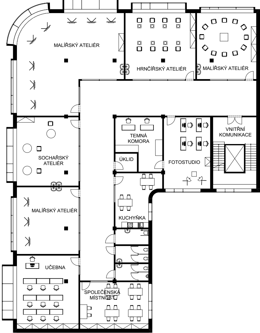
PŮDORYS TYPYCKÉHO PODLAŽÍ 1:250
