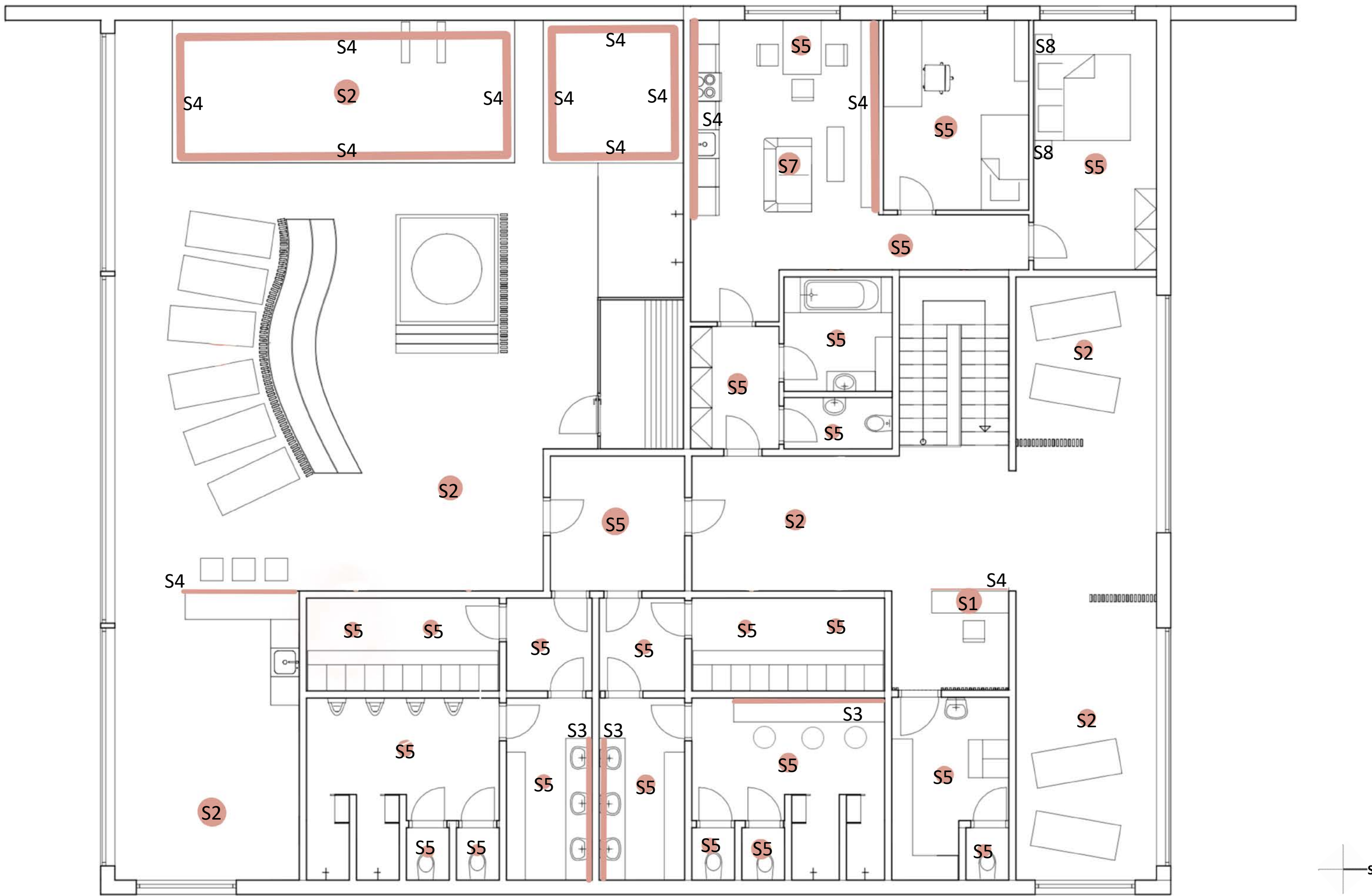
OSVĚTLENÍ schéma 2. podlaží
