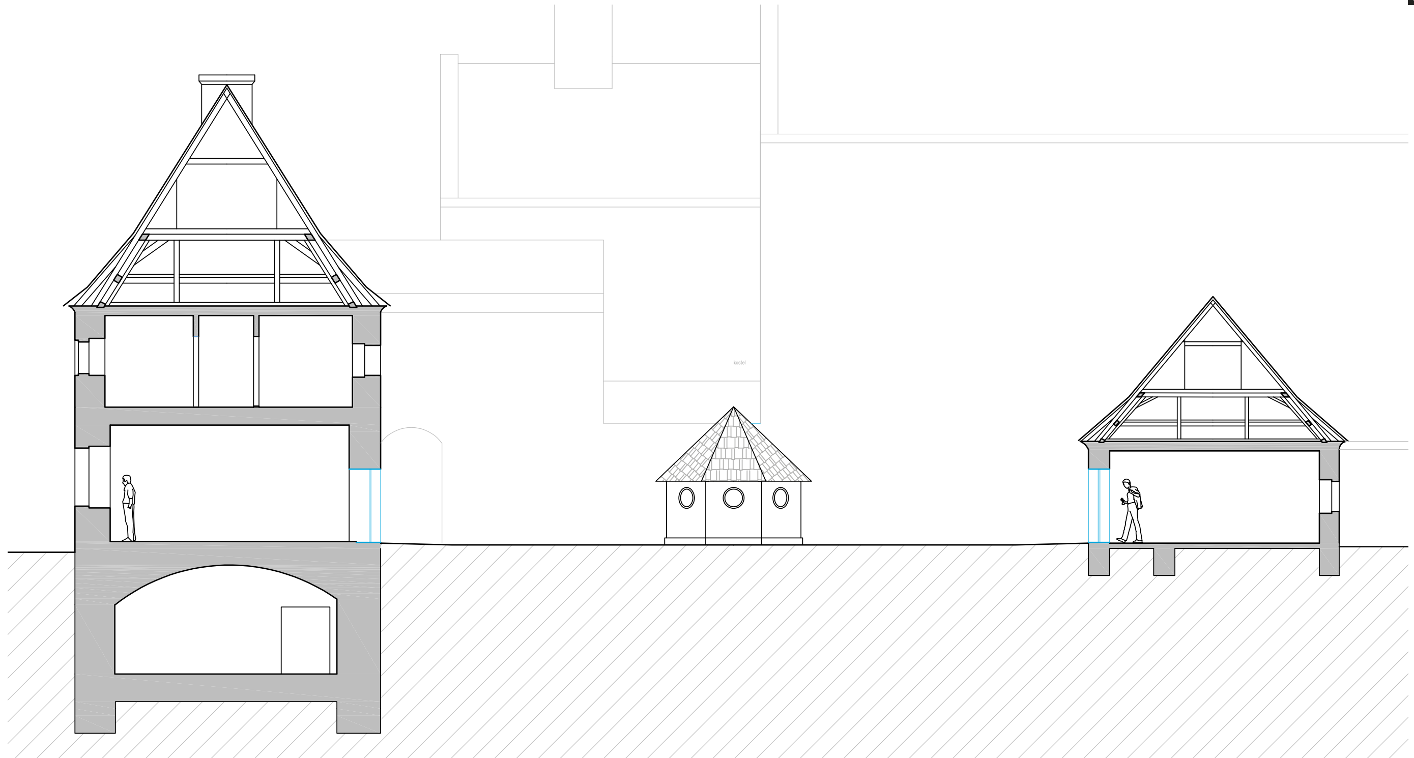
Řez JZ-SV
