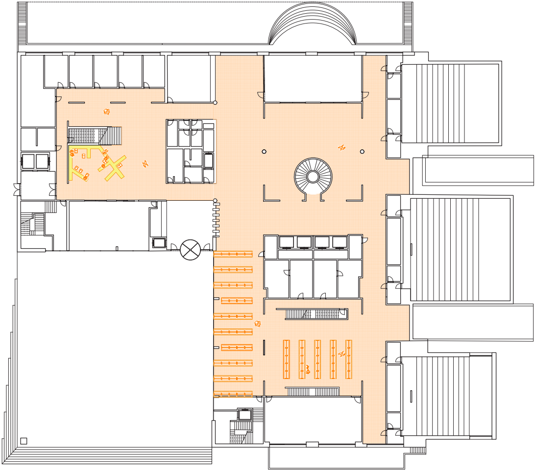
Půdorys - FA ČVUT M 1:500
