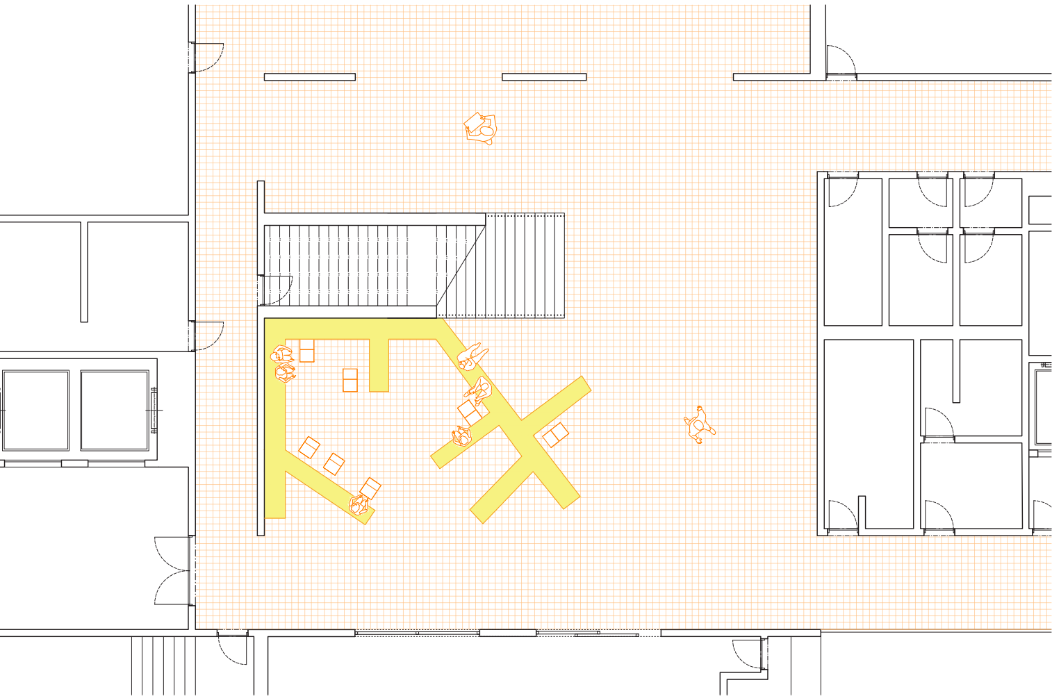
půdorys - atrium jelen M 1:150
