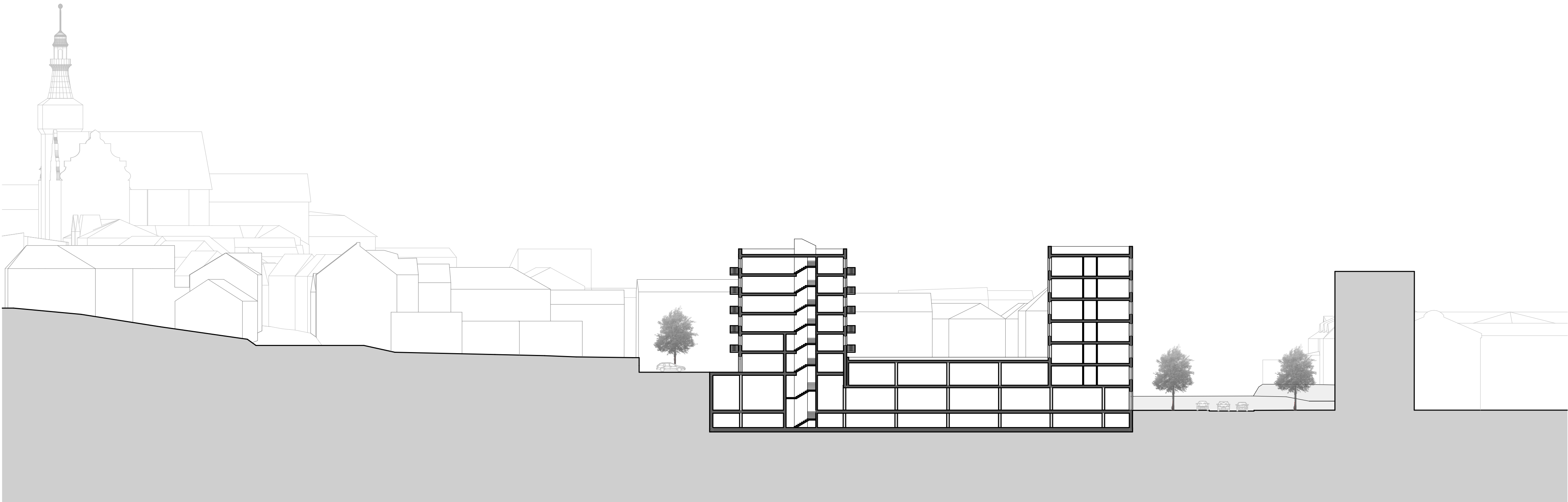
ŘEZOPHLED SEVERNÍ
