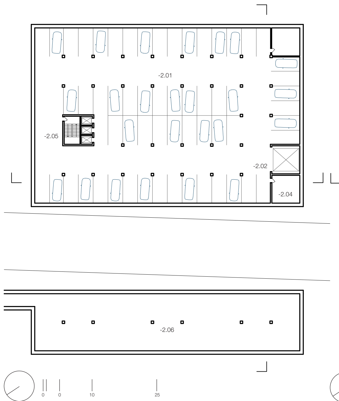
PŮDORYS 2/3 PP
