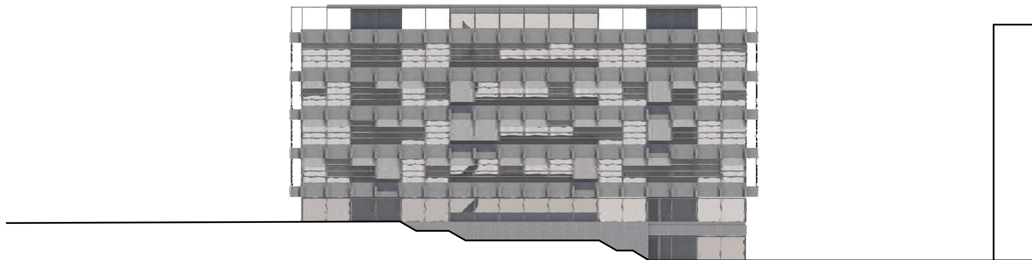
SEVEROVÝCHODNÍ POHLED
