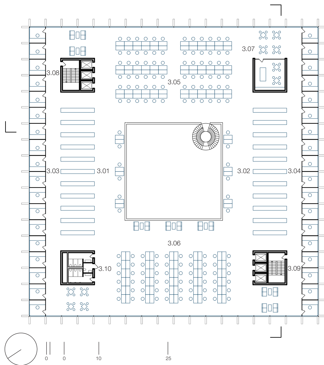
PŮDORYS 3 NP
