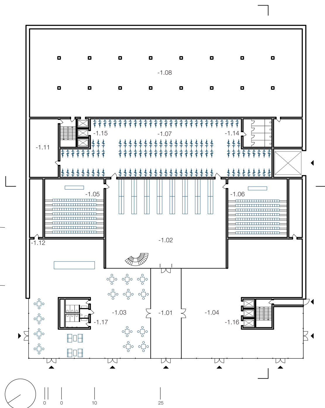
PŮDORYS 1 PP
