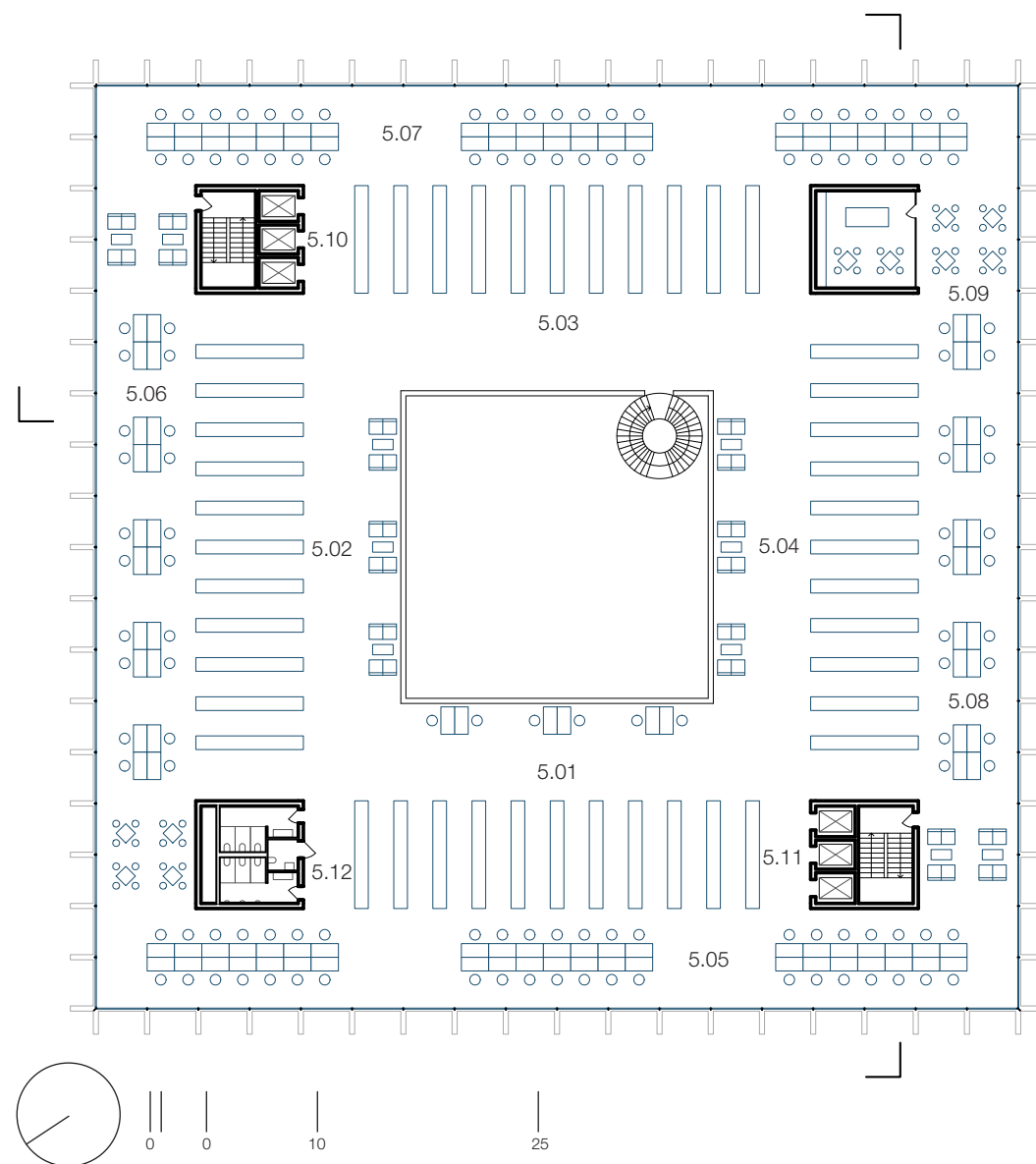
PŮDORYS 5 NP
