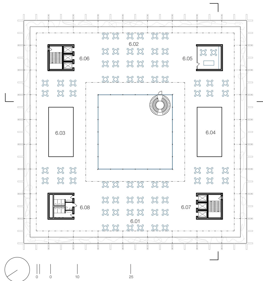
PŮDORYS STŘECHY
