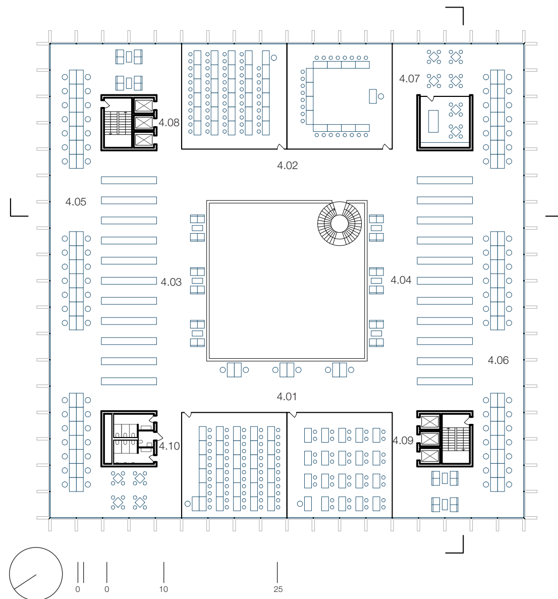
PŮDORYS 4 NP
