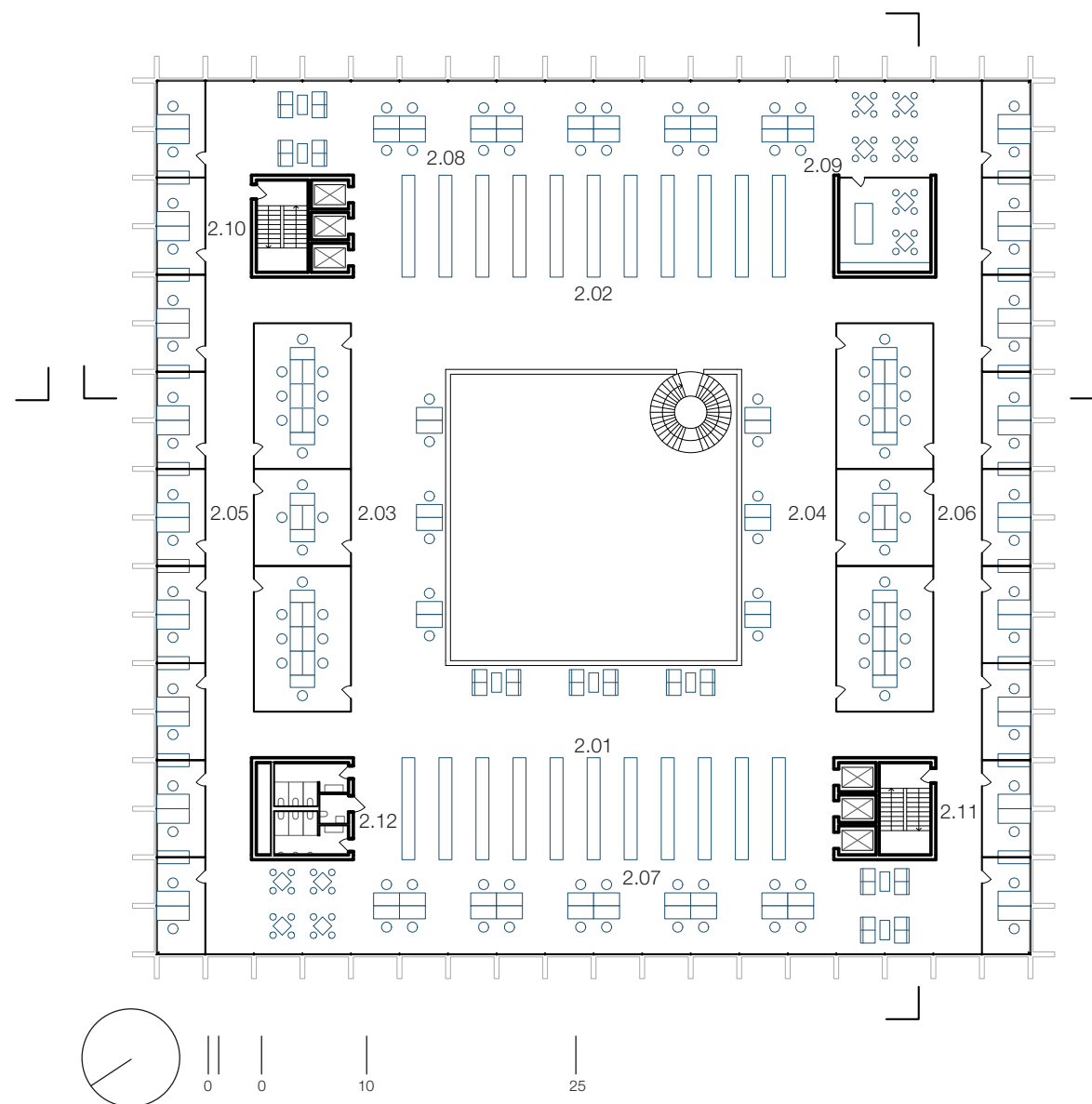
PŮDORYS 2 NP
