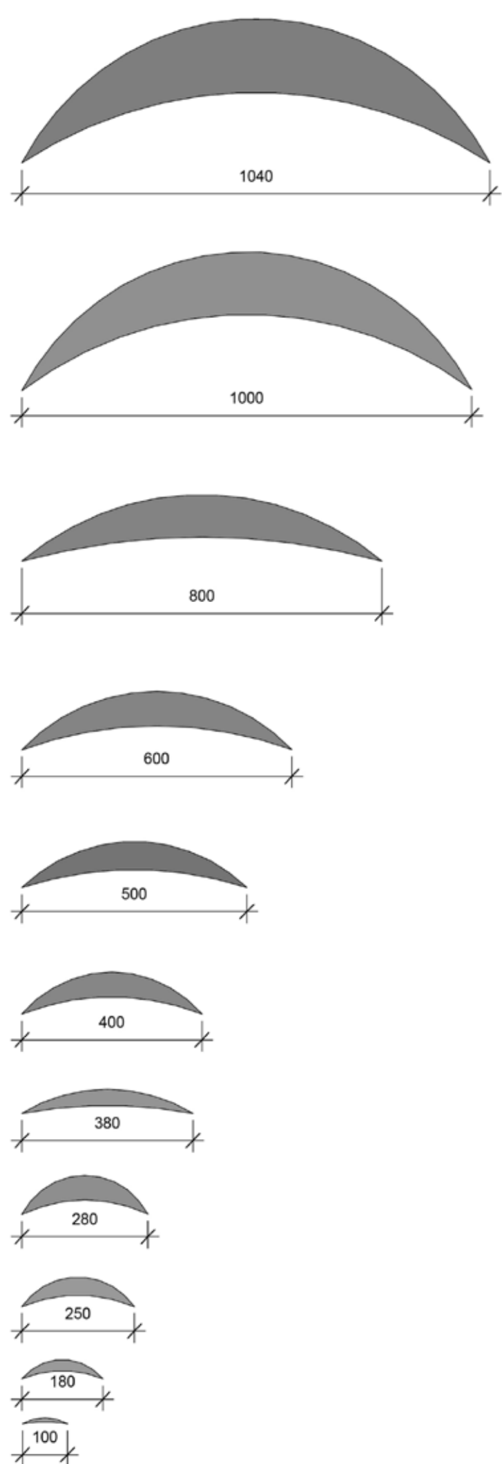
KONSTRUKČNÍ ŘEŠENÍ
