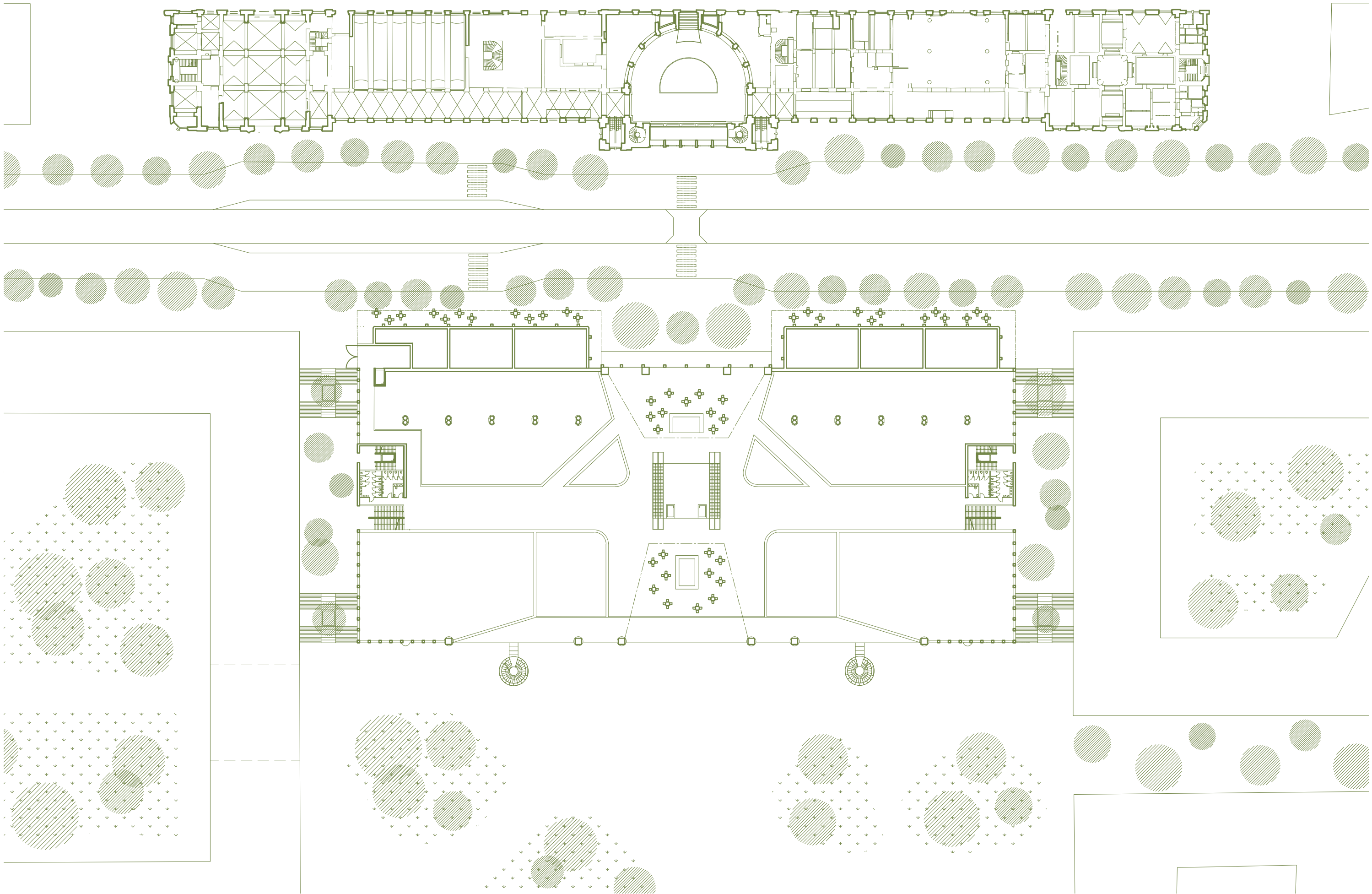
Půdorys úrovně 1, m 1:720
