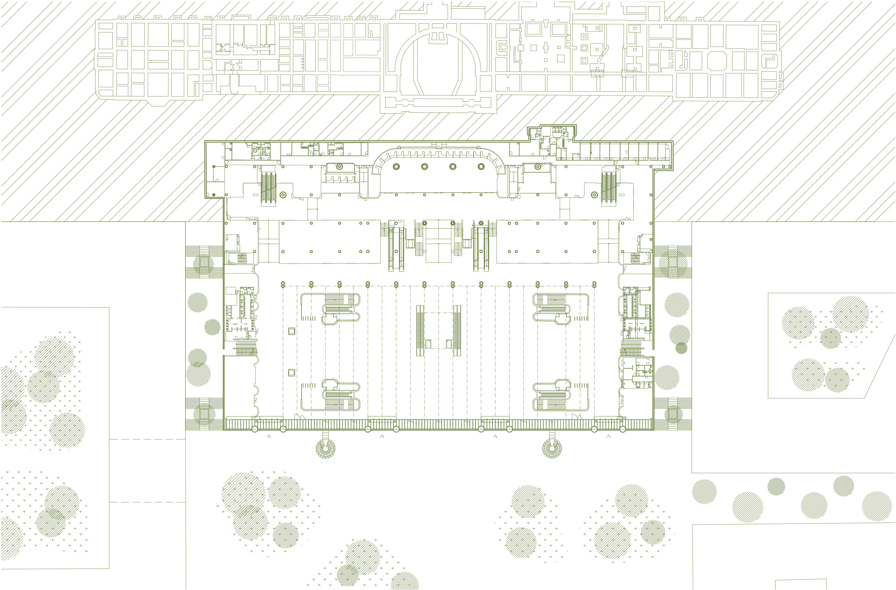
Půdorys úrovně 0, m 1:720
