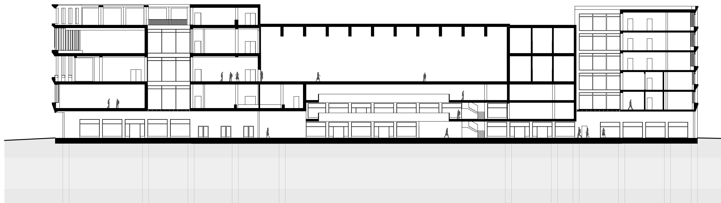
podélný řez
