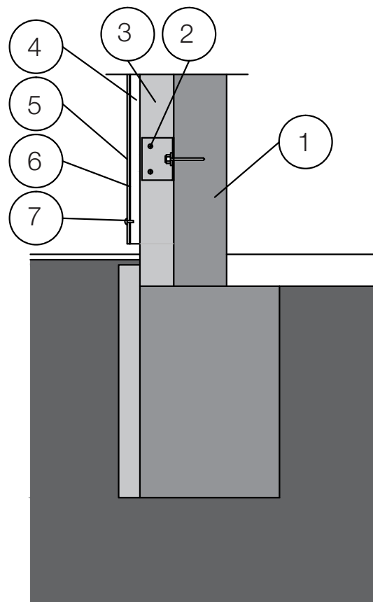
Vertikální řez v oblasti soklu
