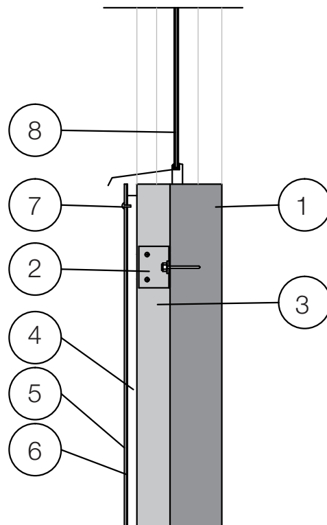
Vertikální řez parapetem okna
