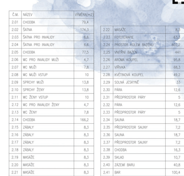
WELLNESS • PUDORYS I.N.
