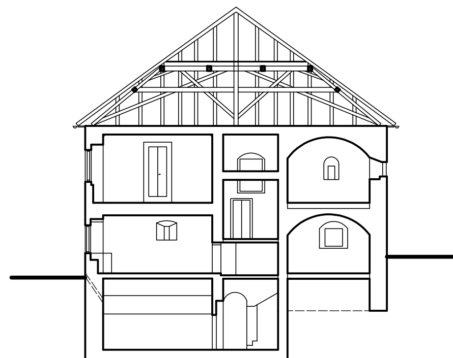
Řez příčný
