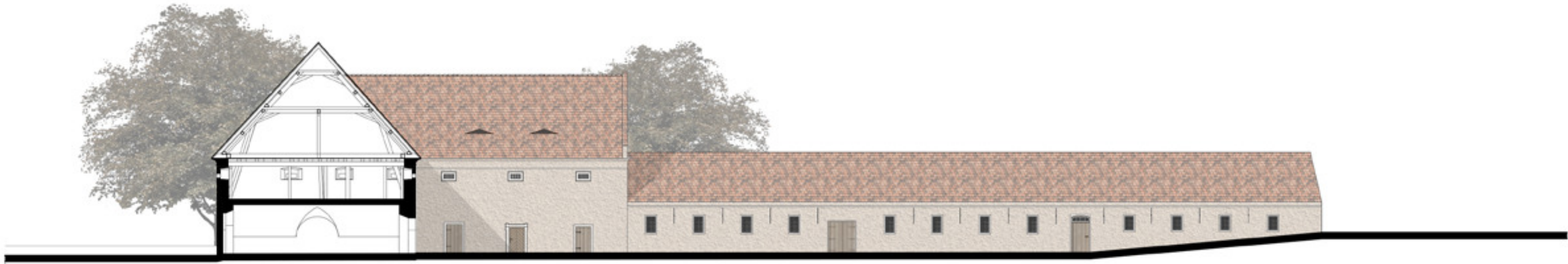
POHLED E - E'
