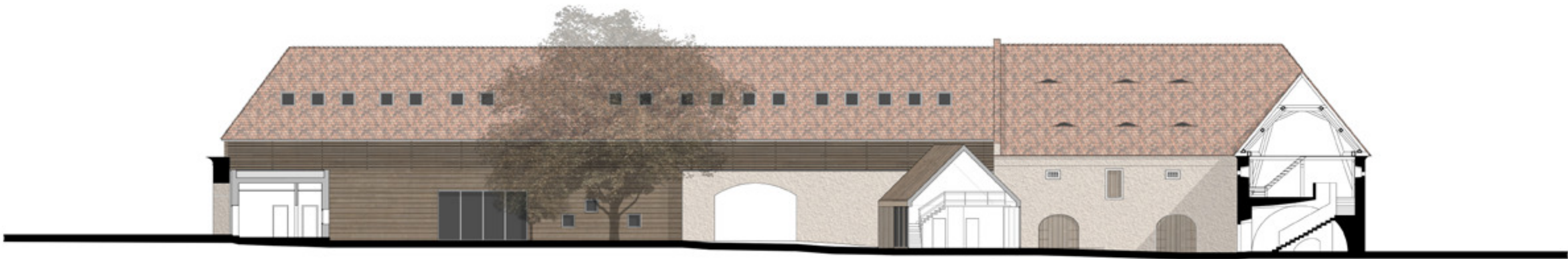
POHLED C - C'
