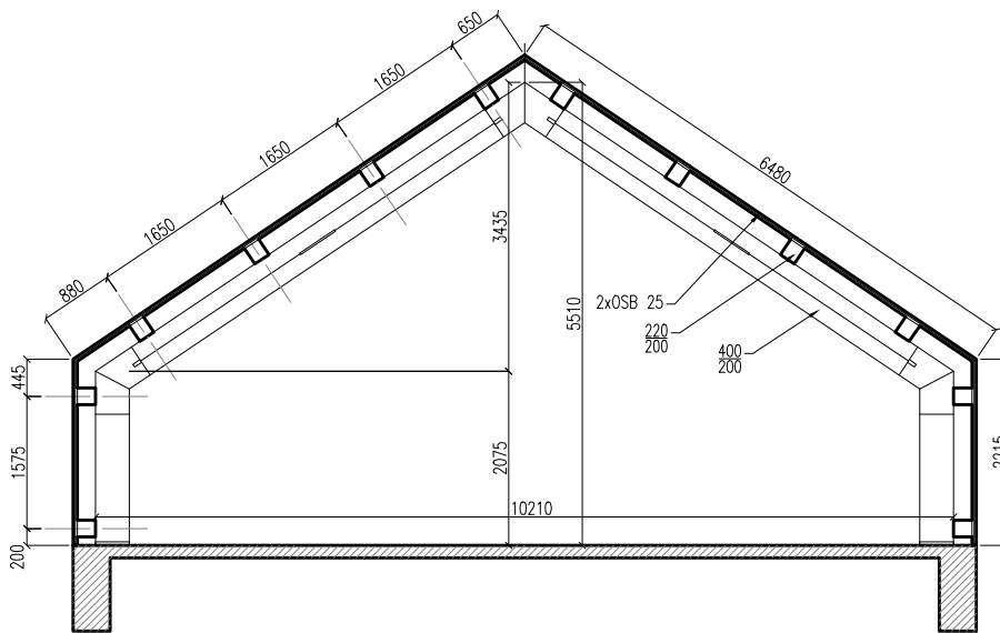
ŘEZ B-B'
