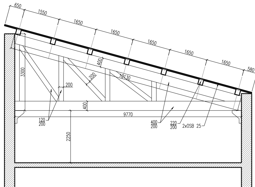
ŘEZ A-A'
