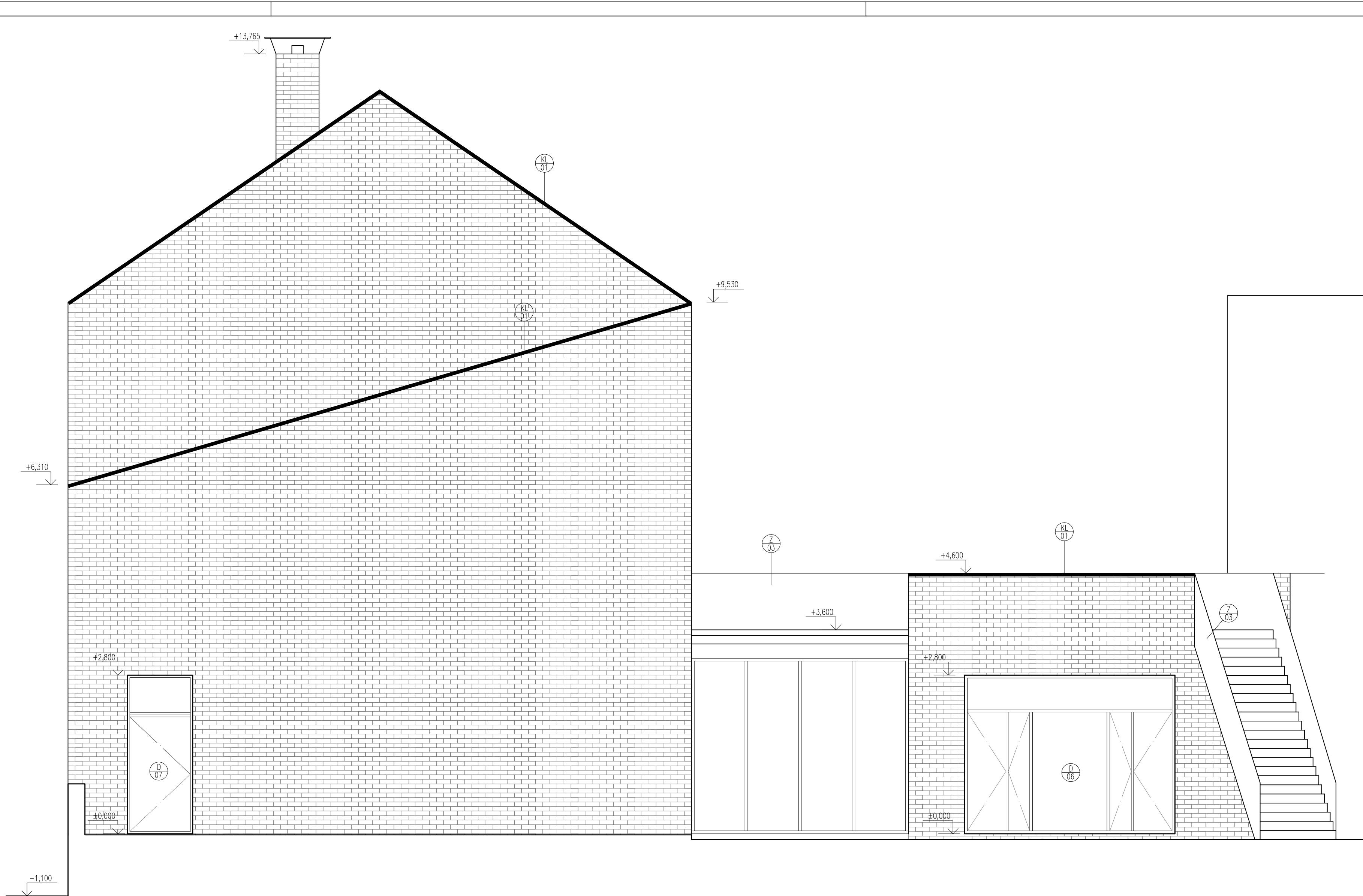
POHLED ZÁPADNÍ
