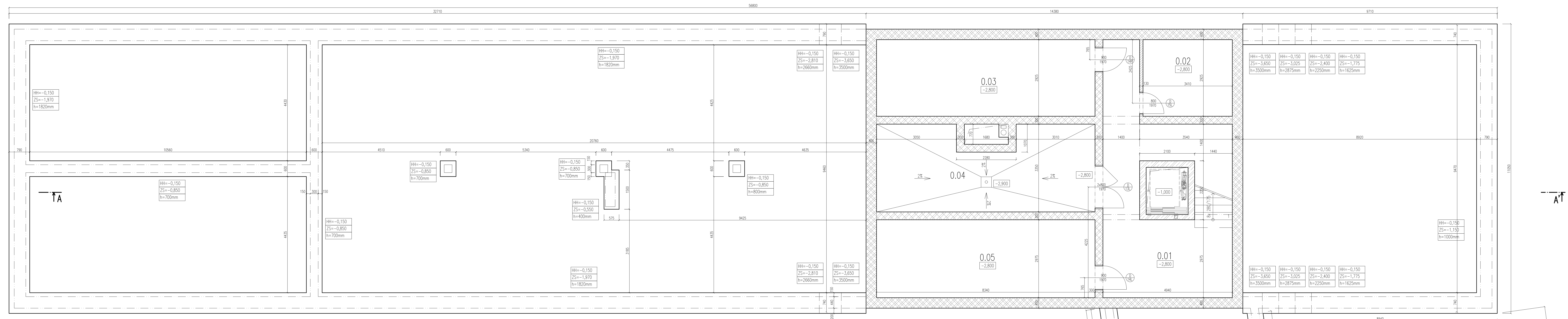
PŮDORYS 1PP, VÝKRES ZÁKLADŮ 1NP
