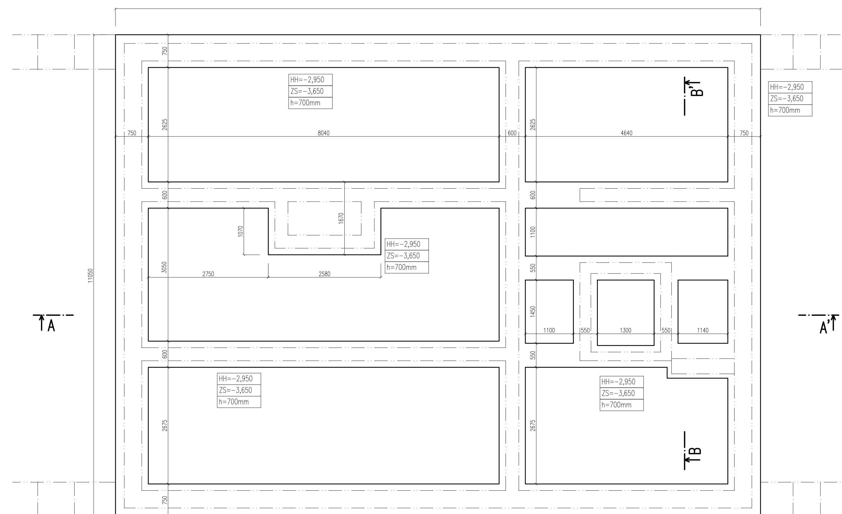
VÝKRES ZÁKLADŮ 1PP
