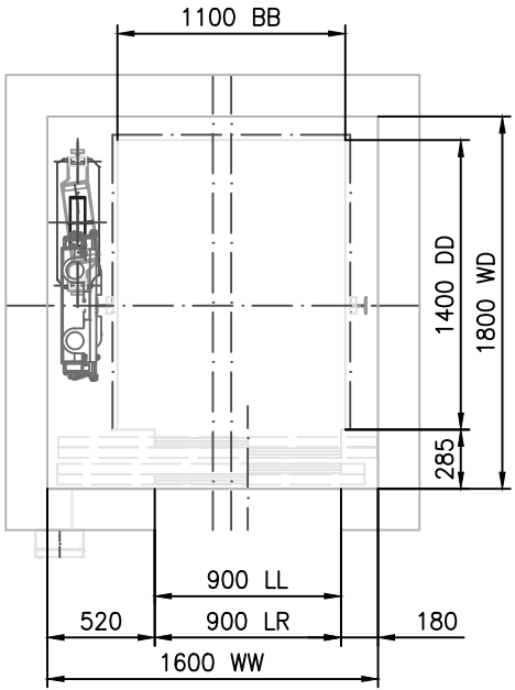
SVETLE VYSKY V HORNÍ ČASTI ŠACHTY
