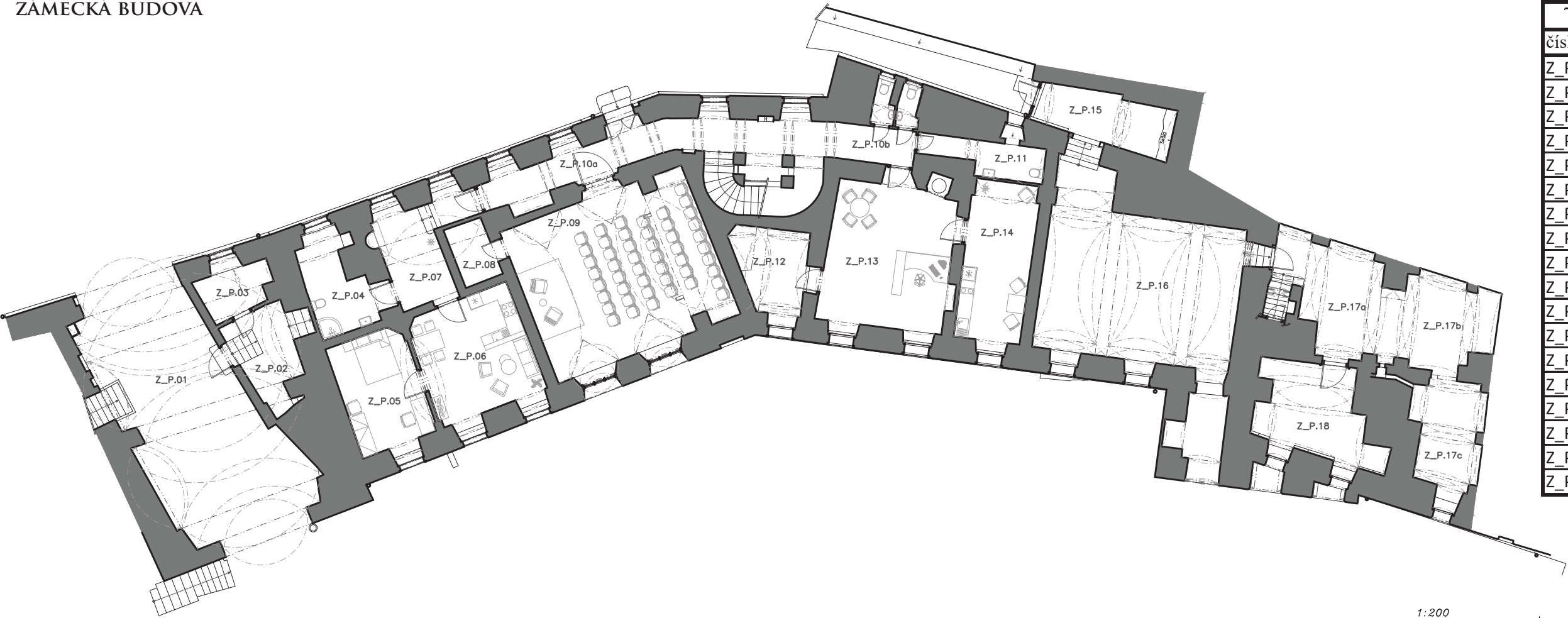
^ půdorys přízemí | M 1:200
