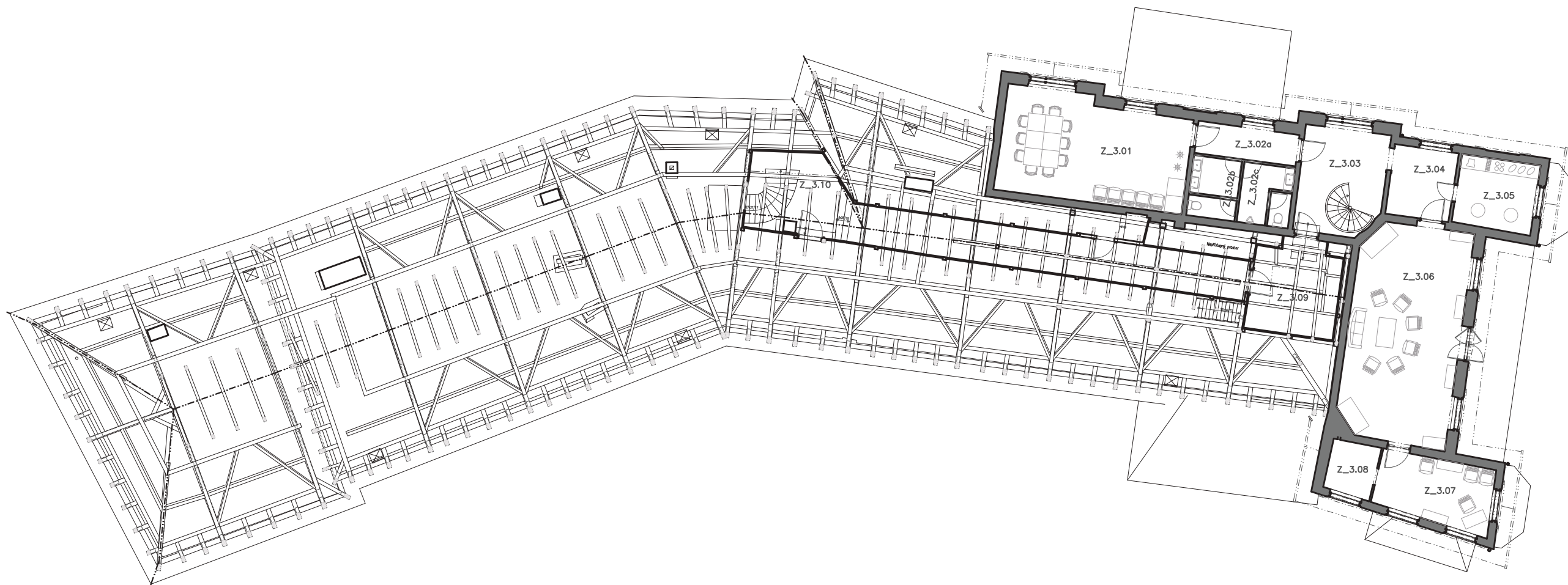
^ půdorys 3. patra a krovu | M 1:200
