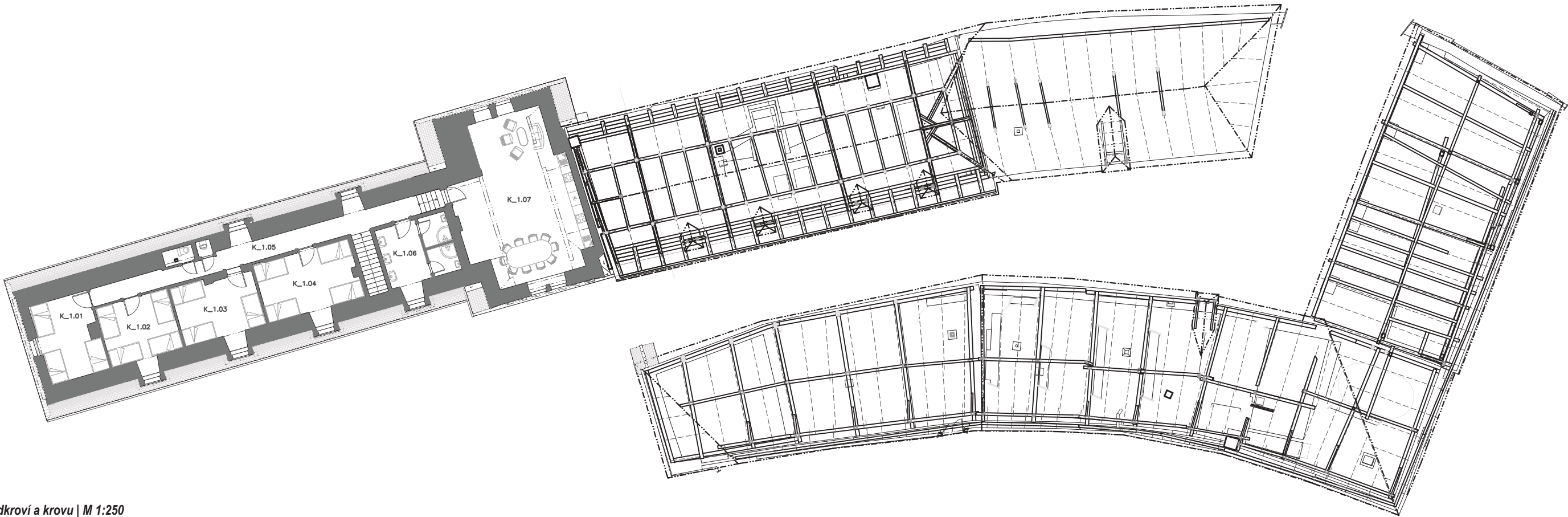
^ půdorys podkroví a krovu | M 1:250
