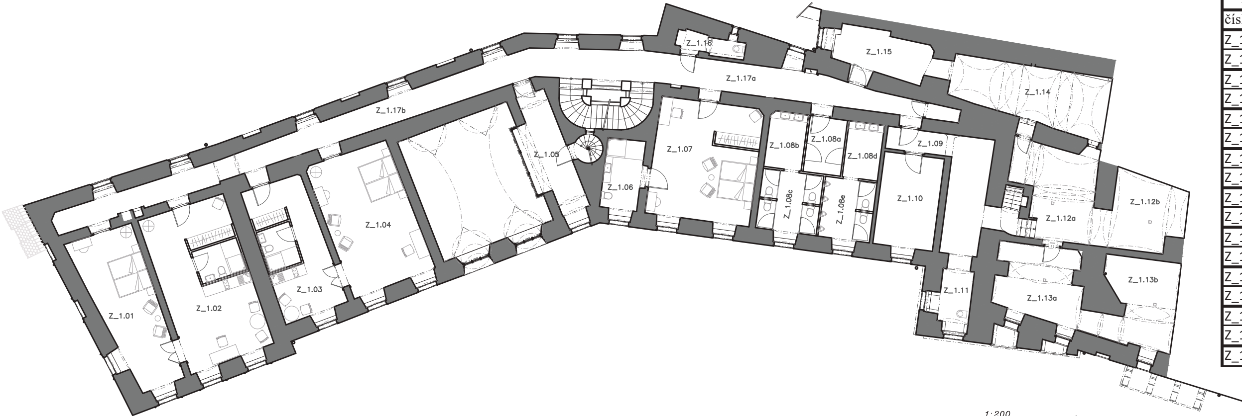
^ půdorys 1. patra | M 1:200
