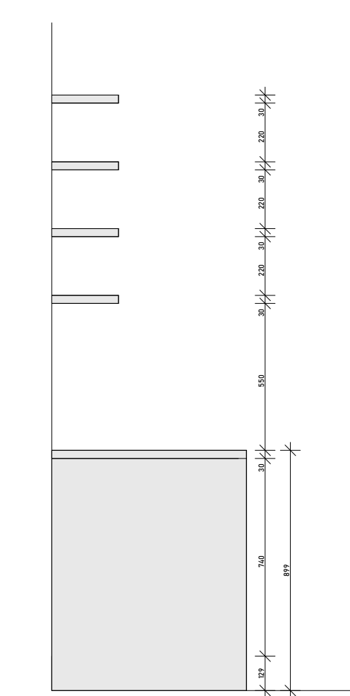
BOČNÍ POHLED NA ZÁBAŘÍ
