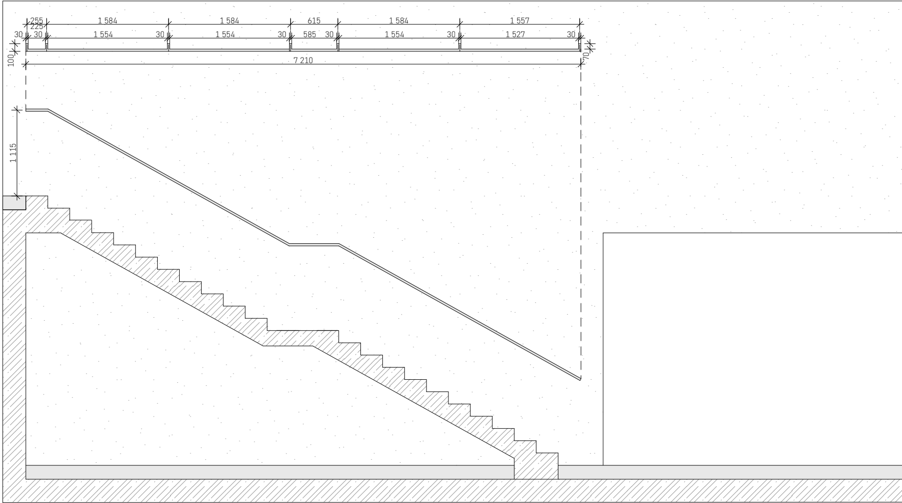
NEREZOVÉ MADLO PROFIL 30x30 MM
