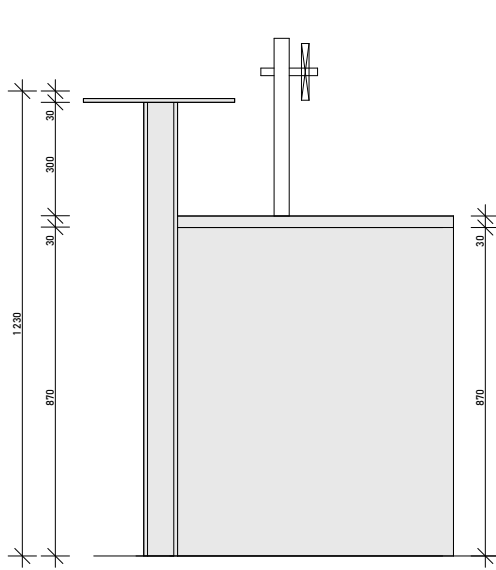
BOČNÍ POHLED NA BAR
