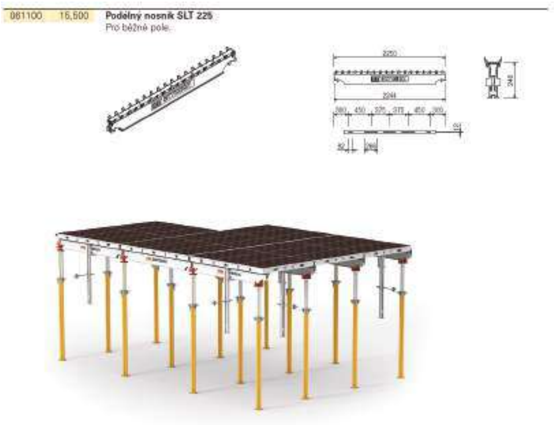
Obrázek 2 – Panelové stropní bednění SKYDECK
