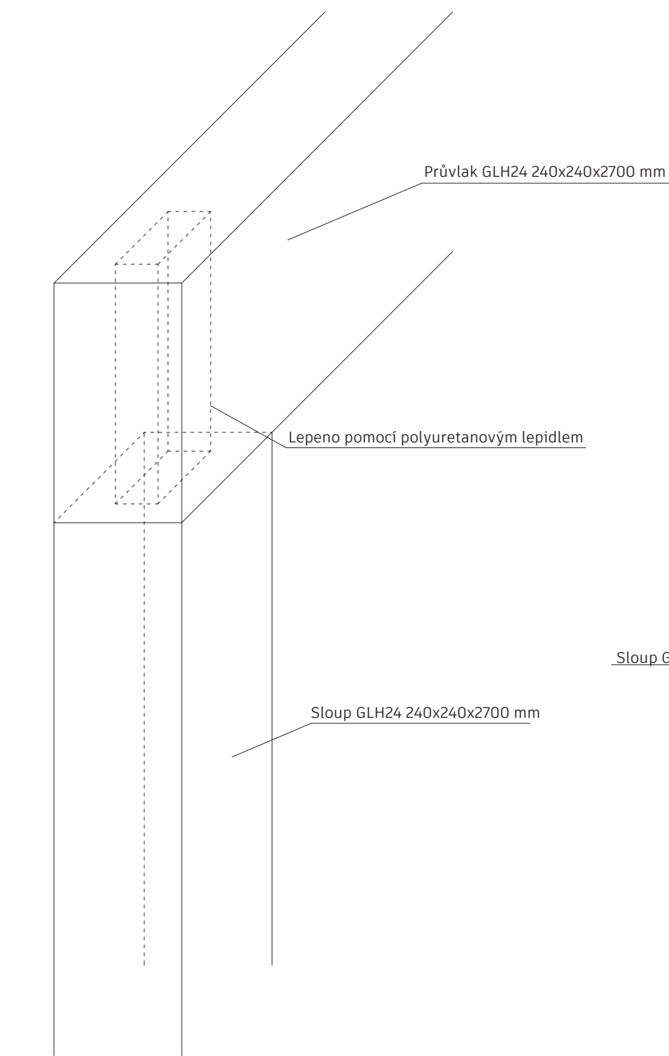
AXONOMETRIE NAPOJENÍ PRŮVLAKU NA SLOUP
