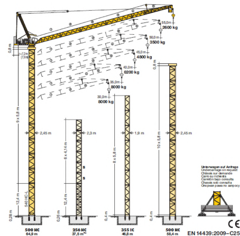
Obrázek 16 - zvolený jeřáb (zdroj: liebherr.com)
