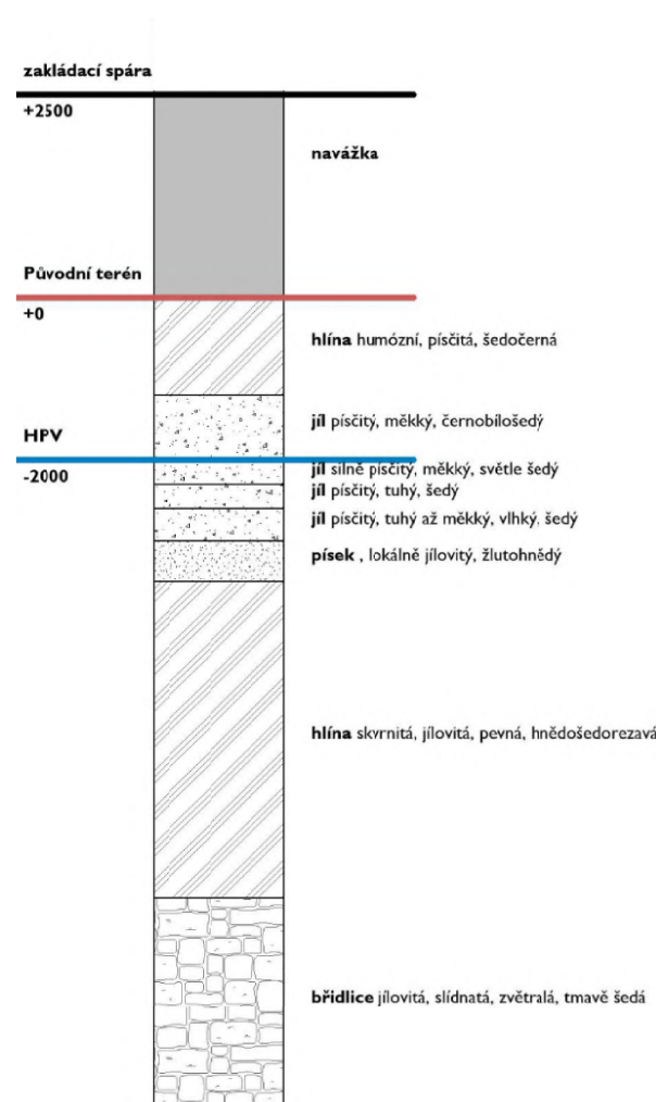
Obrázek 1 – geologický profil terénu, vrt V 2B [GDO 582030]
