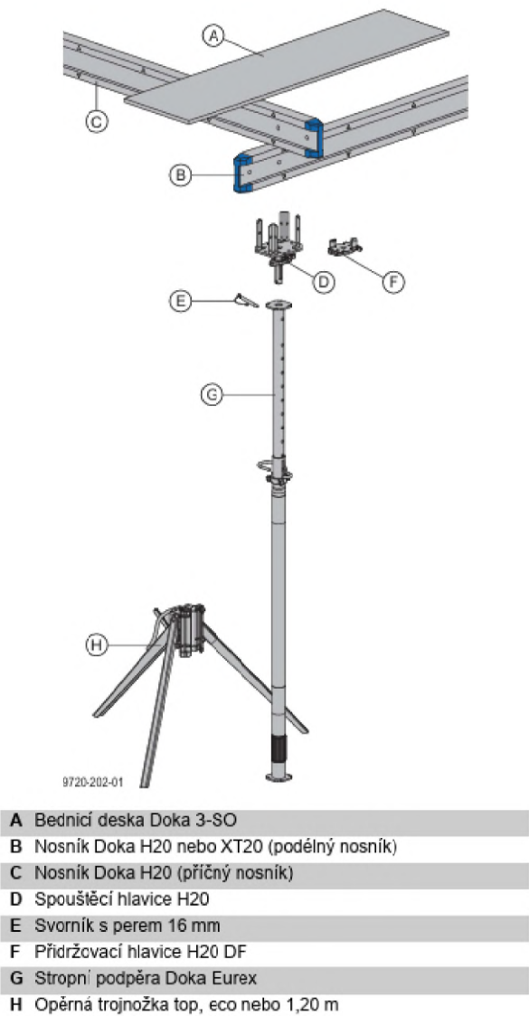
Obrázek 10 - prvky bednění (zdroj doka.com)
