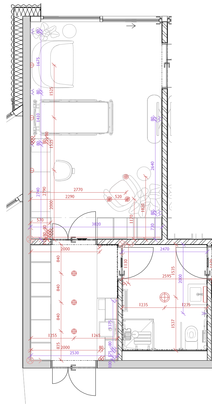
půdorys elektro I : 50
