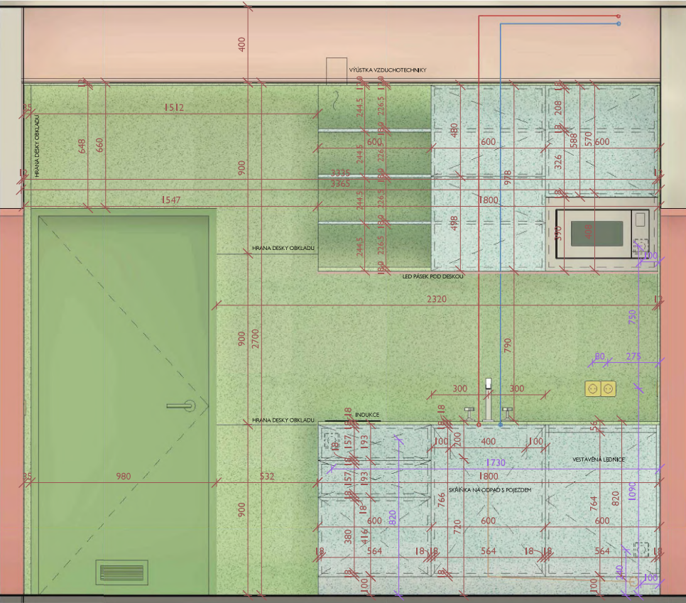
pohled VN3 I : 20
