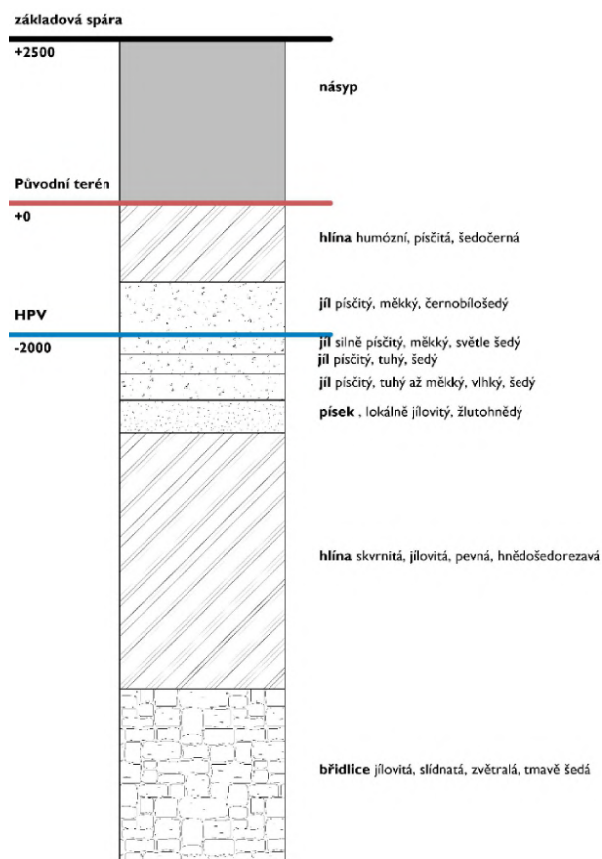
Obrázek 1 – geologický profil terénu, vrt V 2B [GDO 582030]
