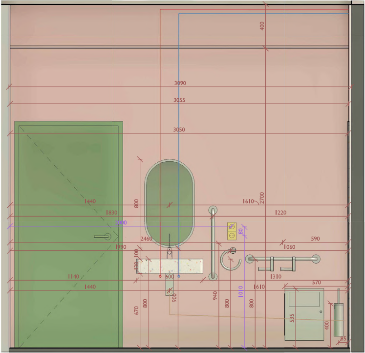
pohled 1 1 : 20
