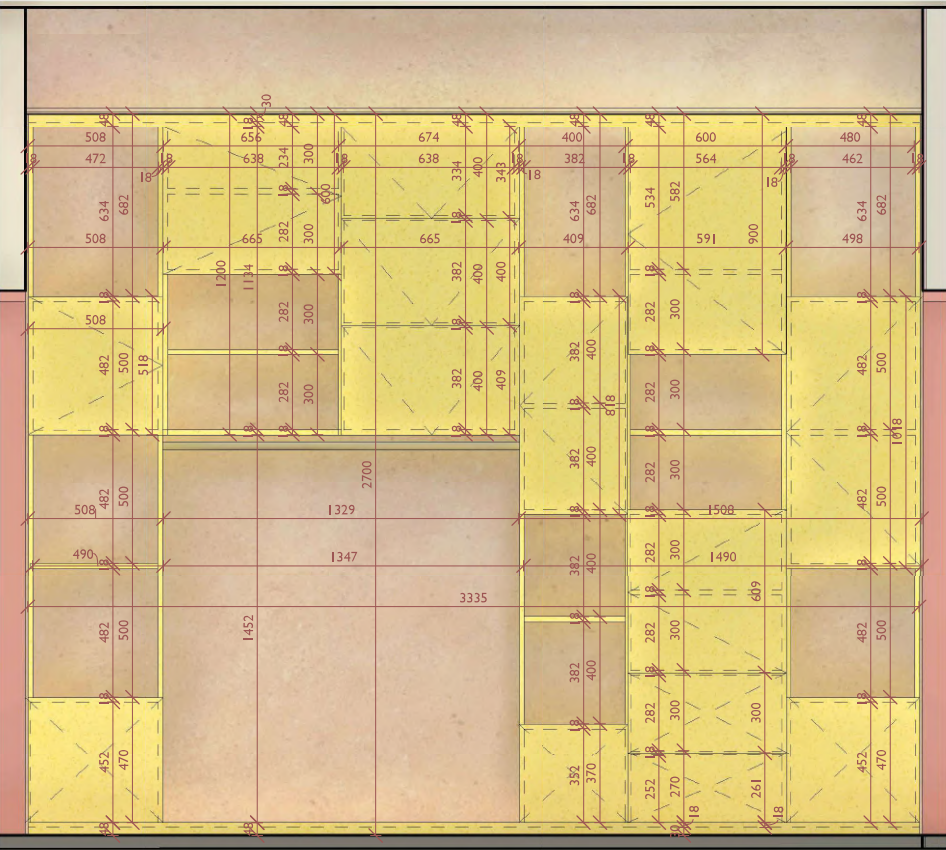
pohled VN2 I : 20
