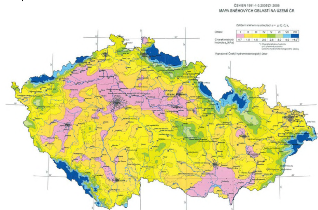
Obrázek 2 - sněhové oblasti
