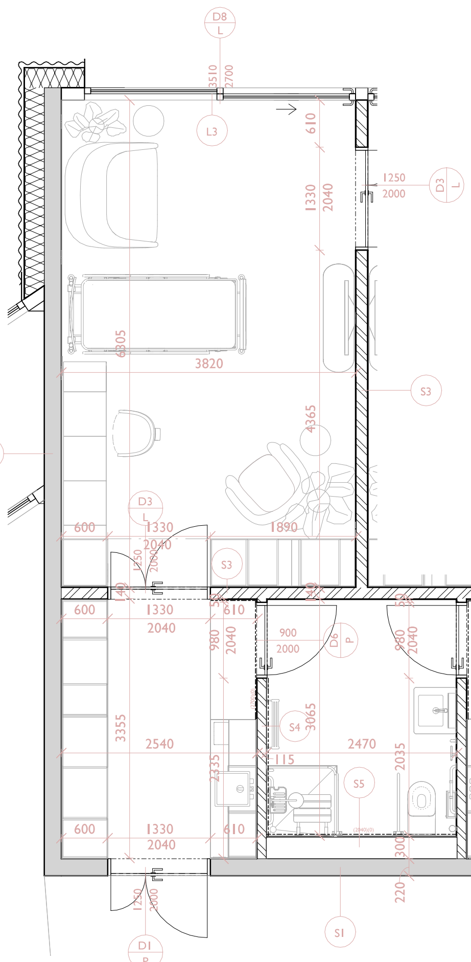
stavařský půdorys 1 : 50
