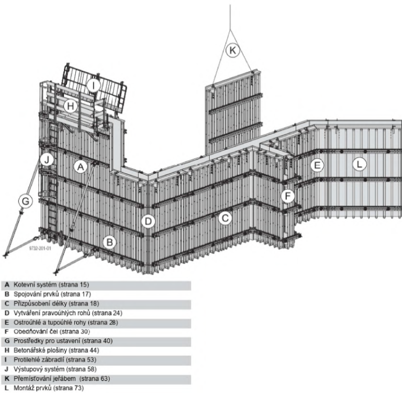
Obrázek 11 - výpis materiálu bednění (zdroj doka.com)
