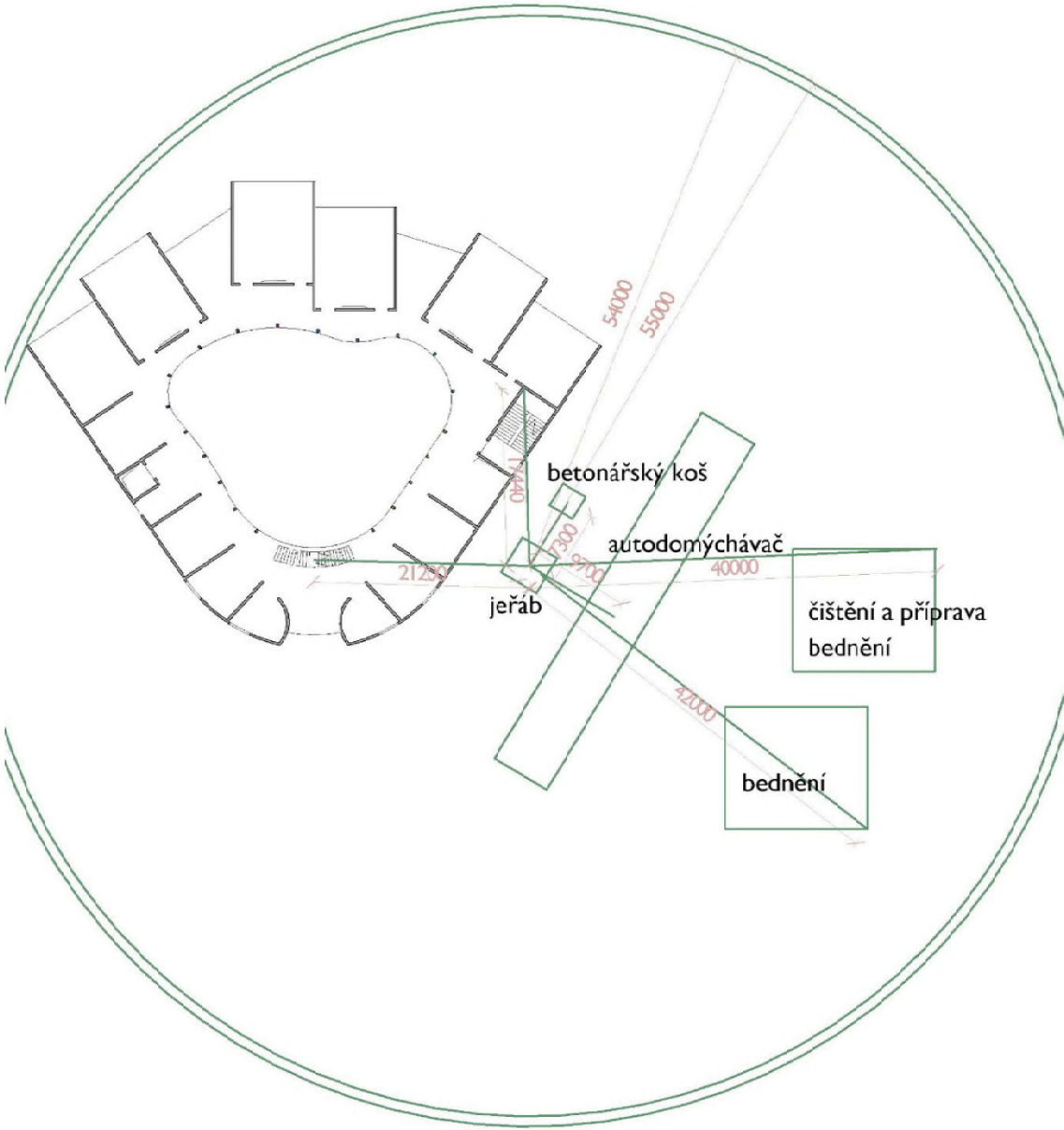
Obrázek 18 - půdorys jeřábu na pozici ve staveništi
