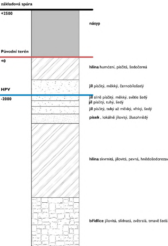
Obrázek 2 – geologický profil terénu, vrt V 2B [GDO 582030]
