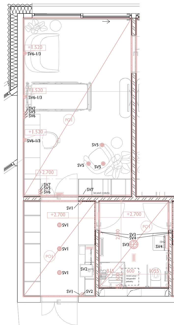
podhledy I : 50
