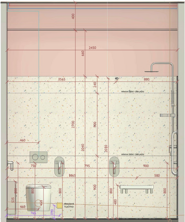
pohled 2 1 : 20
