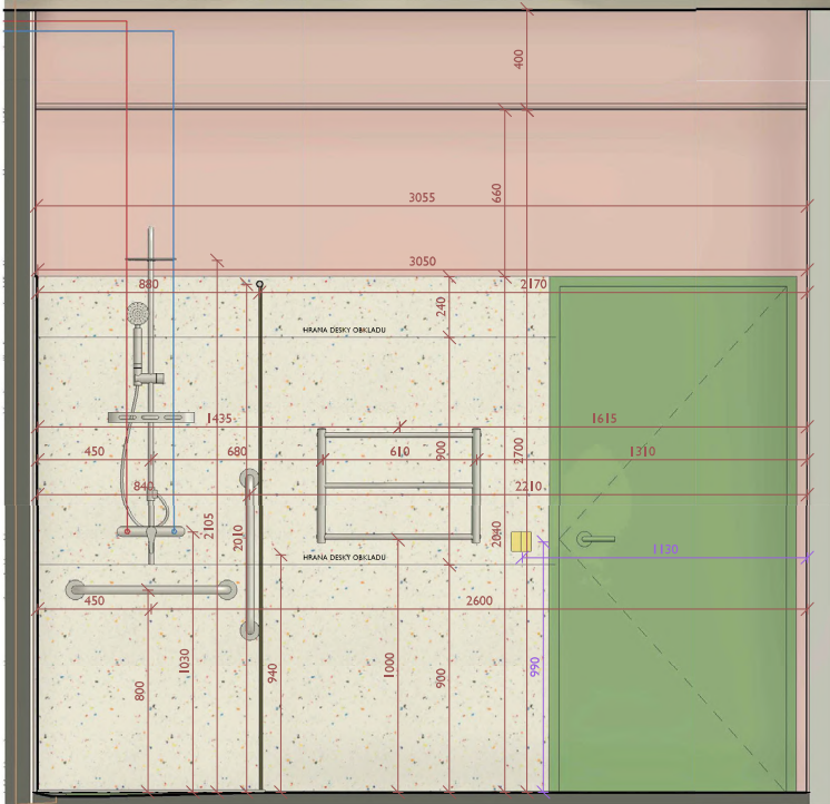
pohled 3 1 : 20
