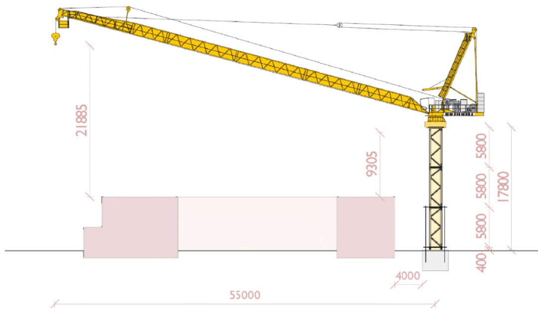
Obrázek 19 - řez jeřábem
