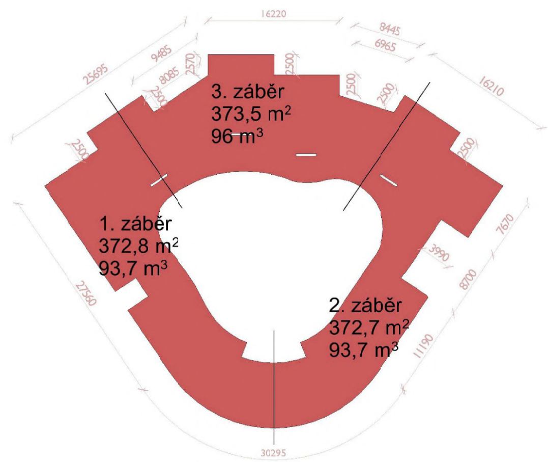
Obrázek 7 - záběry vodorovné konstrukce
