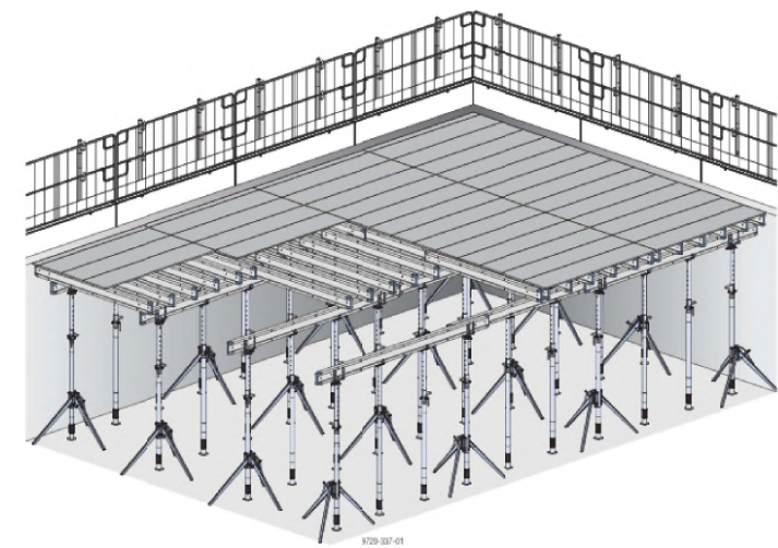
Obrázek 9 - bednění stropů Dokaflex I-2-4 (zdroj doka.com)
