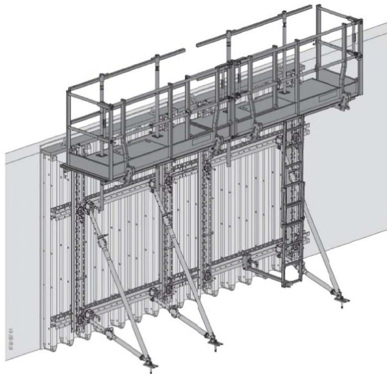
Obrázek 12 - nosíkové bednění stěn (zdroj doka.com)
