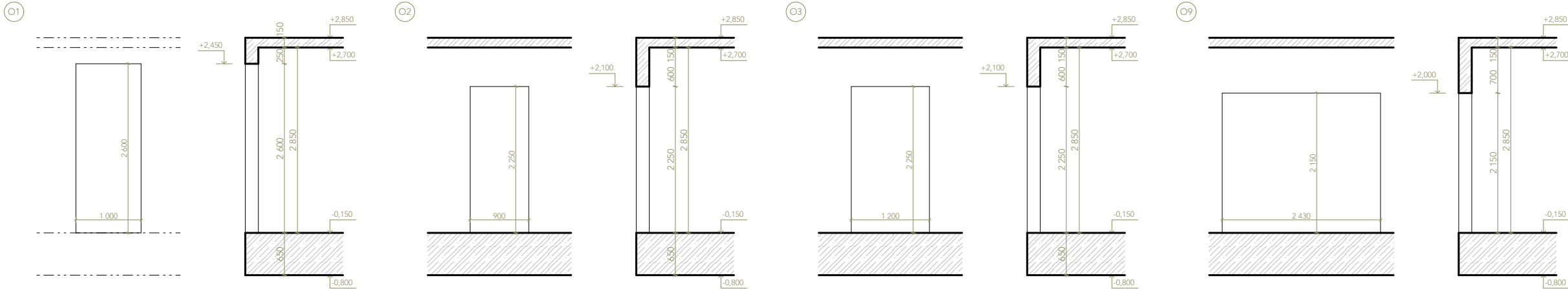
SCHÉMA OTVORŮ M 1:75
