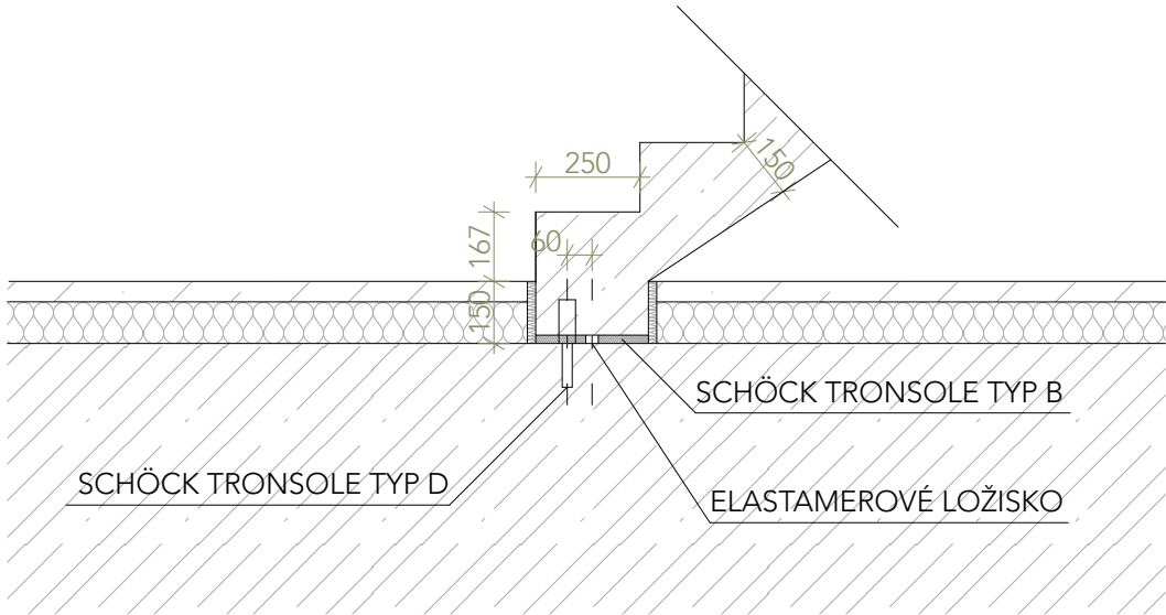
DETAIL OSAZENÍ PREFABRIKOVANÉHO SCHODIŠTĚ NA DESKU M 1:20
