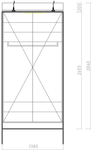
POHLED D
