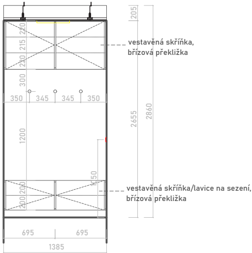
POHLED B
