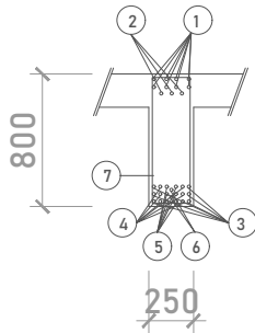
ŘEZ A
