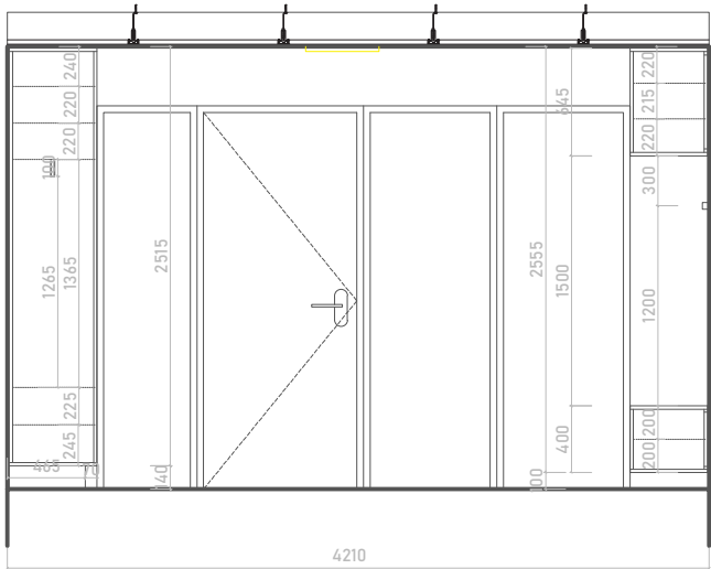
POHLED A
