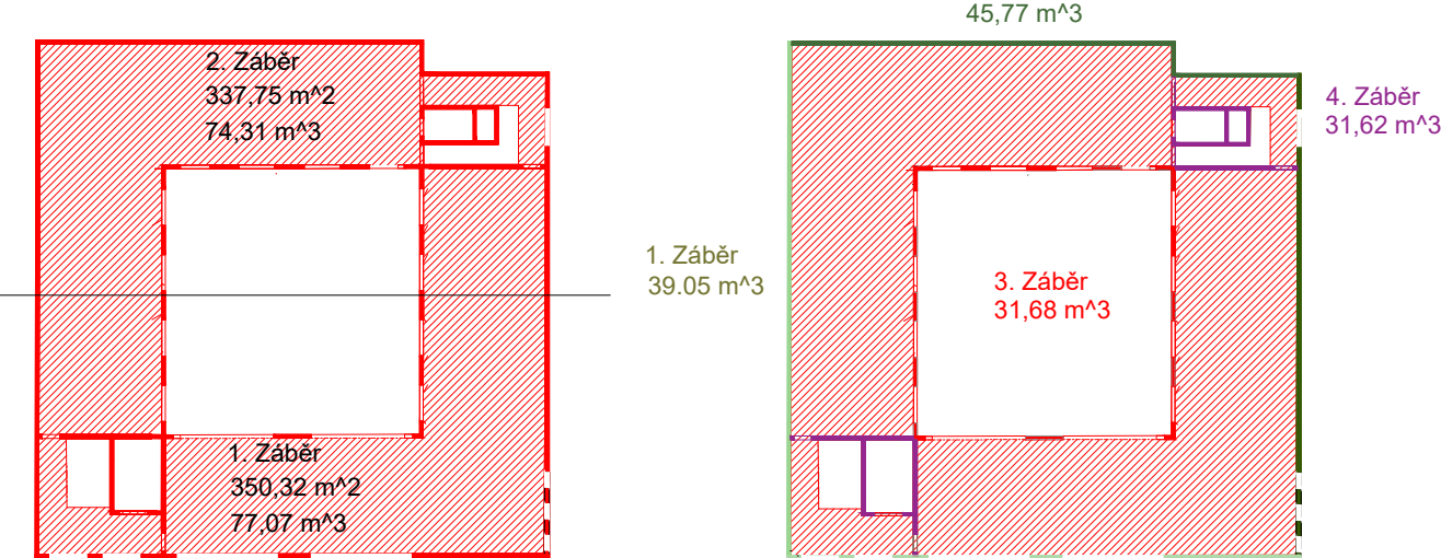
Obr.č.4. vodorovní bednění, záběry
