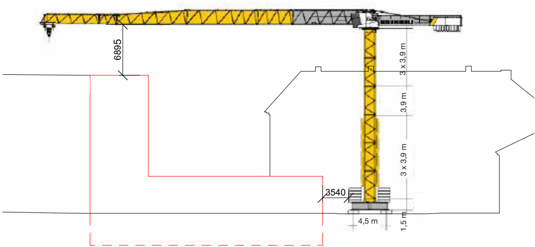
Obr.č. 19. Limity pro užití jeřábu Liebherr 125 EC - B6
