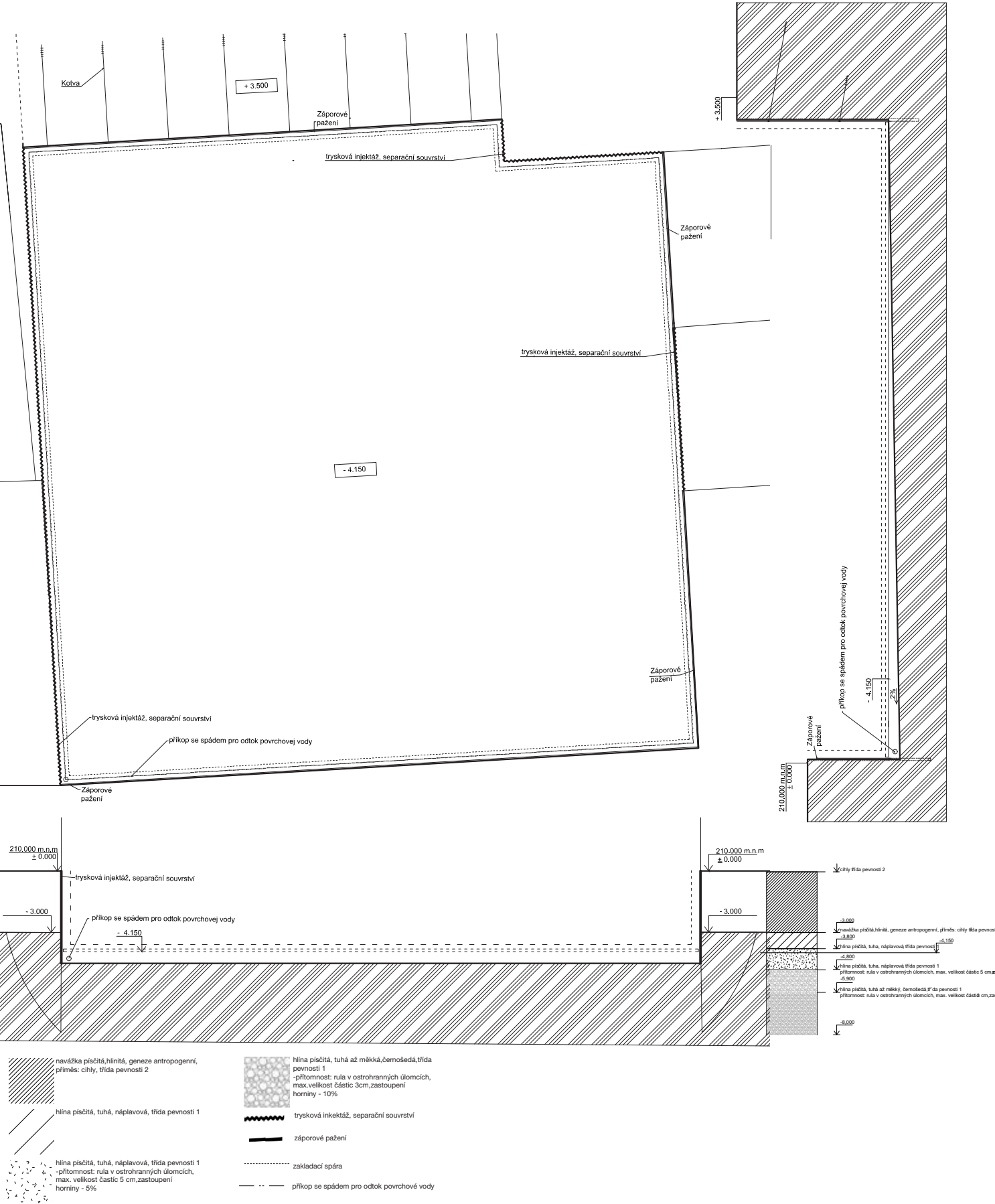
Obr.č.2 : Schématický řez a půdorys stavební jámy
