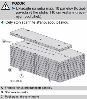
Obr.č.11. DOKAXlight ukladaní bednění do stohů
