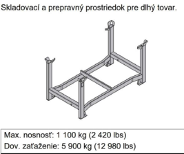
Obr.č.16. Dokadek 30ukladací paleta
