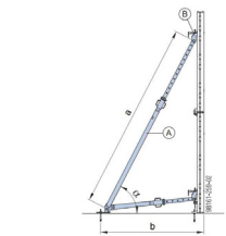
Obr.č.7. DOKAXlight panalová opěra
