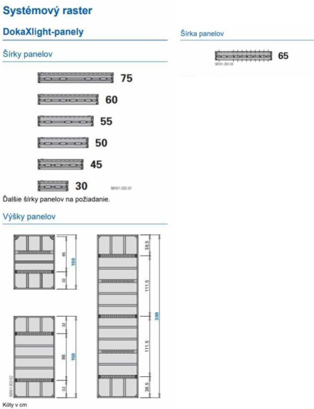
Obr.č.9. DOKAXlight systémový rastr
