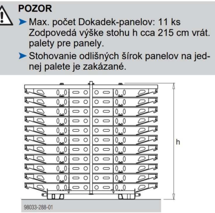
Obr.č.15.Dokadek 30 balení panelů
