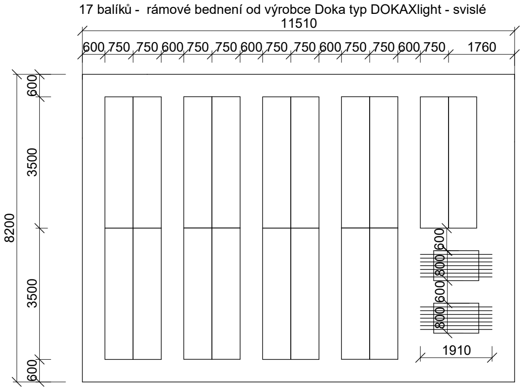
Obr.č.17 : Schématické půdorysy návrhu skladovacích ploch
