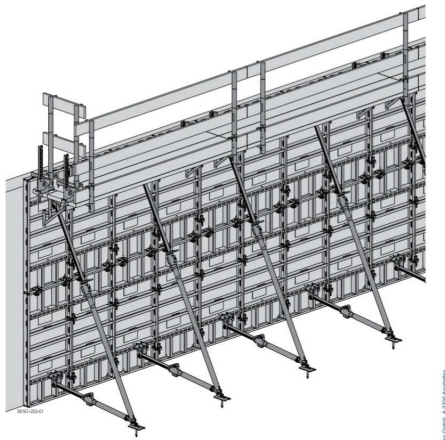
Obr.č.6. rámové bednění od výrobce Doka
