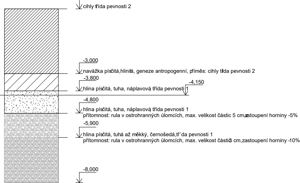
Obr.č.1: Půdní profil v řezu
