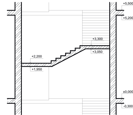
S1 ŘEZ
