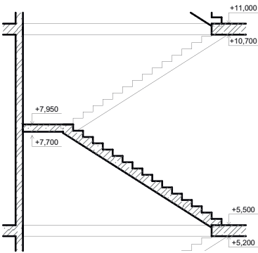
S2 ŘEZ
