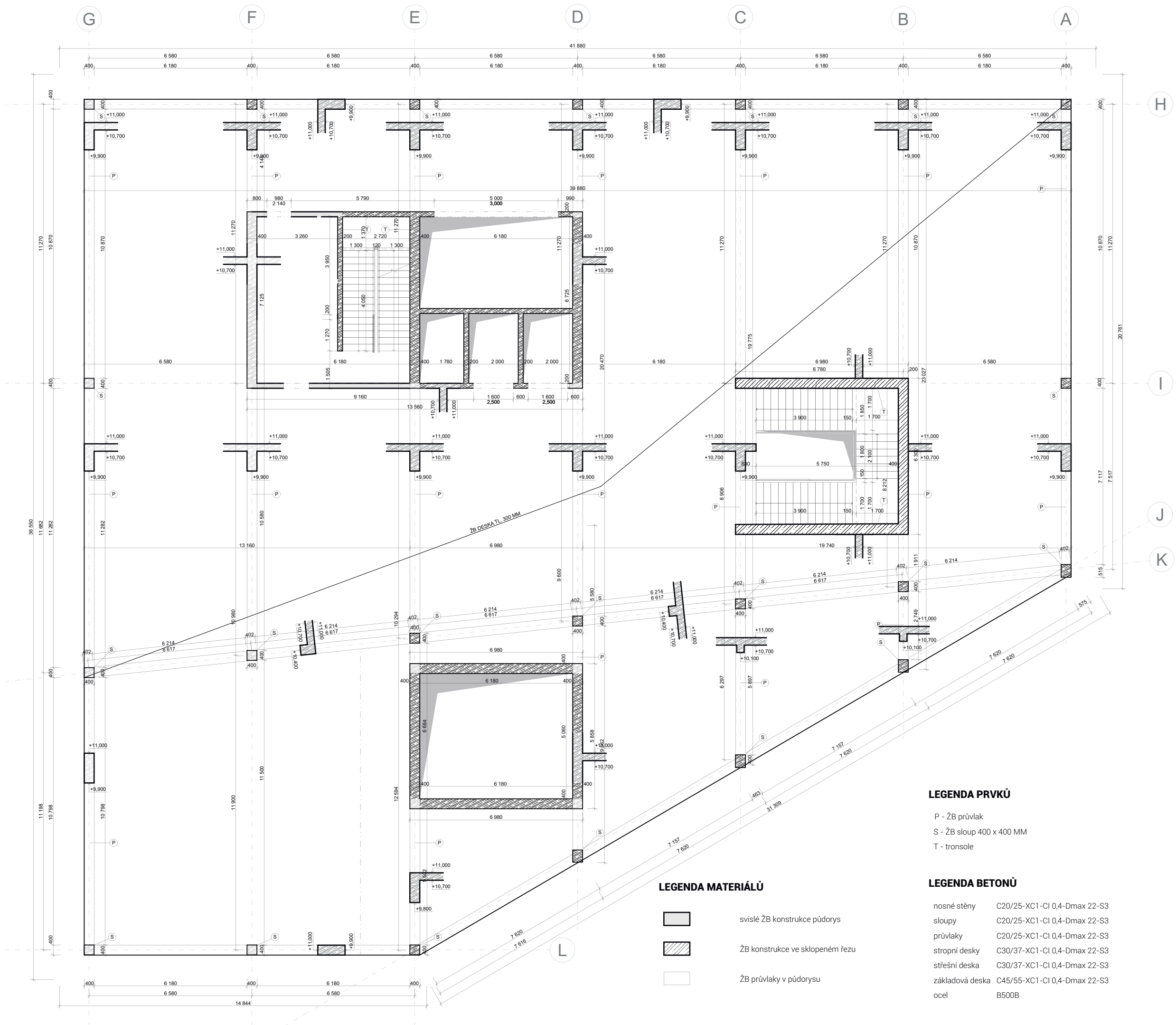
S2 PŮDORYS
