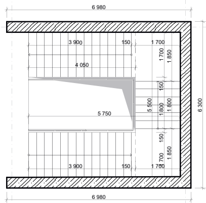
S1 PŮDORYS
