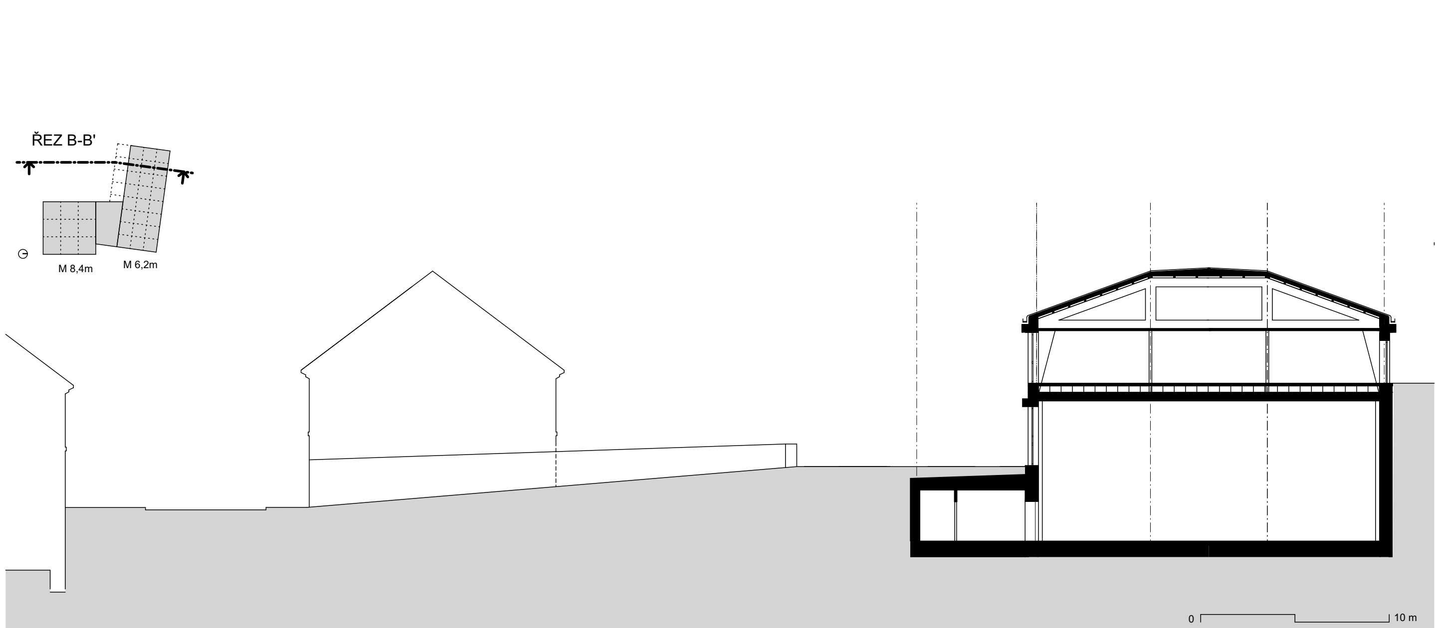
ŘEZ B-B'
