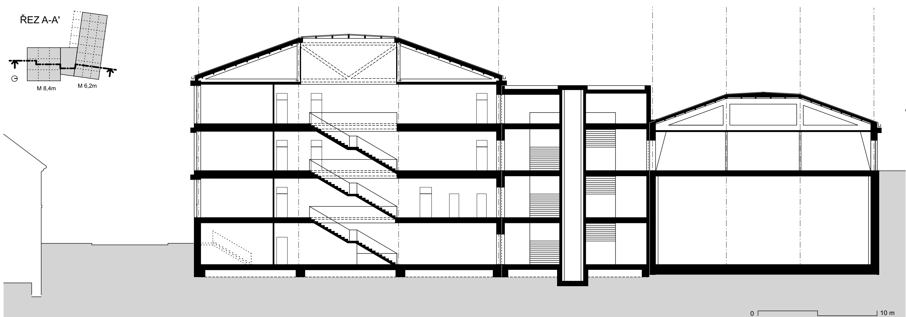
ŘEZ A-A'
