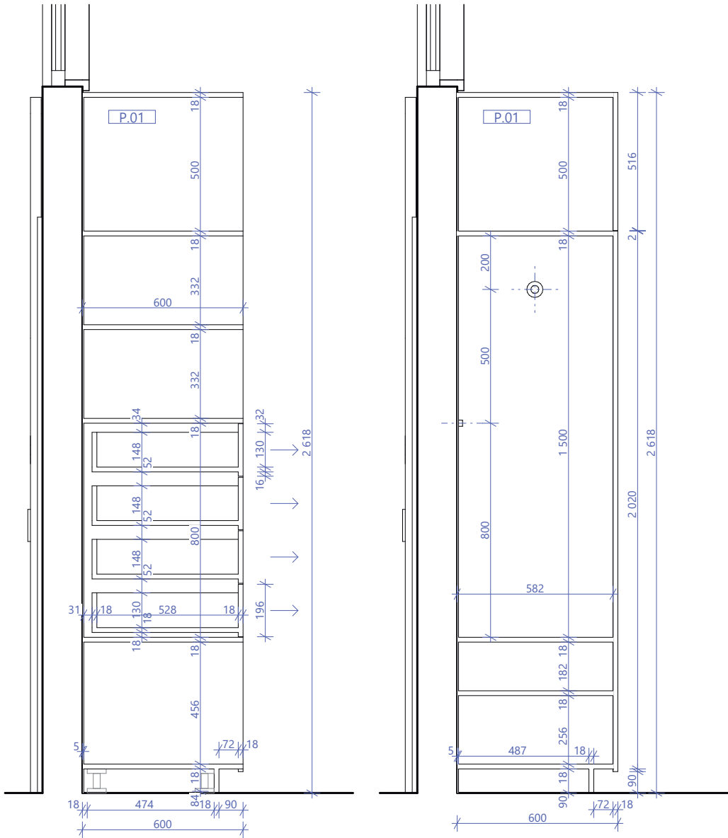
ŘEZ SKŘÍNÍ AA'
