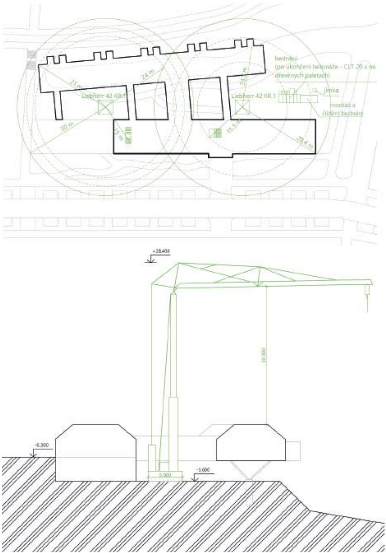
D.5.A.5. ZAŘÍZENÍ STAVENÍŠTĚ
