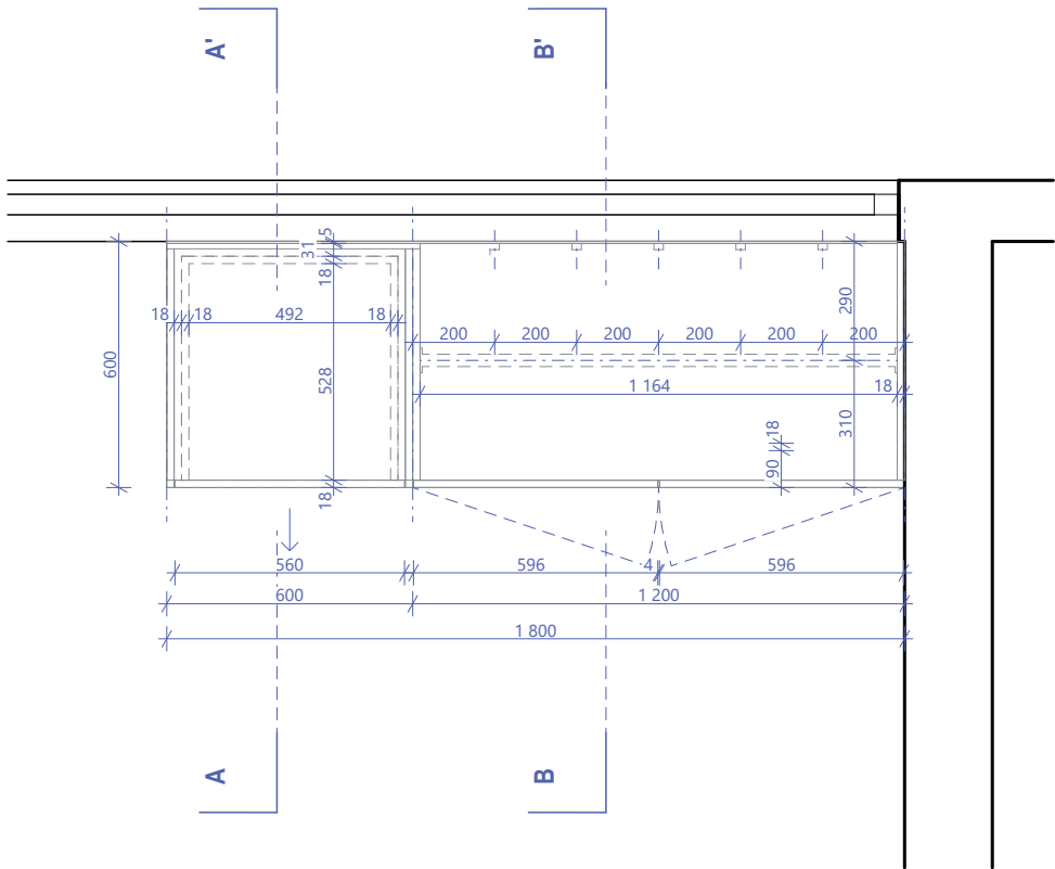
PŮDORYS SKŘÍNĚ
