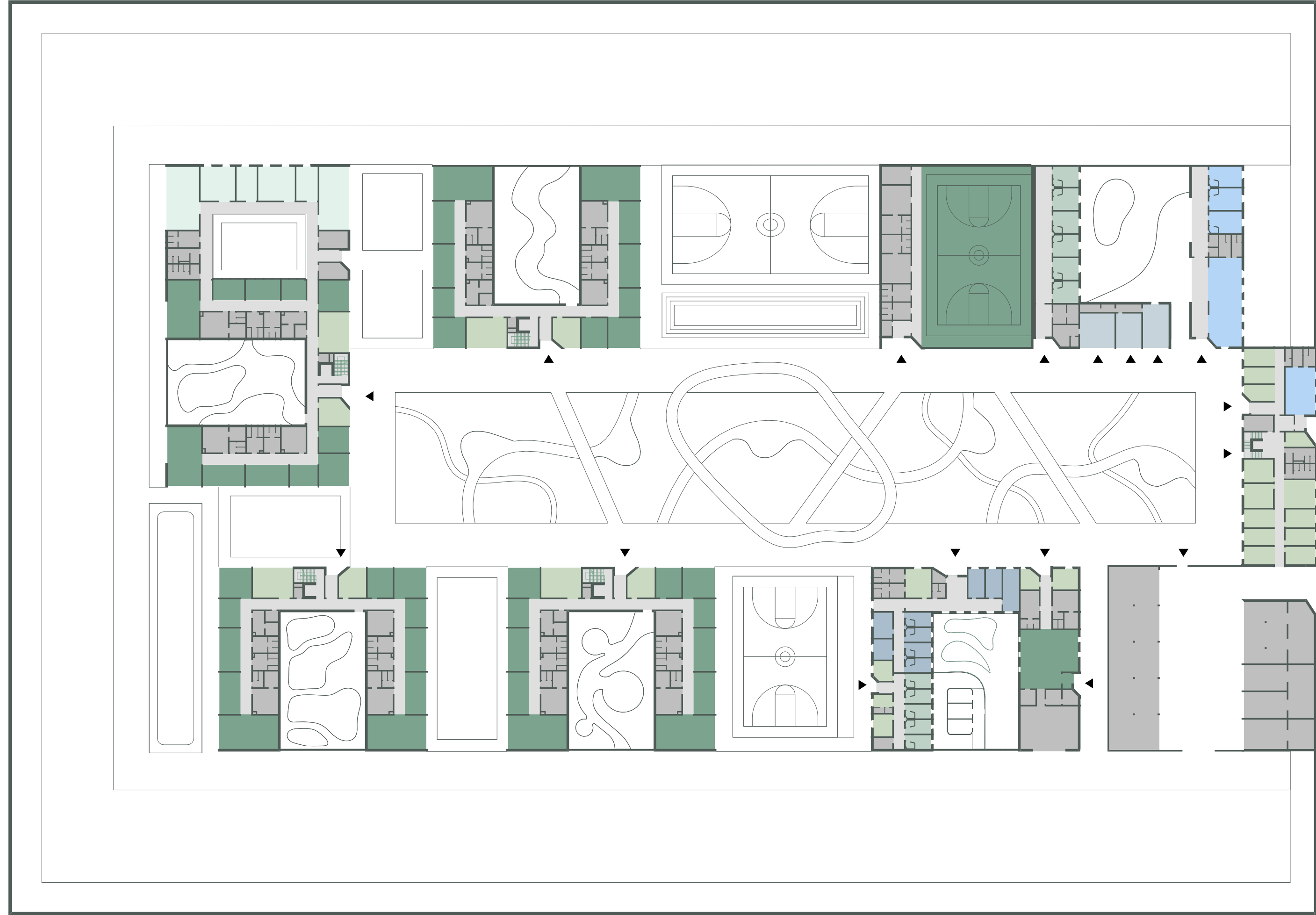
FUNKČNÍ SCHEMA - 1.NP
