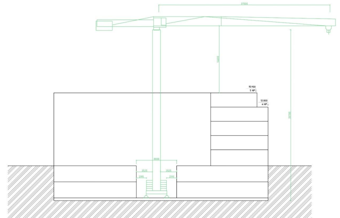
Zobrazení polohy a rozsahu jeřábu na staveništi – půdorys
