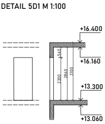
D1 DETAIL 5D1 M 1:100
