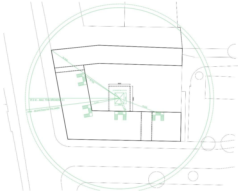
Zobrazení polohy a rozsahu jeřábu na staveništi – půdorys
