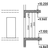
D1 DETAIL 3D1 M 1:100
