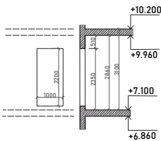
O4 DETAIL 304 M 1:100
