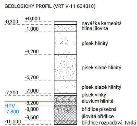
Obrázok D.2.1.1.3. – Geologický profil V-11 634318
