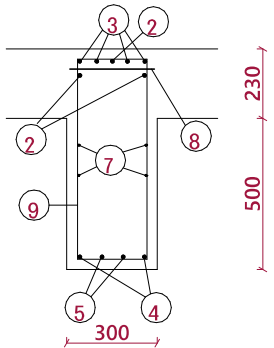
REZ B-B'1:25
