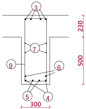
REZ A-A'1:25
