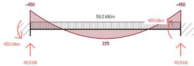
Obrázok D.2.3.2.3. – Momenty a reakcie na priznanom prievlaku nad 1.NP (výpočet cez statický model STRAIN)
