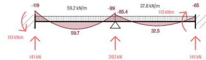
Obrázok D.2.3.3.9 – Momenty a reakcie na priznanom prievlaku nad 1.NP (výpočet cez statický model STRAIN)
