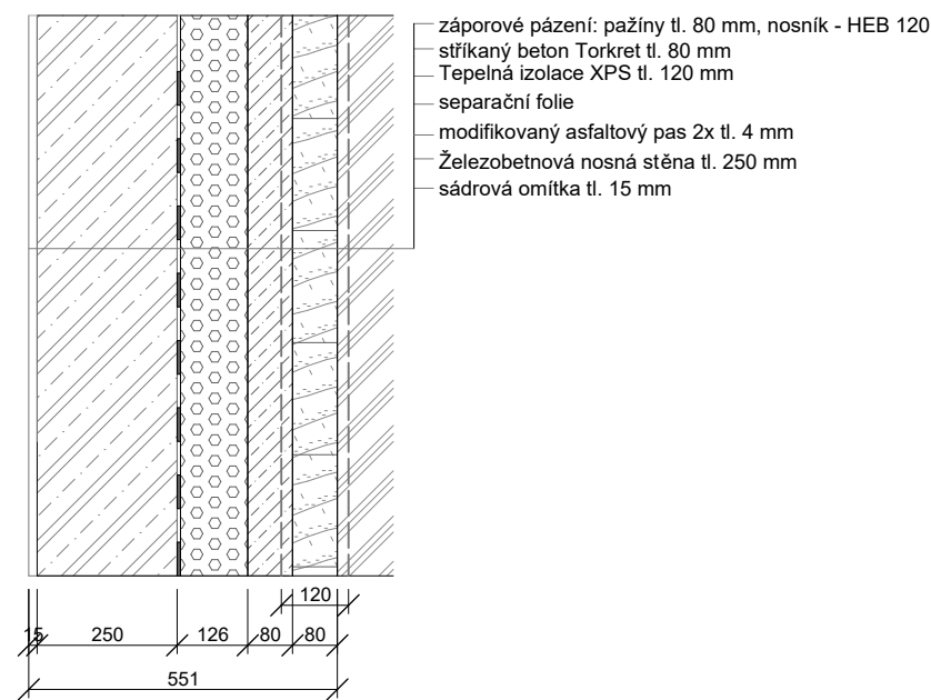
S2 Obvodová stěna v 1PP objektu
