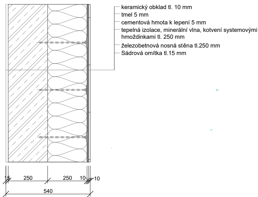
S2 Obvodová stěna v 1NP a 2NP objektu
