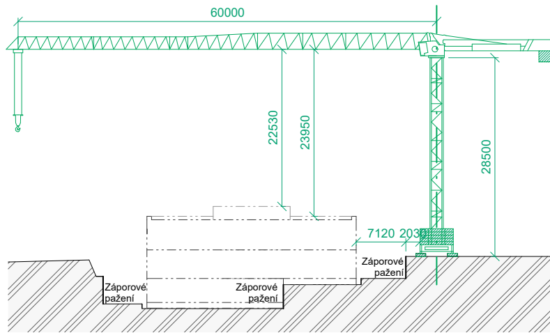
LM 1 LEIBHERR 270 EC - B 12
