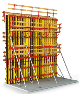
Stěnové bednění PERI VARIO GT 24
