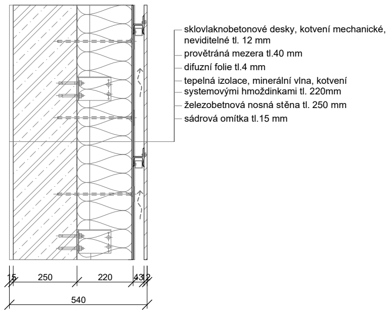
S1 Obvodová stěna v 1NP a 2NP objektu
