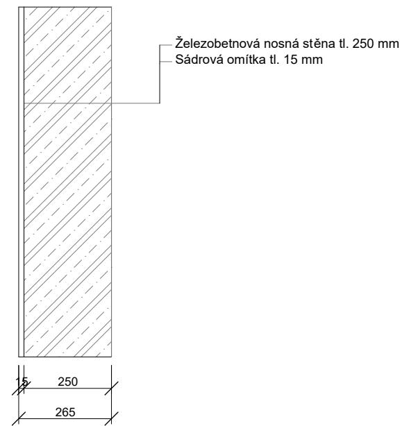
S2 Vnitřní nosná stěna
