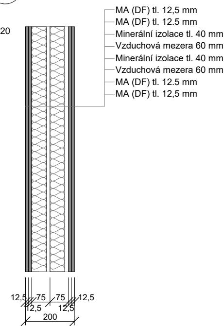
S2 Vnitřní SDK příčka Knauf RED Pb
