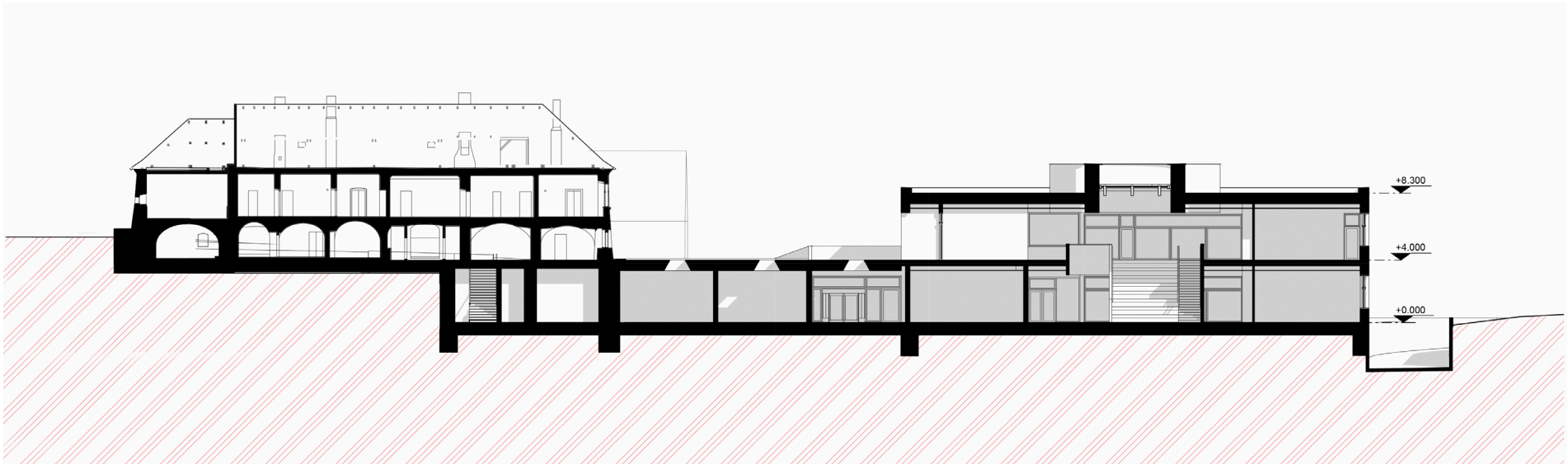
ŘEZ PŘÍČNÝ 1:400
