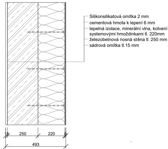
S3 Obvodová stěna ve 1NP, fasádní "niky"
