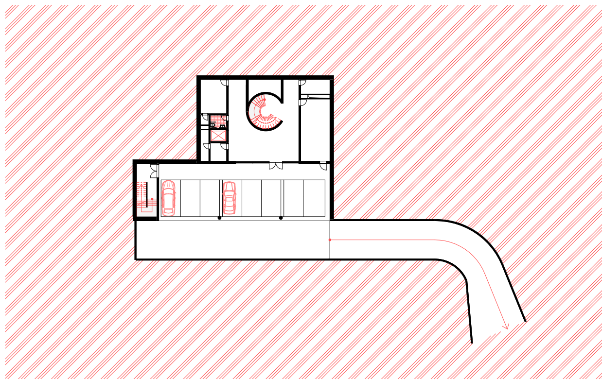
PŮDORYS 1PP 1:500
