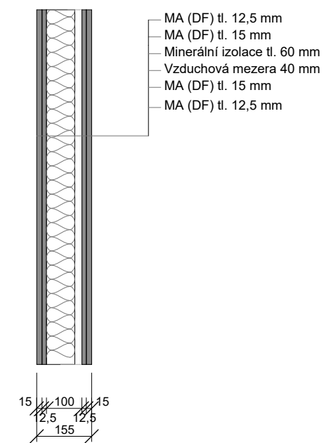
S2 Vnitřní SDK příčka Knauf RED Pb
