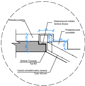
D1 Nonsý prvek pro izolaci proti kročejovému zvuku
