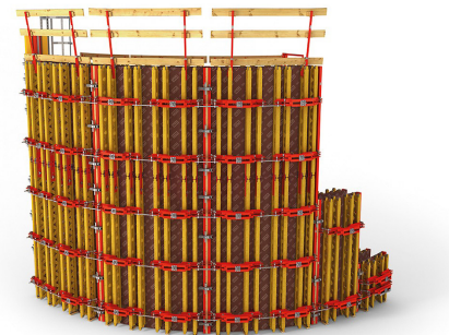
Kruhové stěnové bednění PERI RUNDFLEX
