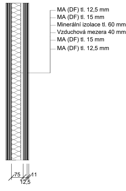
S2 Vnitřní SDK příčka, Knauf Aquapanel
