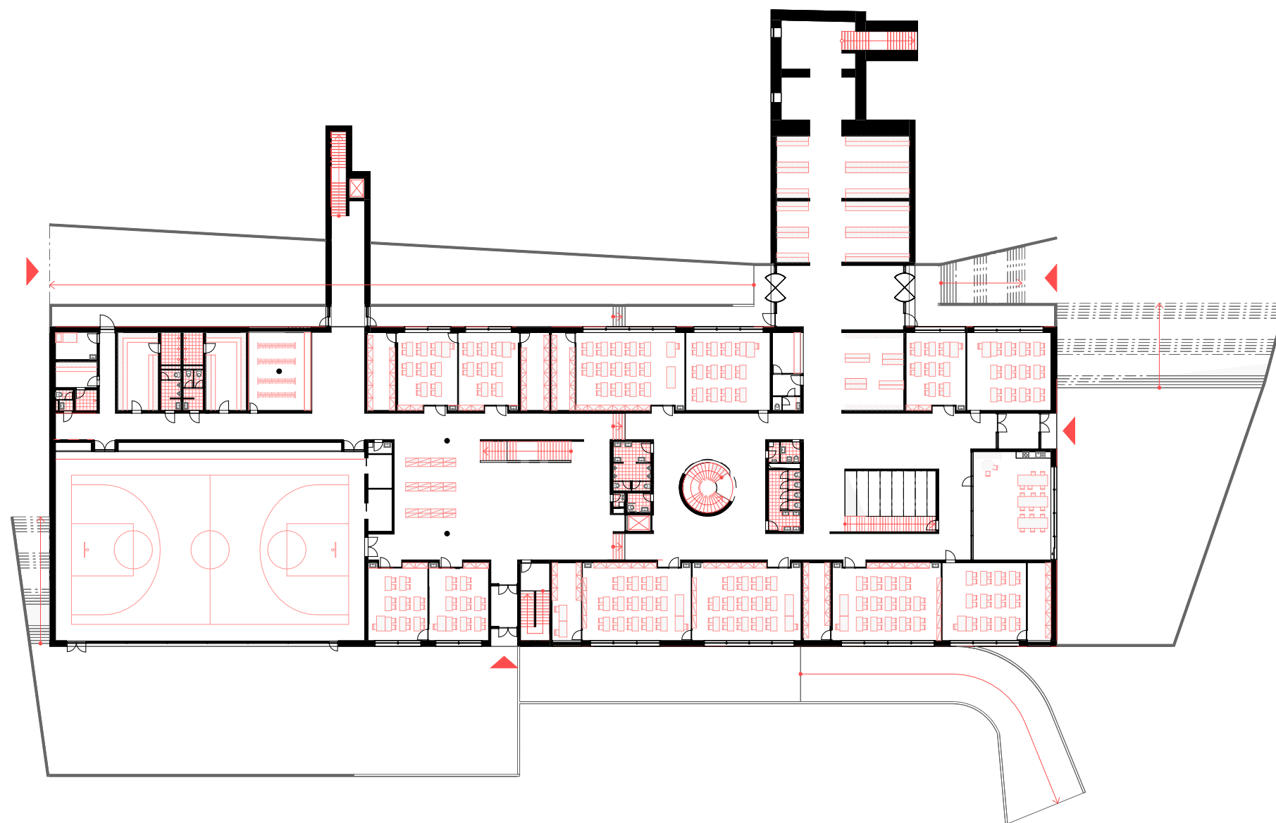
PŮDORYS 1NP 1:500
