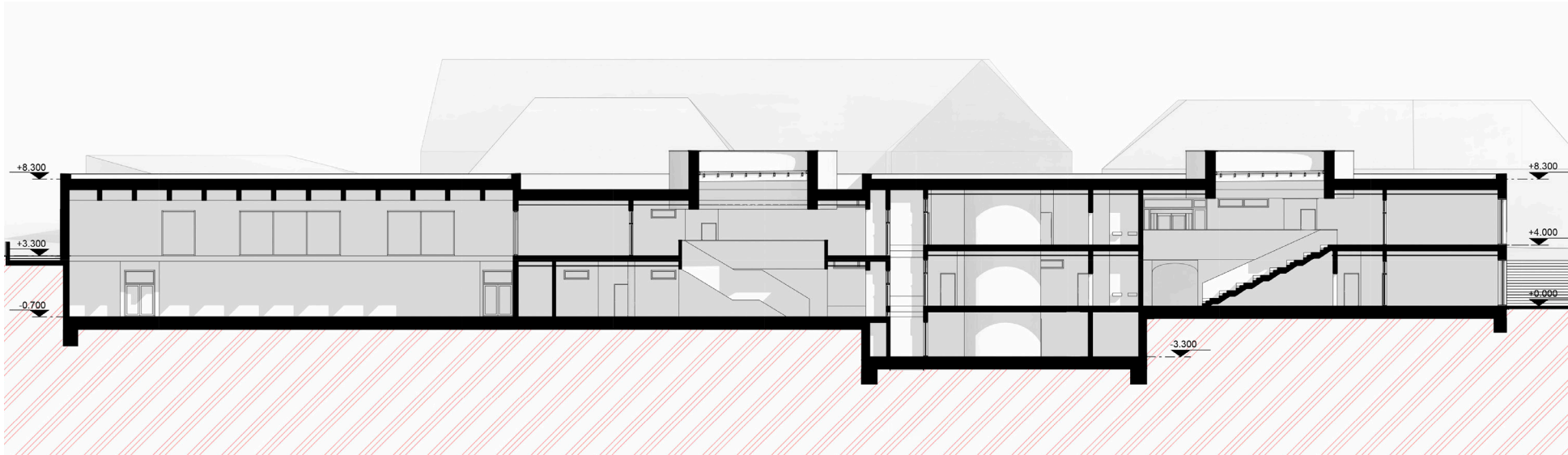
ŘEZ PODELNÝ 1:400
