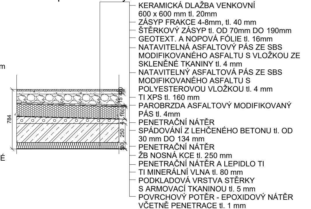
Podlaha pochozí terasy s dalždicemi
