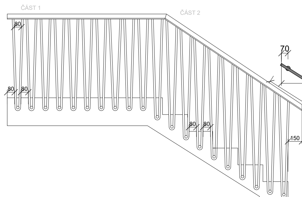
ZÁBRADLÍ Z5 M 1:25
