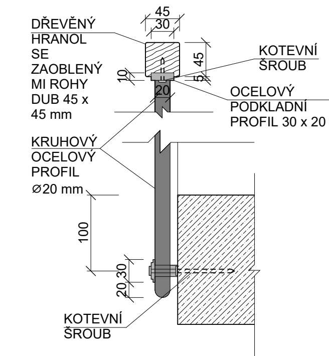
DETAIL KOTVENÉ ZÁBRADLÍ Z6 M 1:5
