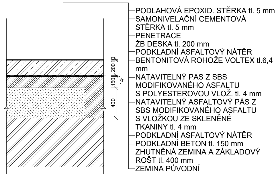
Podlaha spodní stavba
