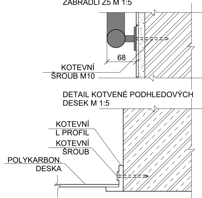
DETAIL KOTVENÉ ZÁBRADLÍ Z5 M 1:5
