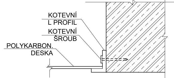
DETAIL KOTVENÉ PODHLEDOVÝCH DESEK M 1:5
