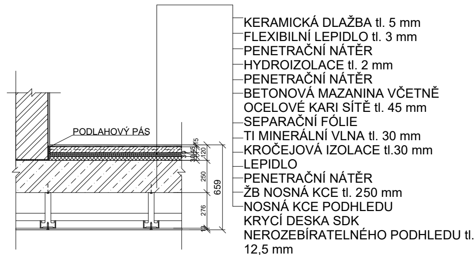
Podlaha koupelen/toalet bytu + podhledy
