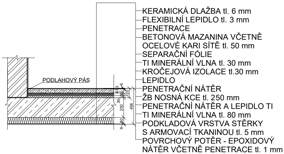
Podlaha společné chodby
