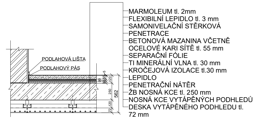
Podlaha obytné prostory bytu + vytápěné podhledy
