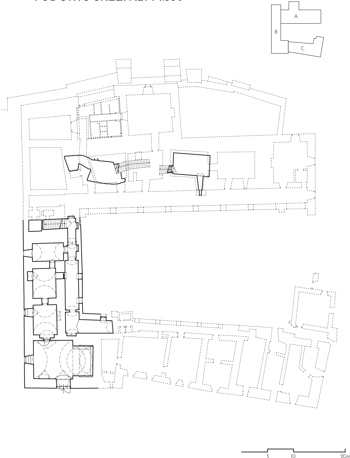
PŮDORYS SKLEPA_M 1:350
