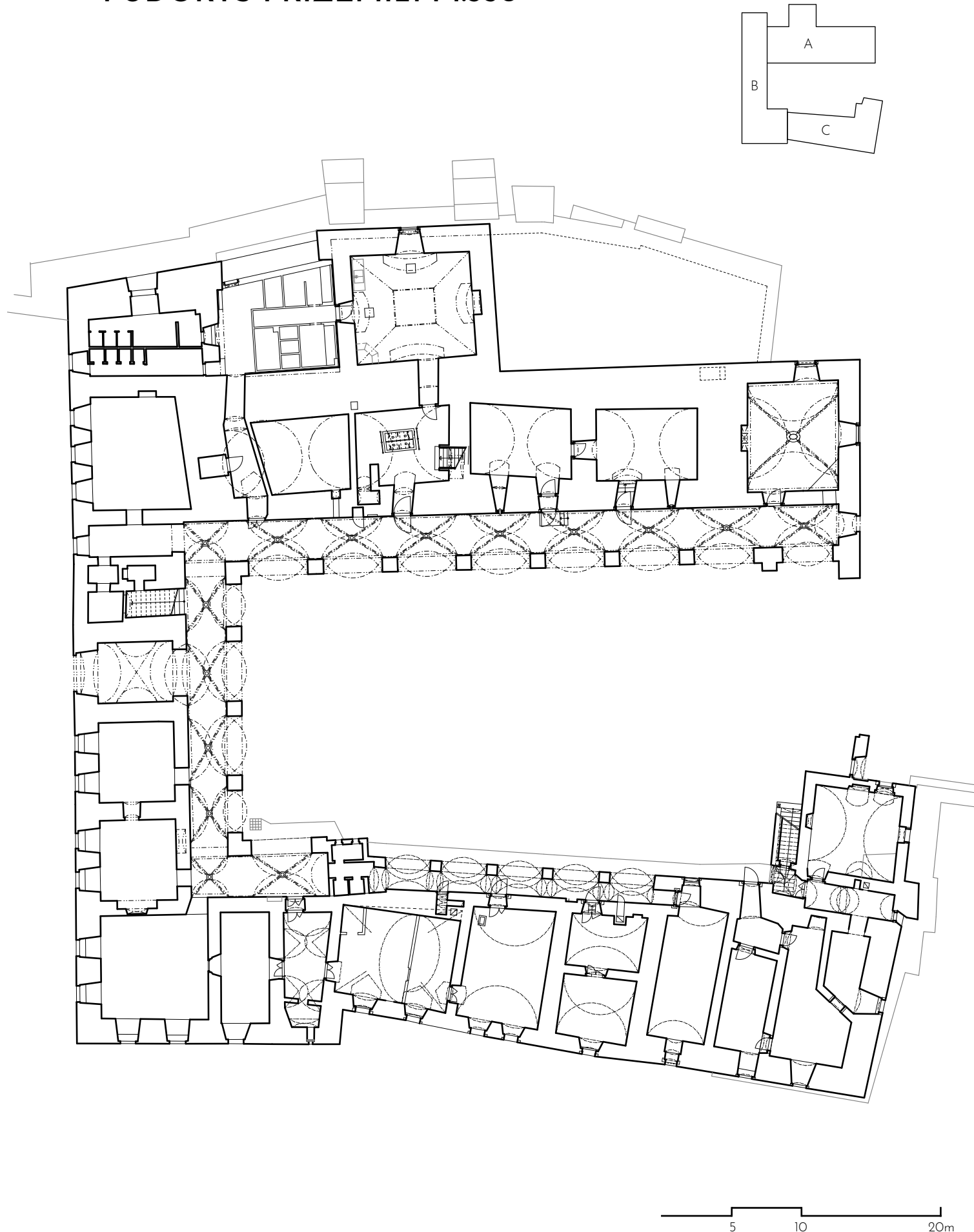
PŮDORYS PŘÍZEMÍ_M 1:350
