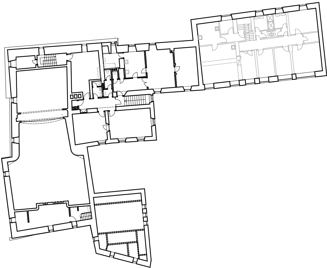
PŮDORYS 1. PATRA_M 1:350
