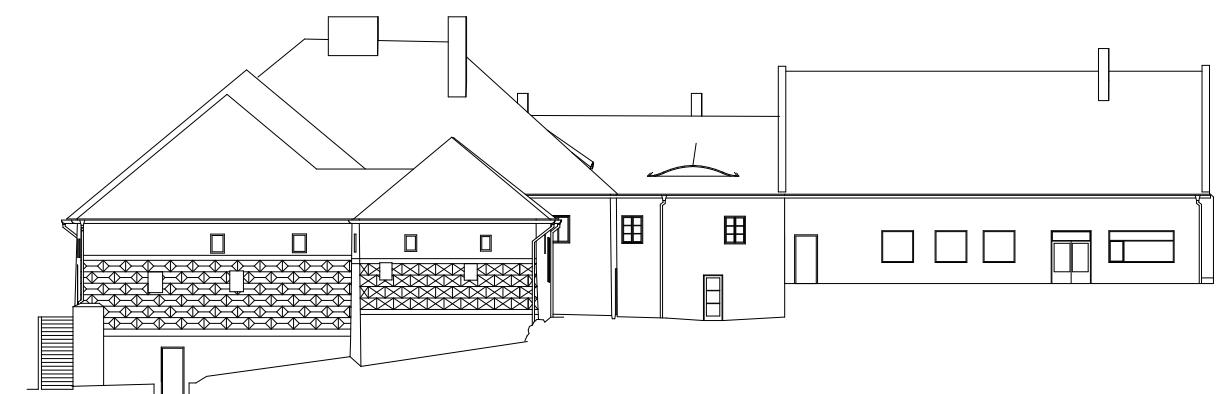
POHLED VÝCHODNÍ_M 1:350
