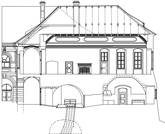
ŘEZ A2_M 1:350
