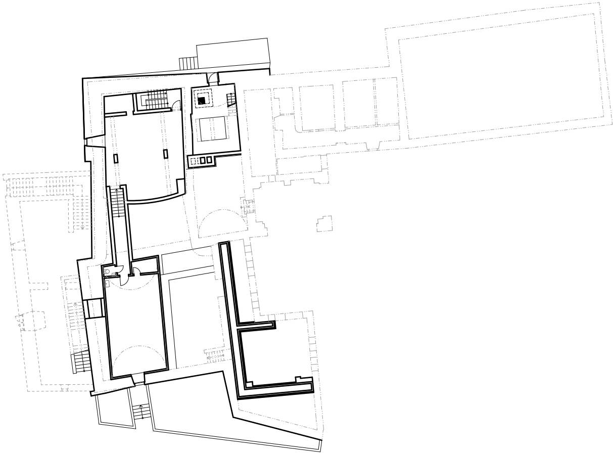
PŮDORYS SKLEPA_M 1:350
