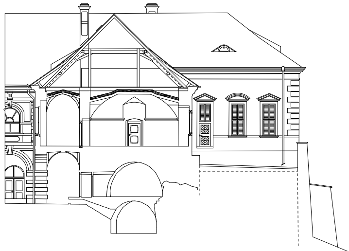
JIŽNÍ KŘÍDLO C ŘEZ C1_M 1:350
