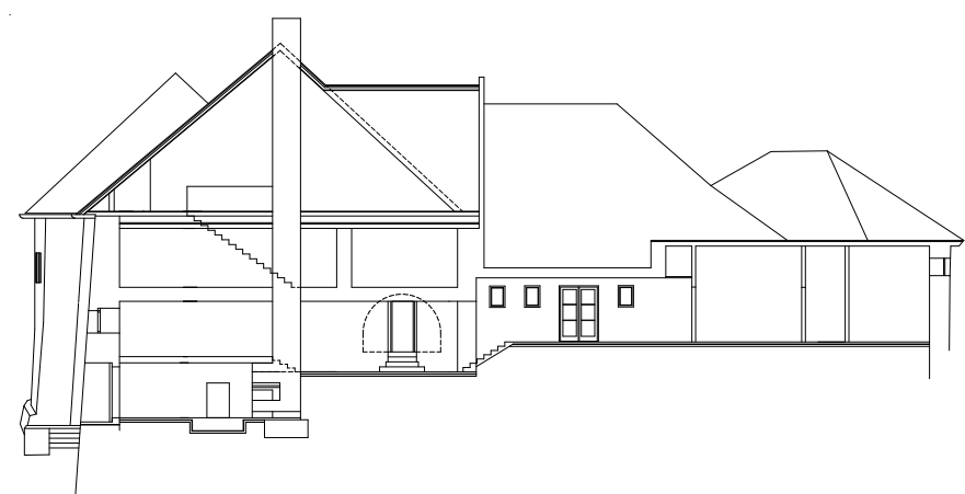
ŘEZ A2_M 1:350
