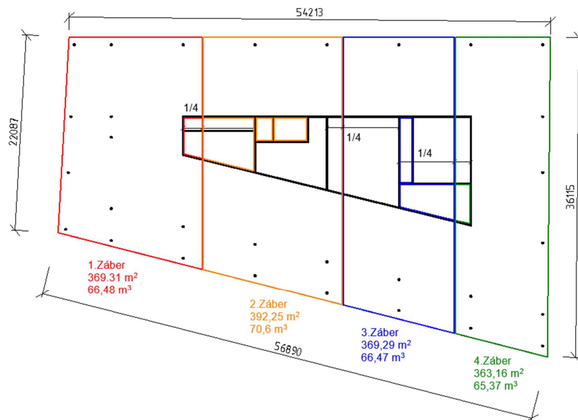
Obr. 3.2.1 Schéma betonárskych záberov pre vodorovné nosné konštrukcie
