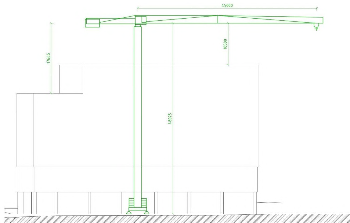
Obr. 4.2.2 Poloha a rozsah žeriavu na stavenisku v pohľade
