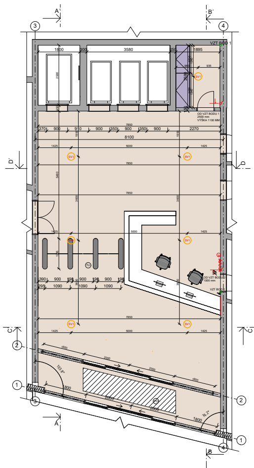
PŮDORYS 1NP
