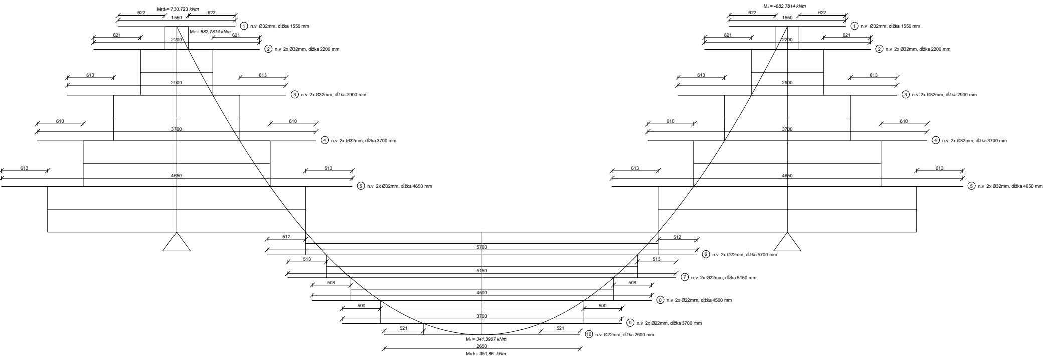
GRAFICKÝ VÝPOČET DĹŽOK PRUTOV 1:25
