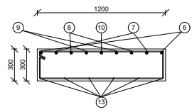
REZ sA - sA' 1:25
