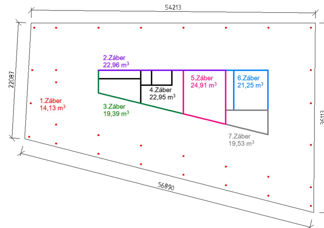
Obr. 3.2.2 Schéma betonárskych záberov pre zvislé nosné konštrukcie
