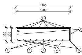
REZ sA - sA' 1:25
