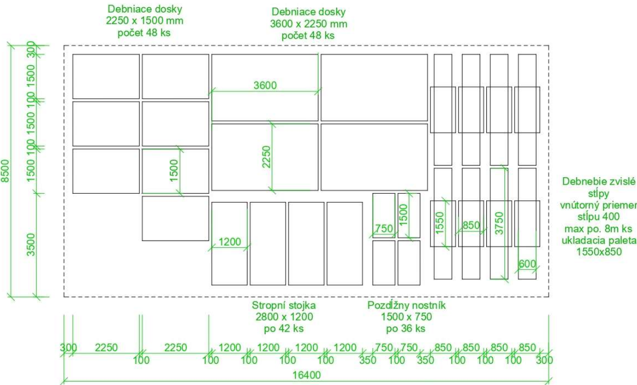
Obr. 3.3.4 Schéma skladovacích plôch debnenia
