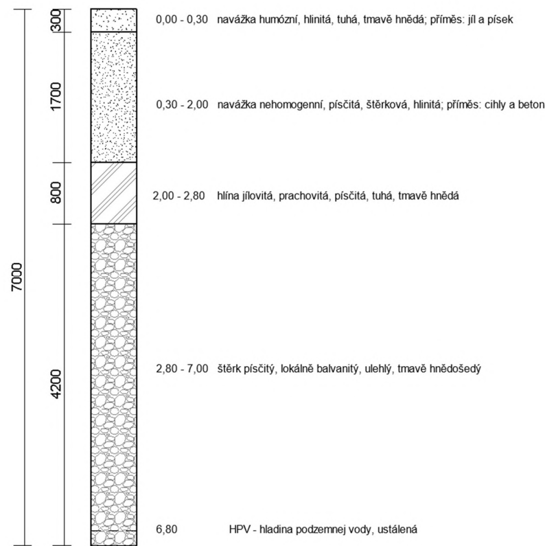
Obr. 2.1.1 Schéma geologického zloženia pôdy na základe informácií a zemného vrtu
