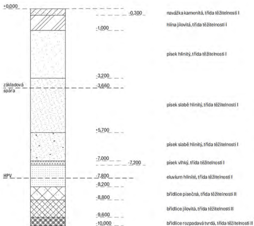
Profil vrtu 634318
