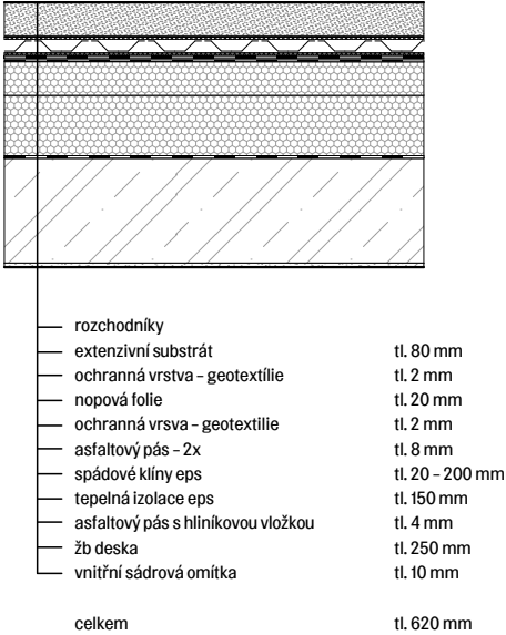
P10 VEGETAČNÍ STŘECHA
