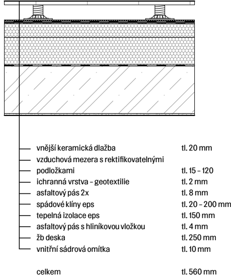
P09 POCHOZÍ TERASA
