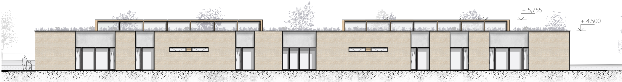
POHLED JIŽNÍ (1) M 1:250
