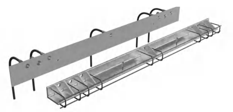
Obrázek 1 – systém ocelové konzoly
