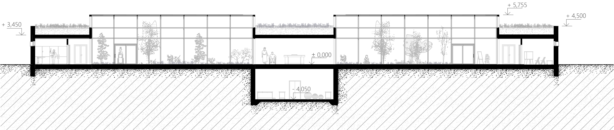
ŘEZ B-B'
