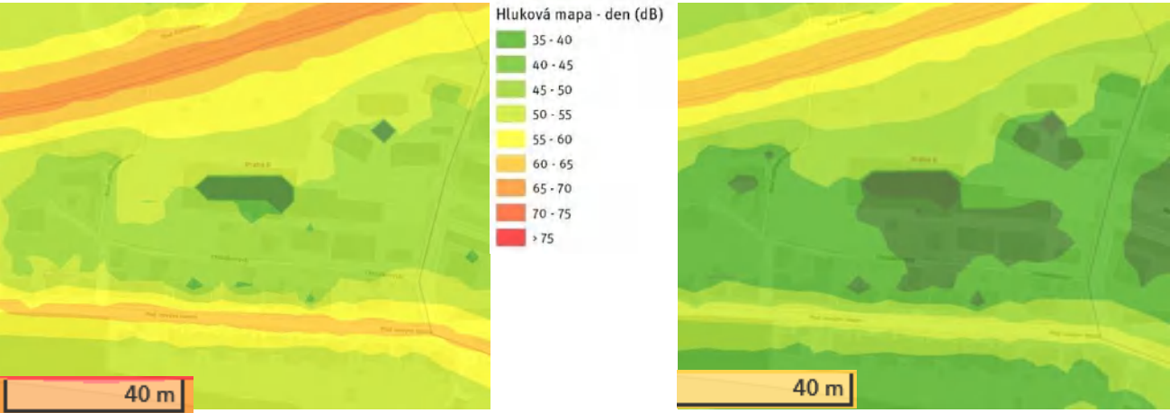
Obrázek 4 - Hladina hluku - noc (22:00 - 6:00)
