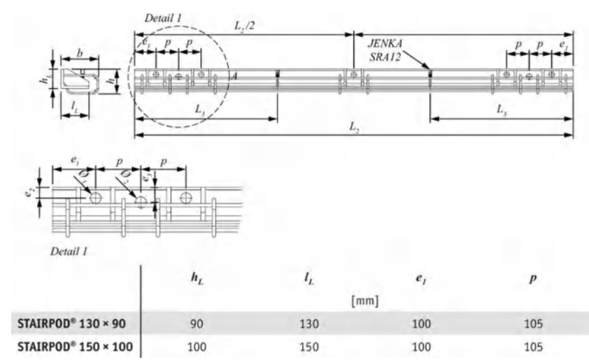
Obrázek 1 – systém ocelové konzoly
