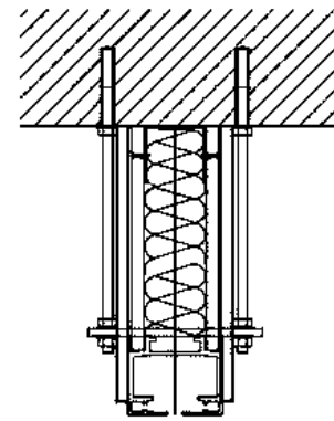
Obrázek 1 - Detail čtyřplášťové přepážky
