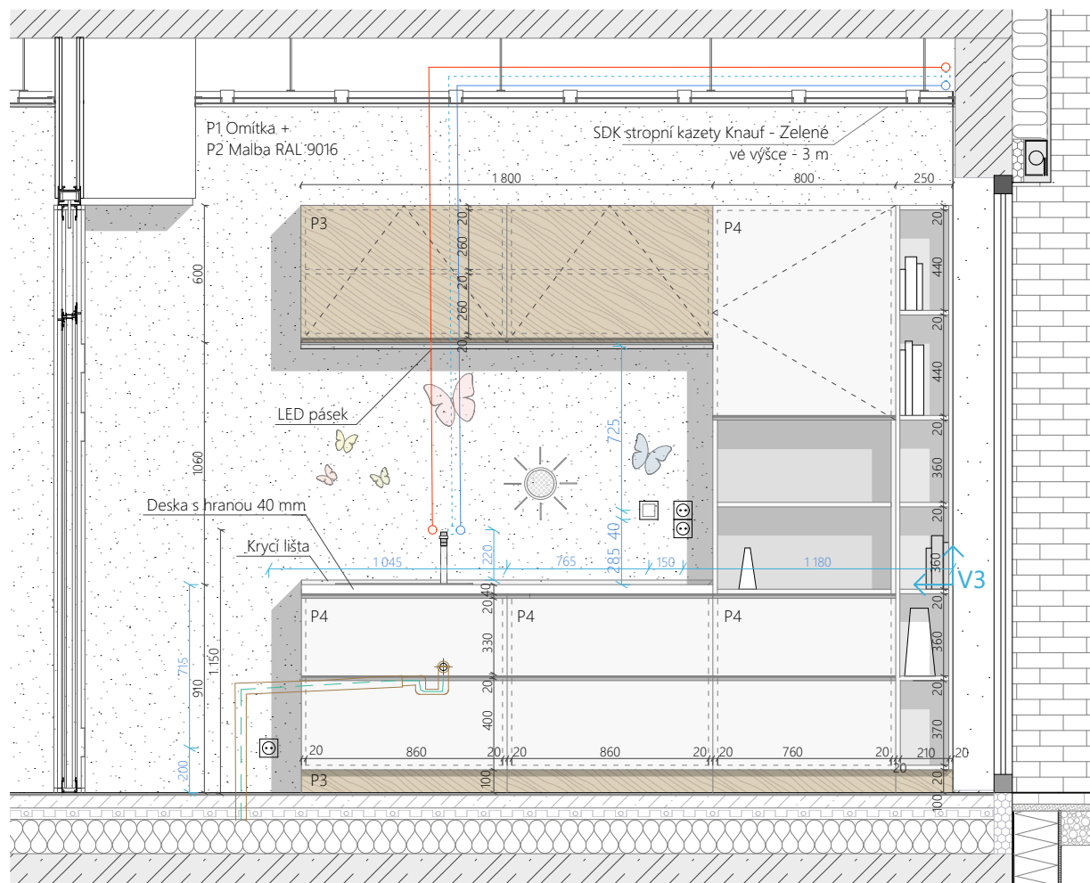
POHLED 3
