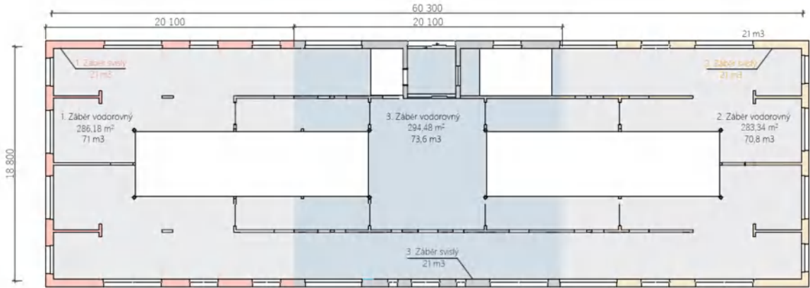
Obrázek 1 - Schéma betonářských záběrů
