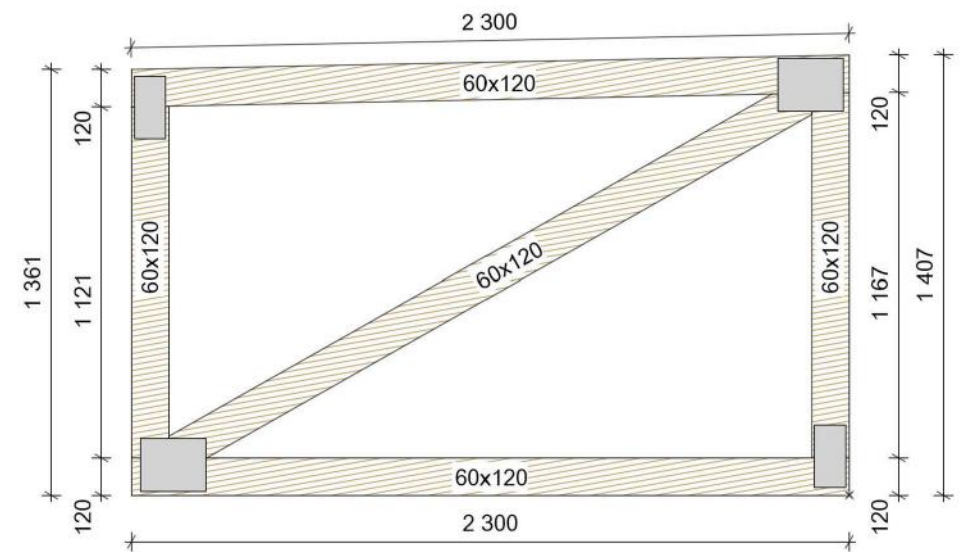
Schéma vazníku V1
