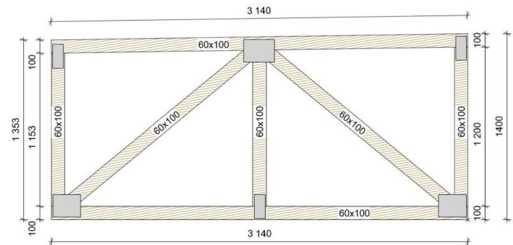
Schéma vazníku V3
