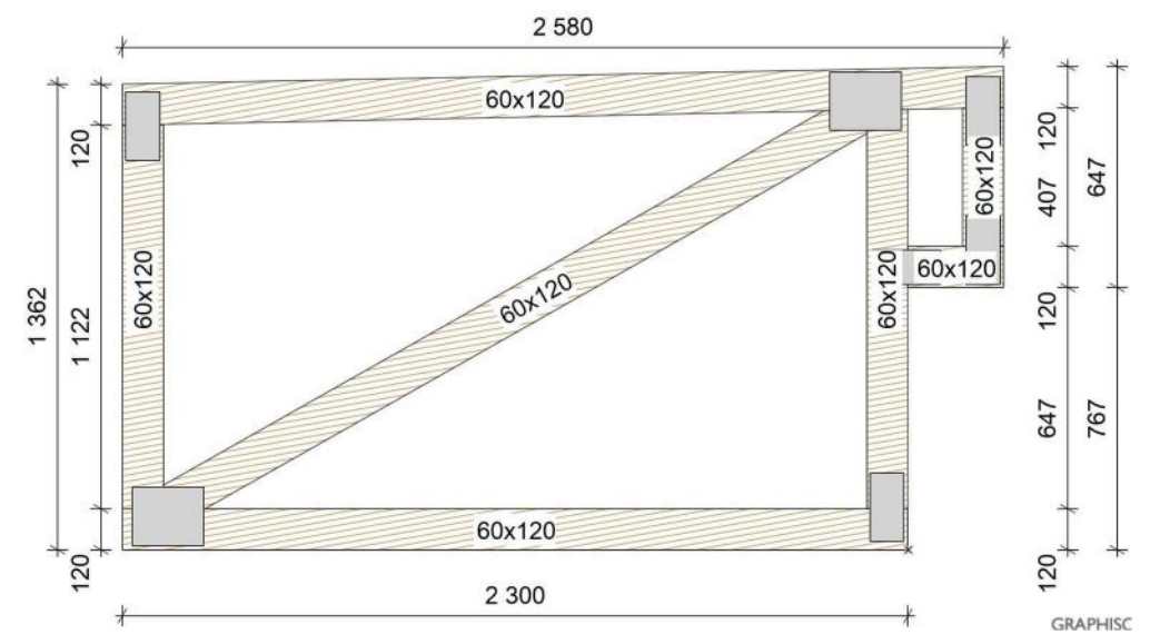
Schéma vazníku V2
