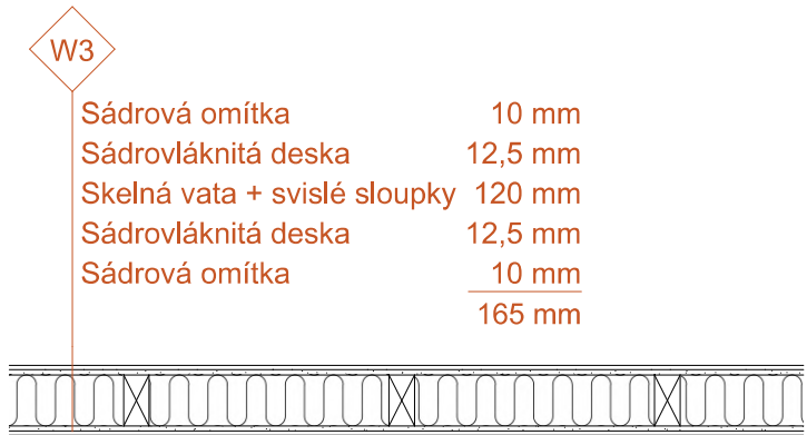
VNITŘNÍ NENOSNÁ STĚNA
