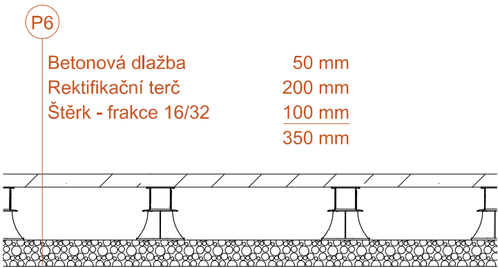
PODLAHA VENKOVNÍ TERASY
