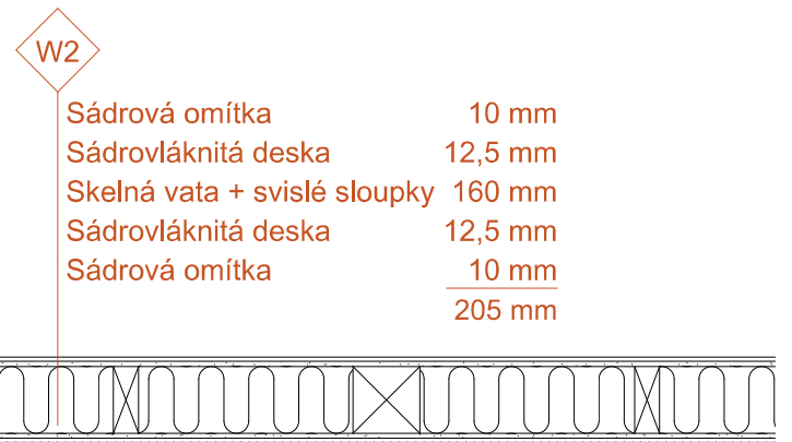
VNITŘNÍ NOSNÁ STĚNA
