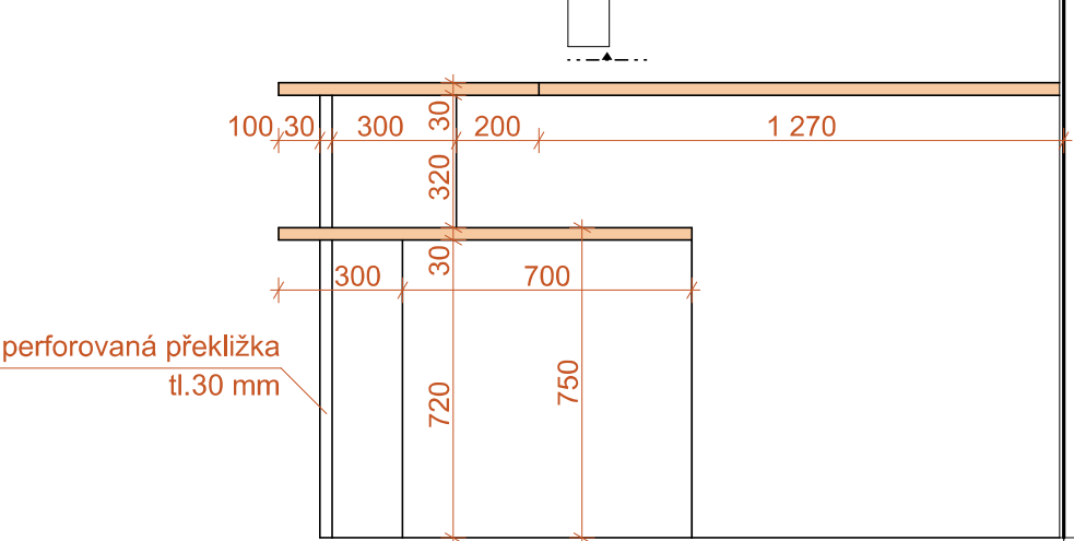
POHLED JIŽNÍ
