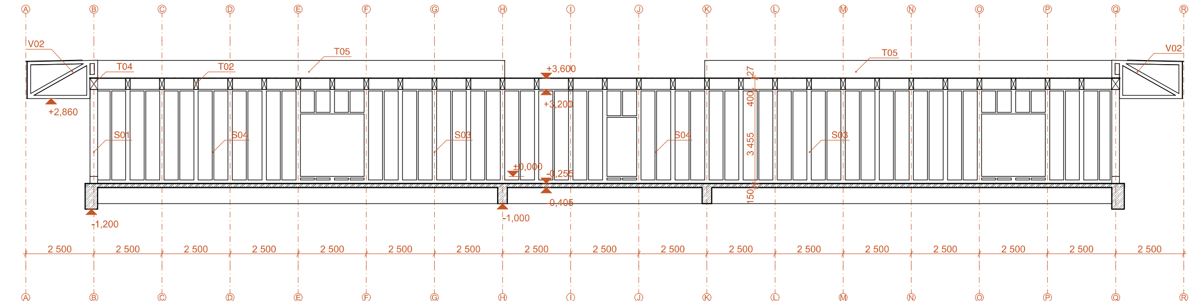
ŘEZ PODÉLNÝ B - B'
