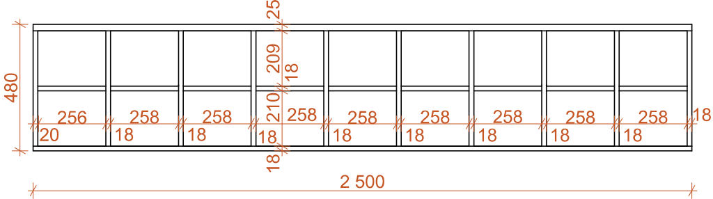
POHLED PŘEDNÍ NA LAVICI NA BOTY
