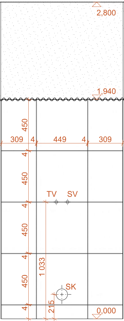
POHLED NA SEVERNÍ STĚNU
