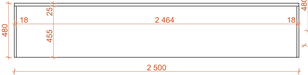
POHLED BOČNÍ
