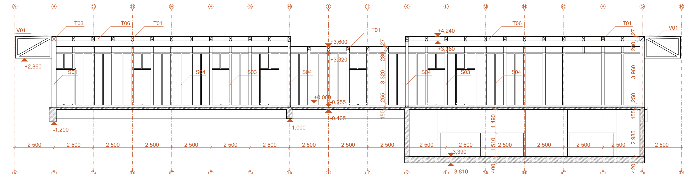
ŘEZ PODÉLNÝ C - C'
