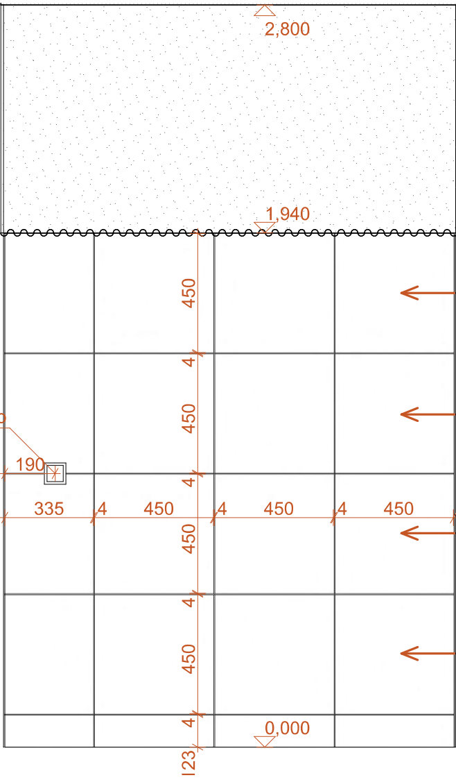
POHLED NA ZÁPADNÍ STĚNU
