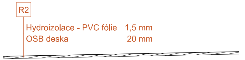
STŘECHA TERASY
