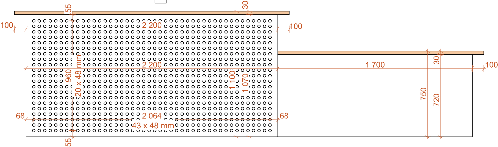
POHLED SEVERNÍ
