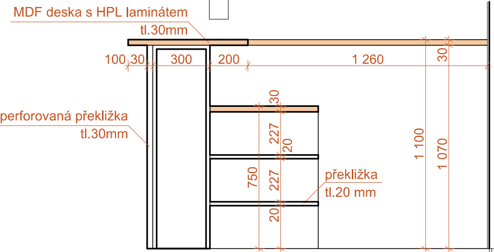
ŘEZ
