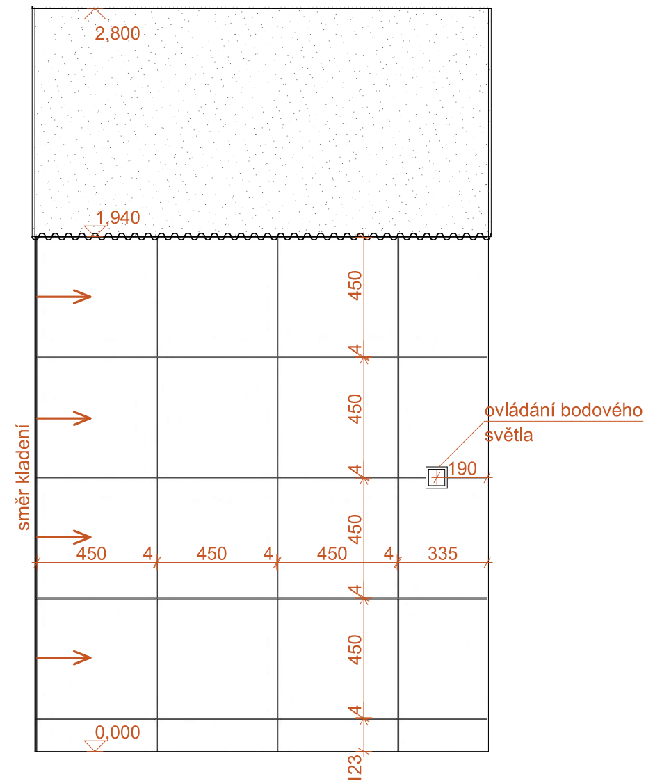
POHLED NA ZÁPADNÍ STĚNU
