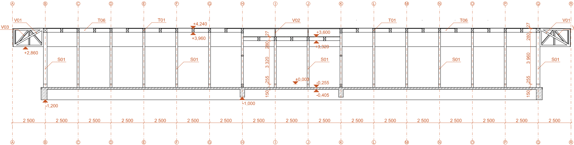
ŘEZ PODÉLNÝ A - A'
