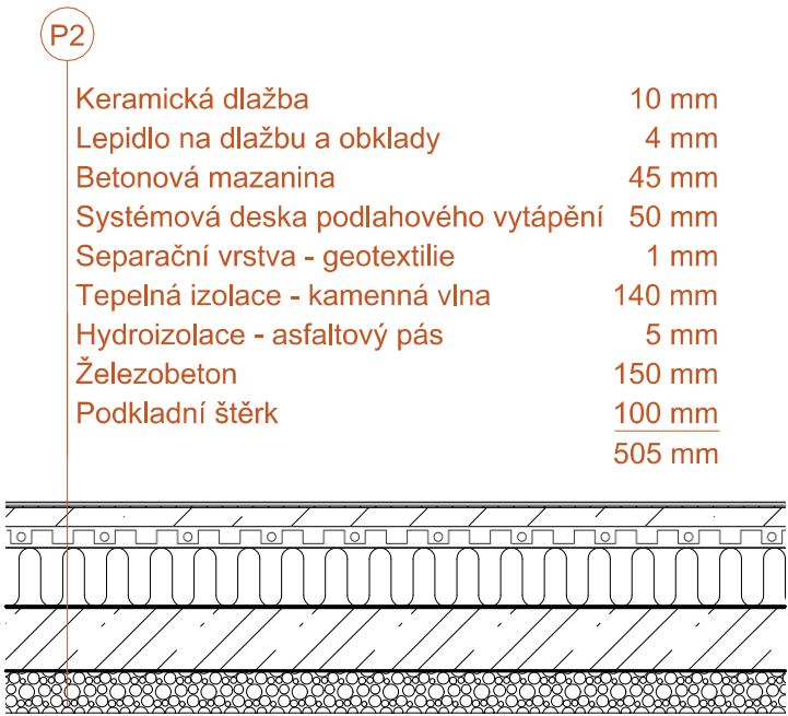
PODLAHA V HYGIENICKÝCH ZÁZEMÍCH
