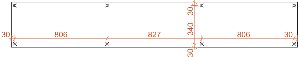
PŮDORYS
