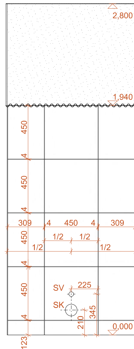
POHLED NA JIŽNÍ STĚNU
