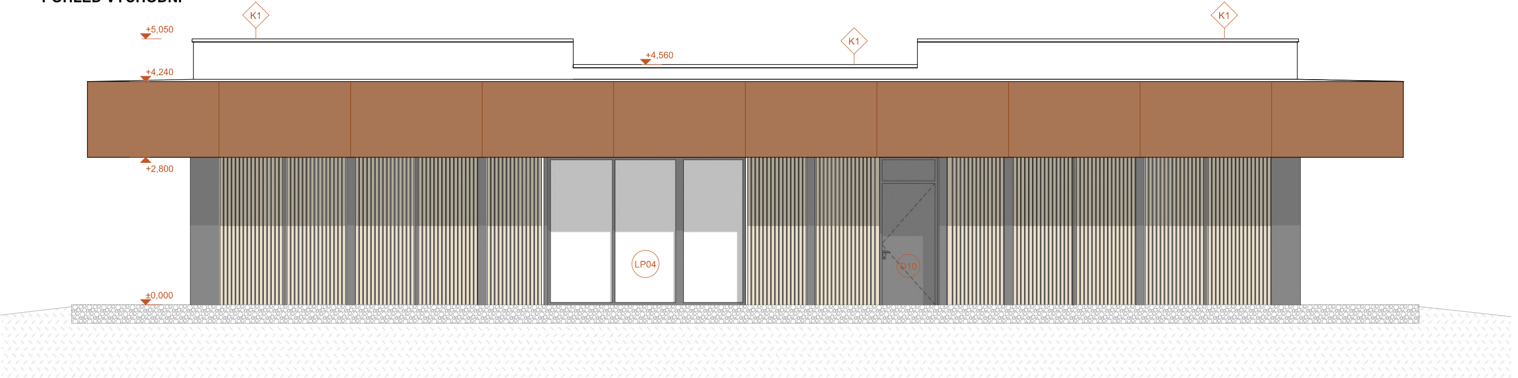
POHLED VÝCHODNÍ
