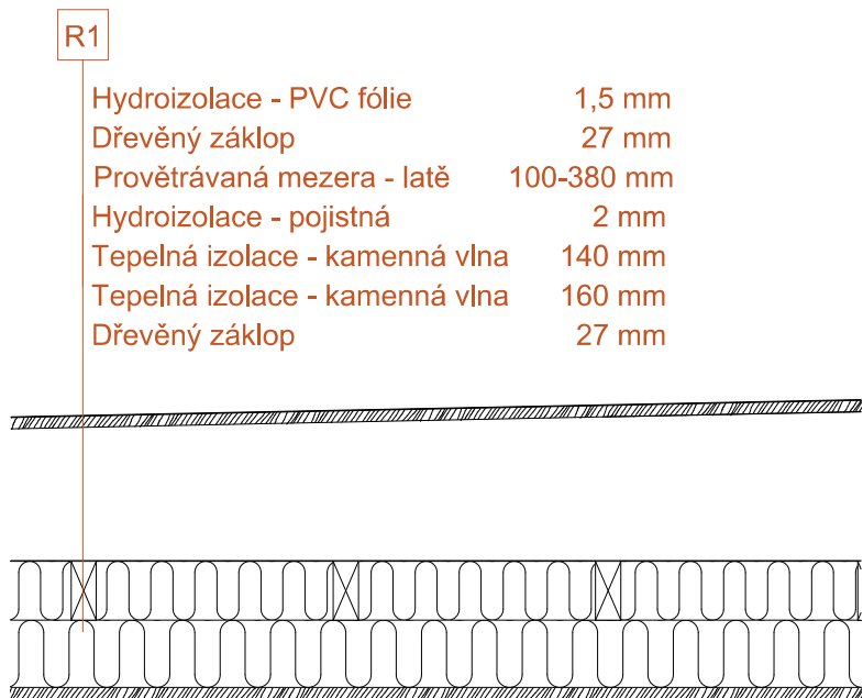
STŘEŠNÍ PLÁŠŤ
