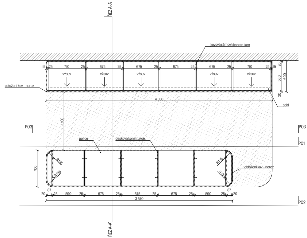
B BAR - PŮDORYS 2 1:25
