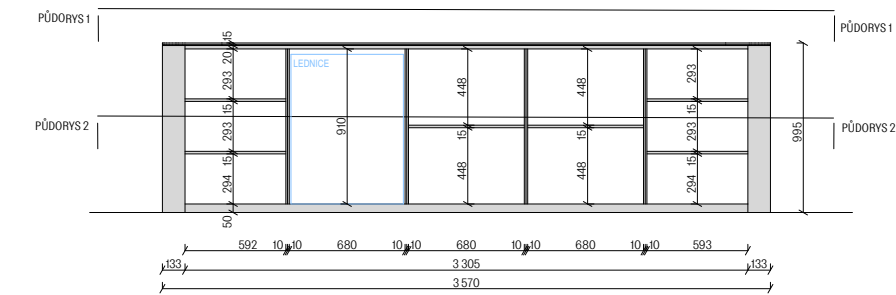
E BAR - POHLED P03 1:25
