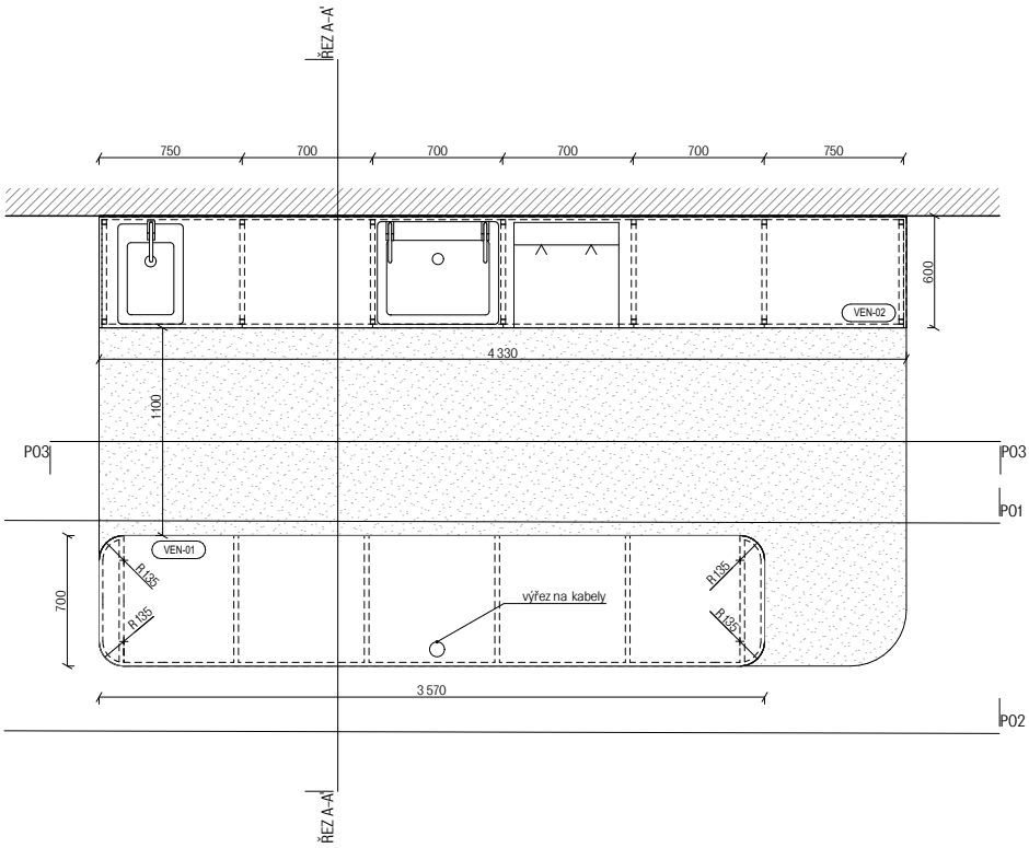
A BAR - PŮDORYS 1 1:25
