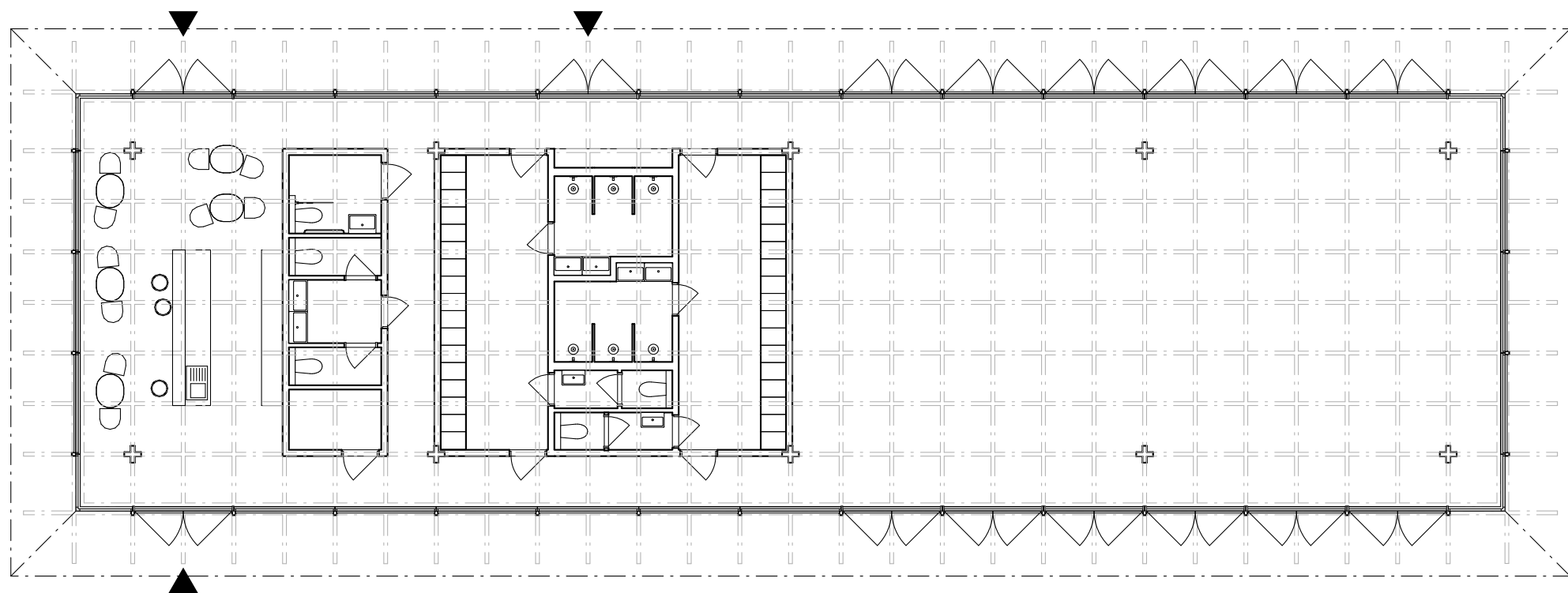
půdorys 1.NP
