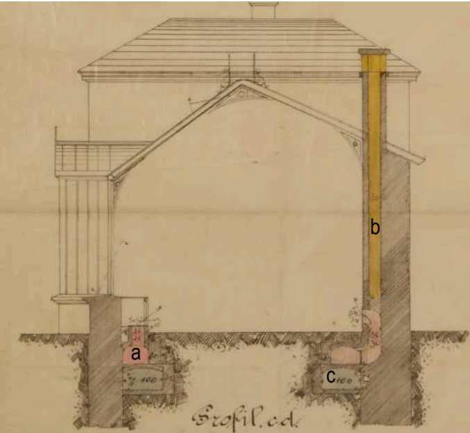
Libochovice detail řezu, legenda: a - teplovodný kanálek, b - větrací kanálek (zakončen komínem), c - cirkulační kanálek
