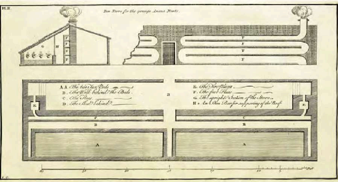
6 „Tan Stove for the younge Anana[s] Plants“, aus: Philip Miller: The Gardners Dictionary, 8. Aufl., London 1768, Pl. II.
