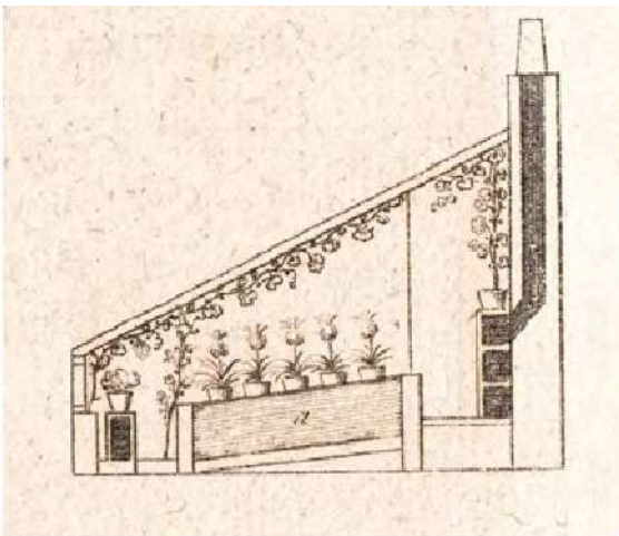
Abb. 4 Kew Gardens, London, Ananashaus, Querschnitt, aus: Gottlob Friedrich Seidel, Der exotische Gärtner, Dresden 1817, Tafel I (Ausschnitt).
