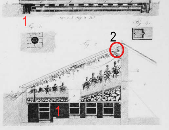
Ananasový skleník 1- Topný systém pro výhřev kořenů ananasů 2-vnitřní kladka pro zavěšení popínavé rostliny
