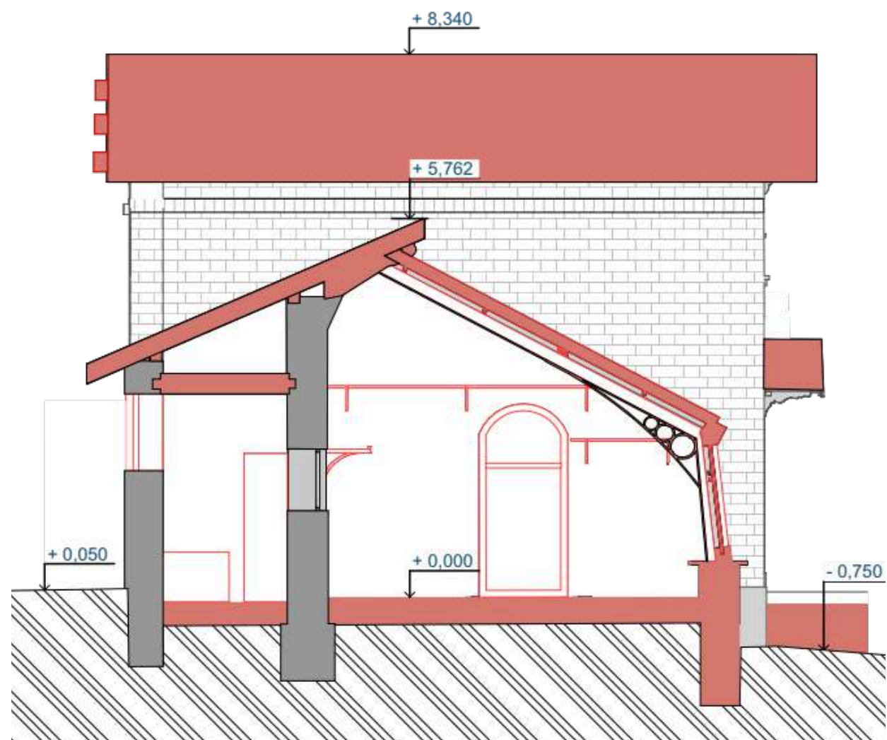
ŘEZ B-B'
