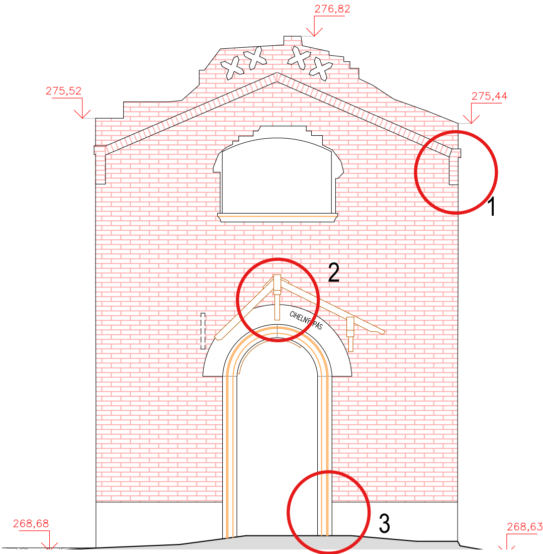
Výkres zaměření jižní pohled na oblужnou budovu zdroj: zaměření 2022, autor: Němec, zaměření poskytnuto kastelánem Mgr. Vladimírem Treglem
