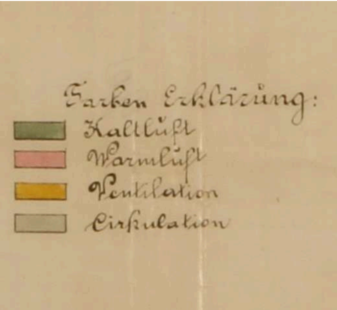
Libochovice - detail a překlad legendy KALTLUFT - studený vzduch, WARMLUFT - teplý vzduch, VENTILATION - větrání, CIRKULATION- cirkulace, oběh
