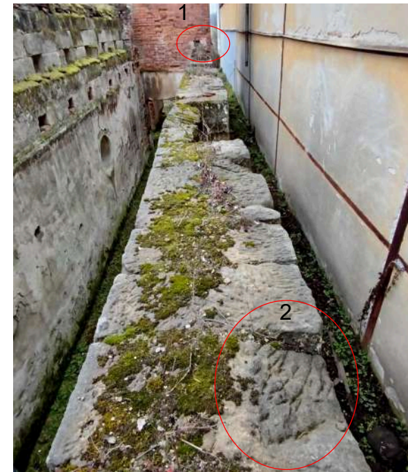
1- Pelíšky pro pozednici, 2- pelíšky v kameni pro krokve
