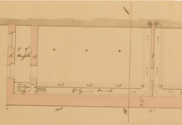
Liběchovice plán půdorysu- Detail směru prodění vzduchu
