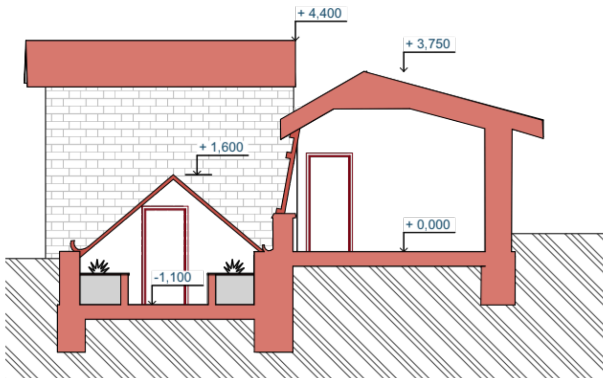
ŘEZ A-A'
