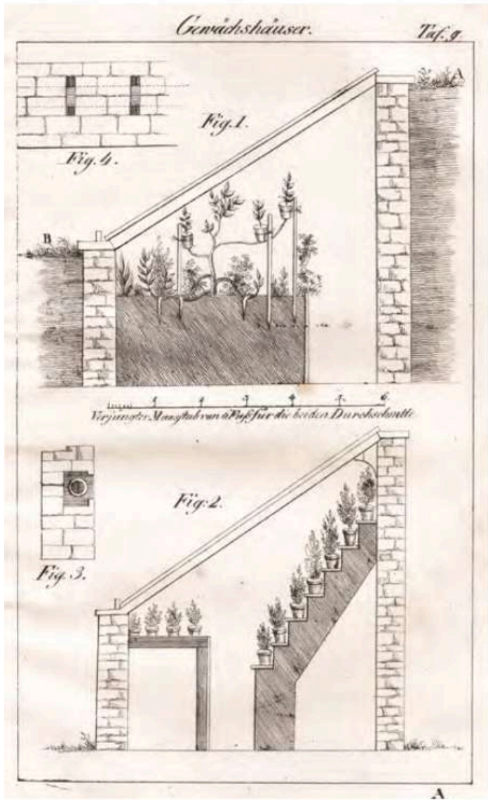
2 „Fig. 3“ und „Fig. 4“ verdeutlichen relevante bauliche Details der von Louis Noisette empfohlenen Rauchgasheizung für Wintergärten und Orangeriegebäude, aus: Louis Noisette: Vollständige Abhandlung von den Gärten und ihrer Anlegung, Stuttgart 1826, Tafel 9.
