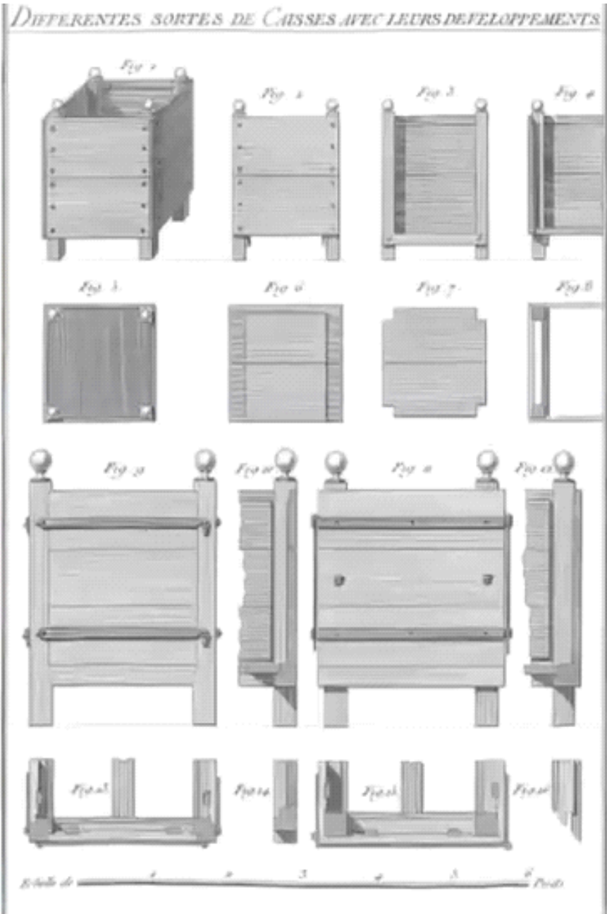
Rohy nádob pro květiny
