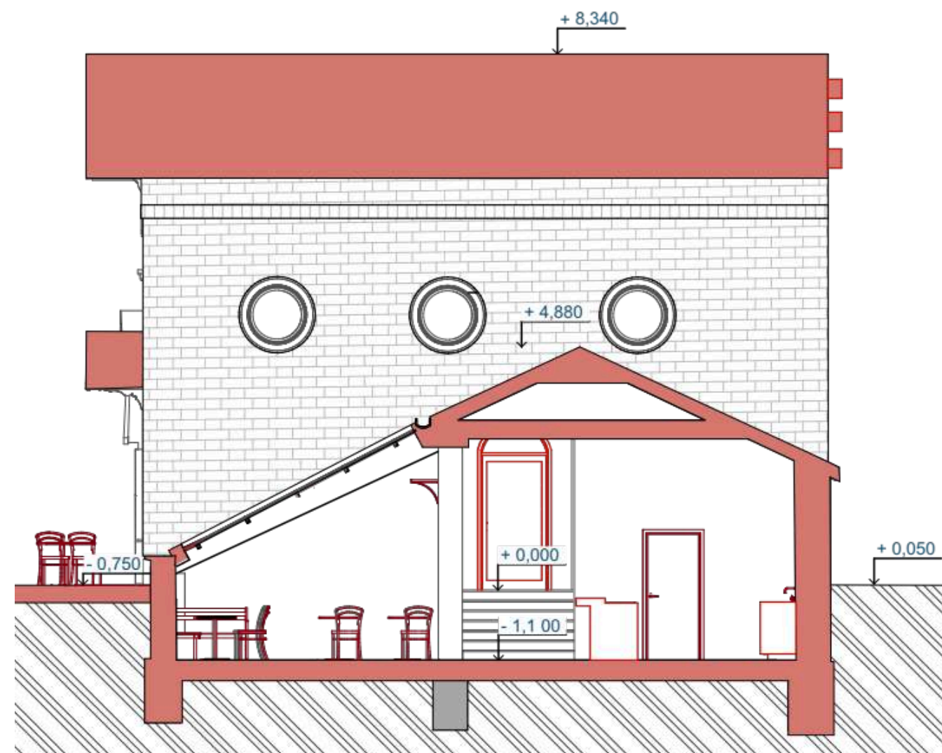
ŘEZ C-C'
