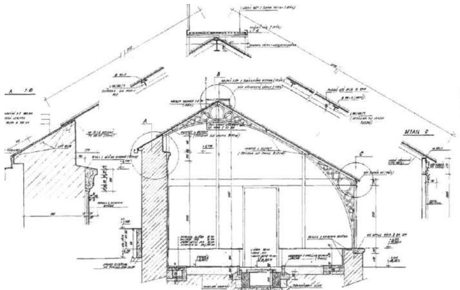
Rámový nosný systém velkého skleníku - inspirace Lány
