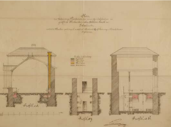
Libochovice výkres
