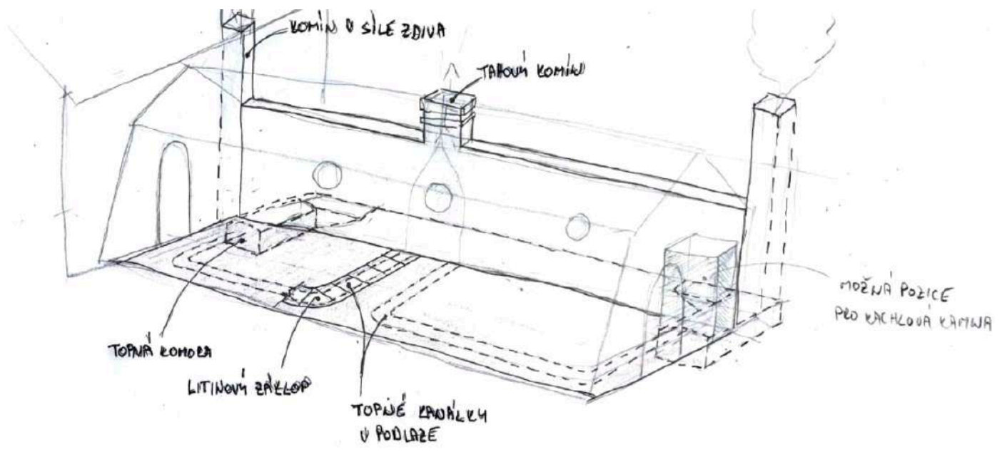
Schématická skica pravděpodobného topného zařízení ve velkém středovém skleníku Zdroj: Převzato od autorů Pokorný a Beránková
