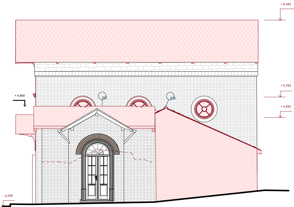
Pohled východní
