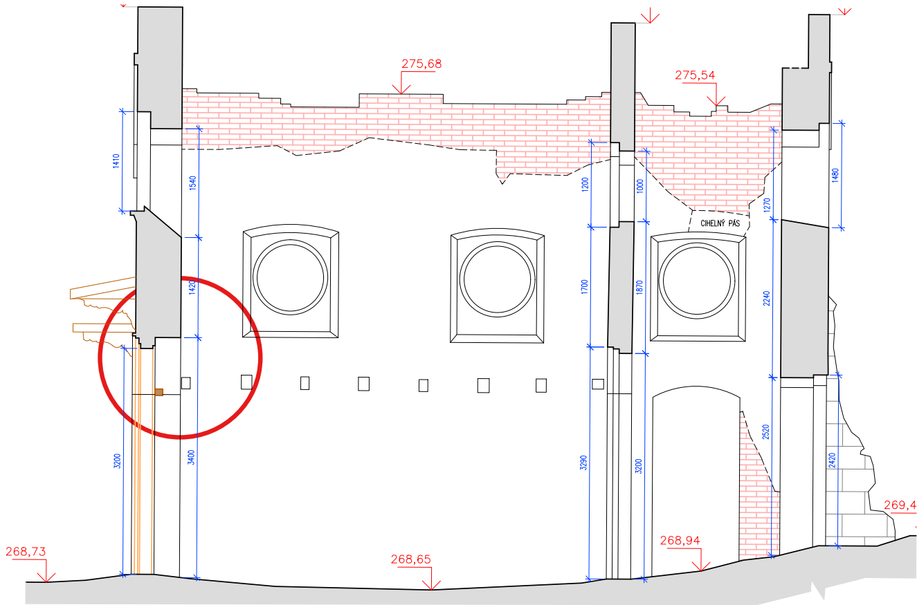
Výkres zaměření j- řez I-I', zaměření 2022, autor: Němec, zaměření poskytnuto kastelánem Mgr. Vladimírem Treglem
