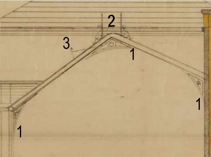
Libochovice výkres - detaily, 1-nosný systém, 2- lávka k obluhování stínění na vrchu skleníku, 3-naznační otevírání okna
