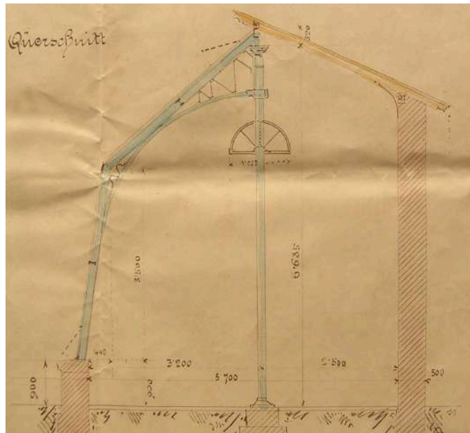
2- Konstrukce s sloupkem Buchlovice - plán
