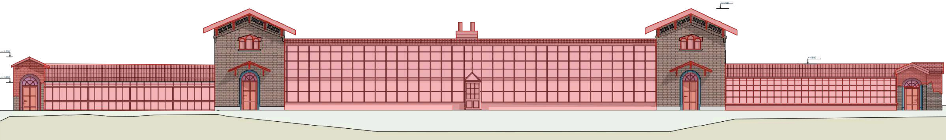
Jižní pohled 1:120
