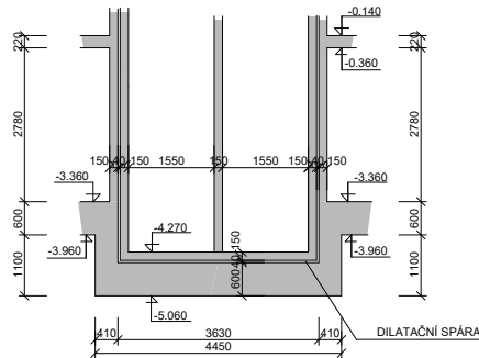
ŘEZ A-A' M 1:100
