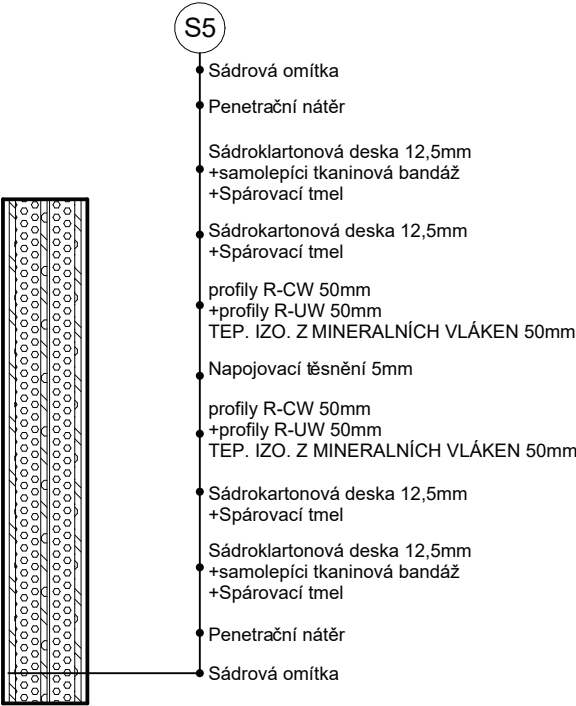
S5 VNITŘNÍ NENOSNÉ MONTOVANÉ PŘÍČKY tl. 170 mm
