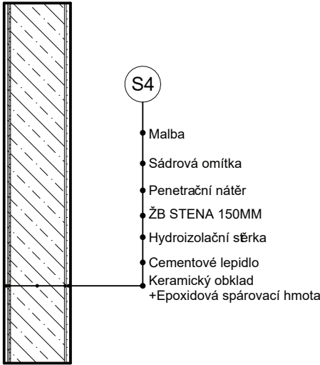
S4 VNITŘNÍ NOSNÉ STĚNY (MOKRÝ PROVOZ) tl. 185 mm
