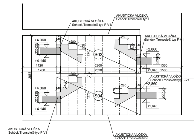
SCHÉMA SCHODIŠTE B 1:50
