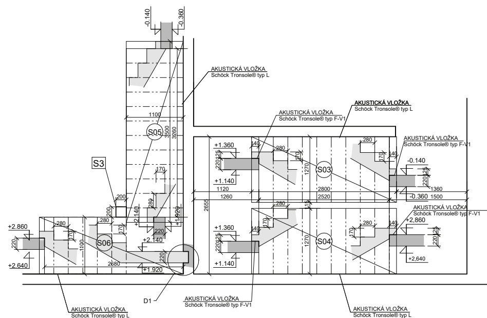
SCHÉMA SCHODIŠTE B 1:50
