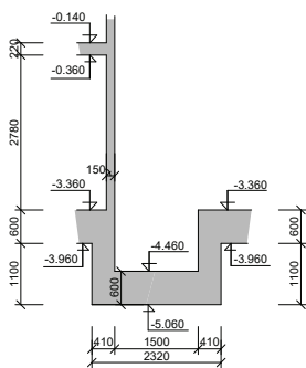
ŘEZ B-B' M 1:100
