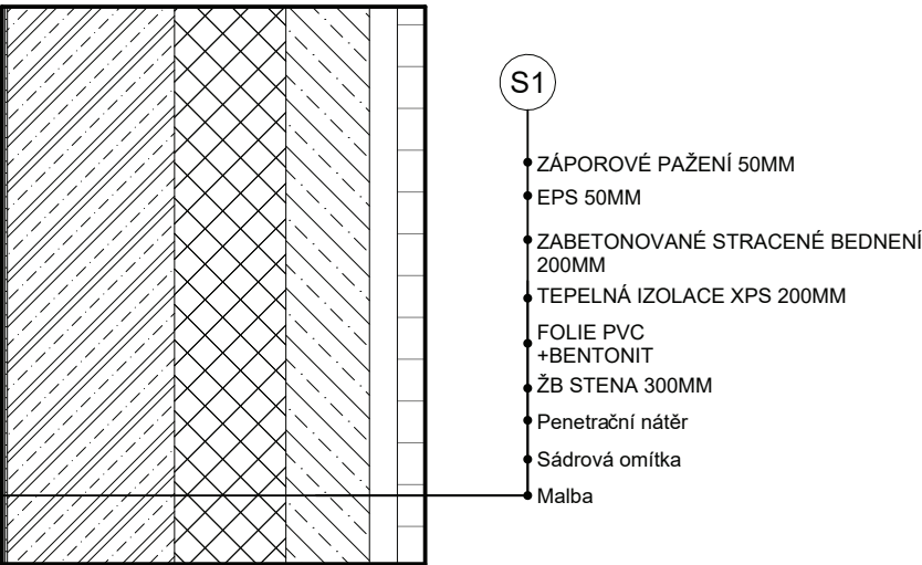
S1 OBVODOVÉ STĚNY SUTERÉN tl. 760 mm
