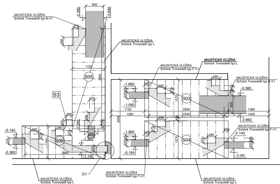
SCHÉMA SCHODIŠTE B 1:50
