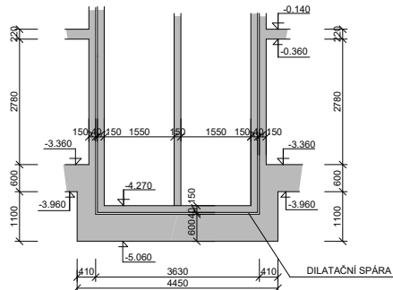
ŘEZ A-A' M 1:100
