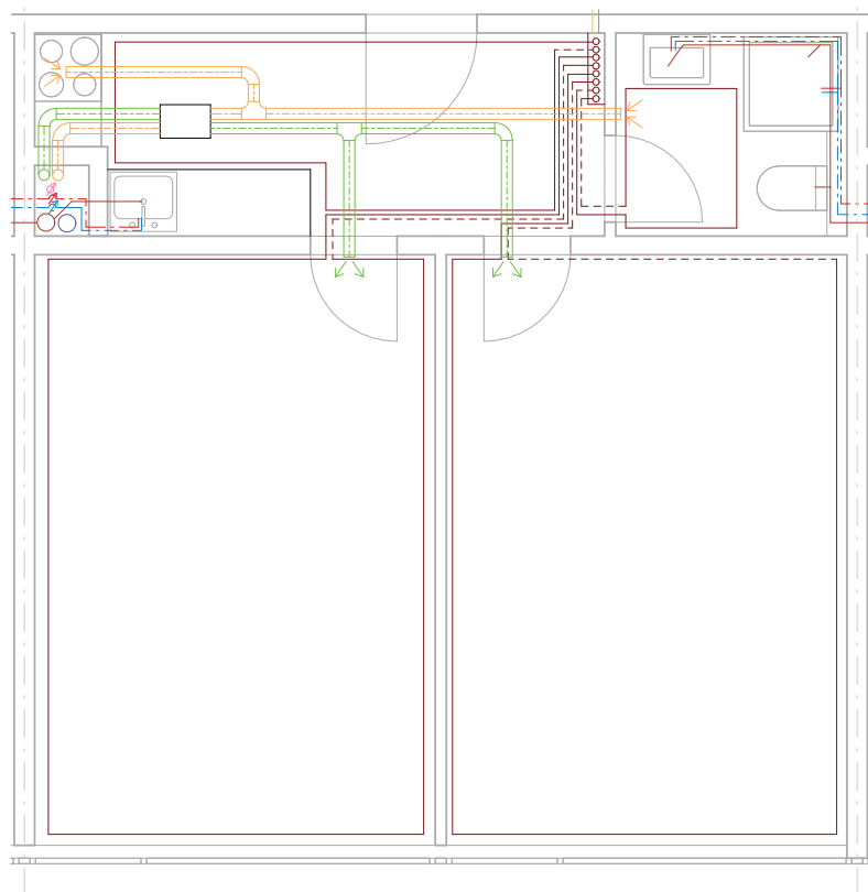
DETAIL OBYTNEJ BUNKY M 1:50
