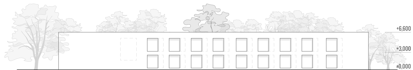
POHLED ZÁPADNÍ
