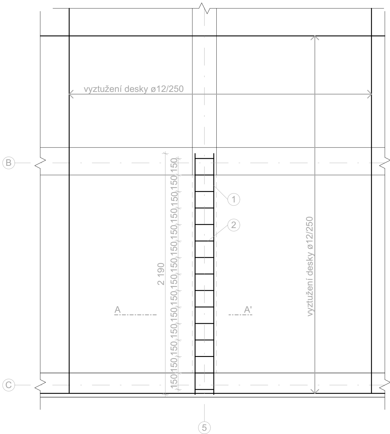
půdorys
